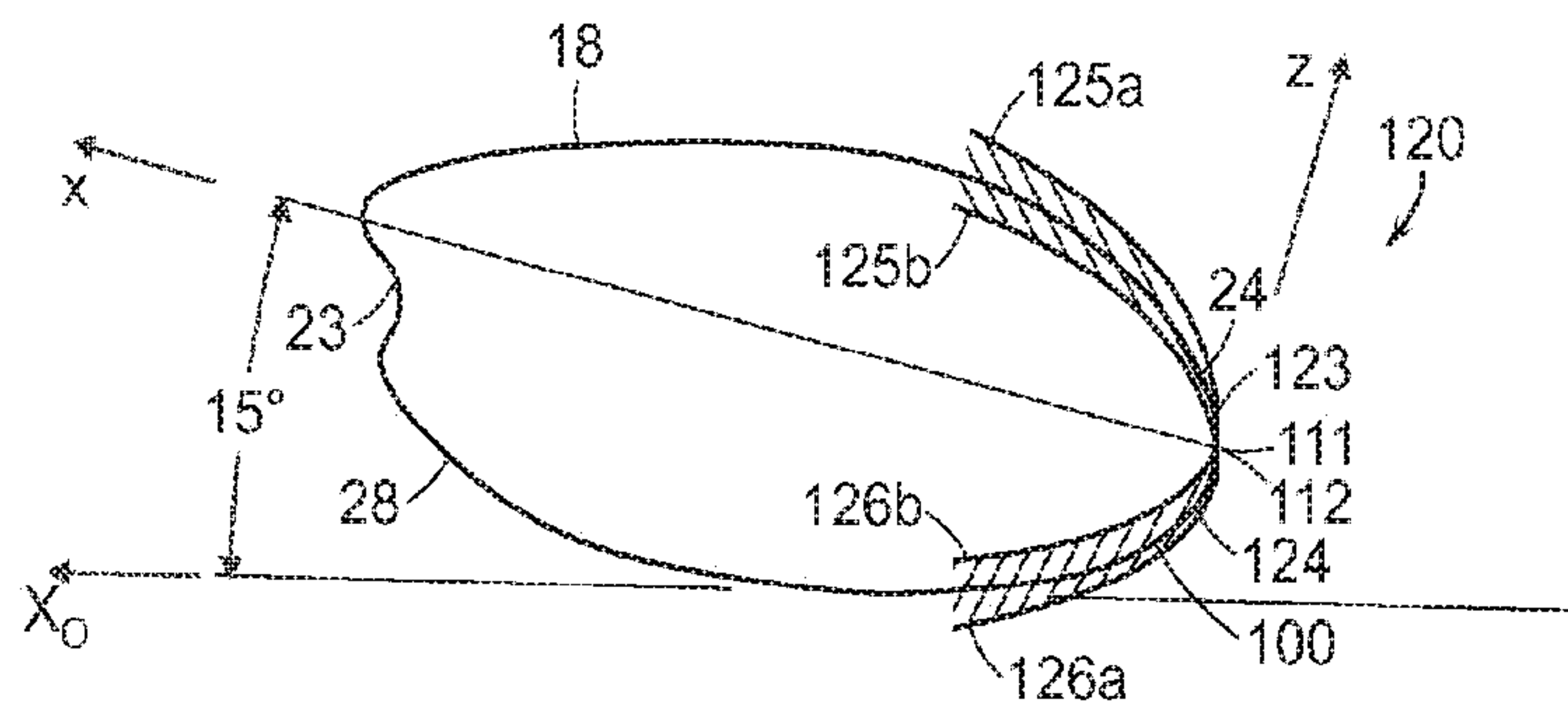
FIG. 30B
