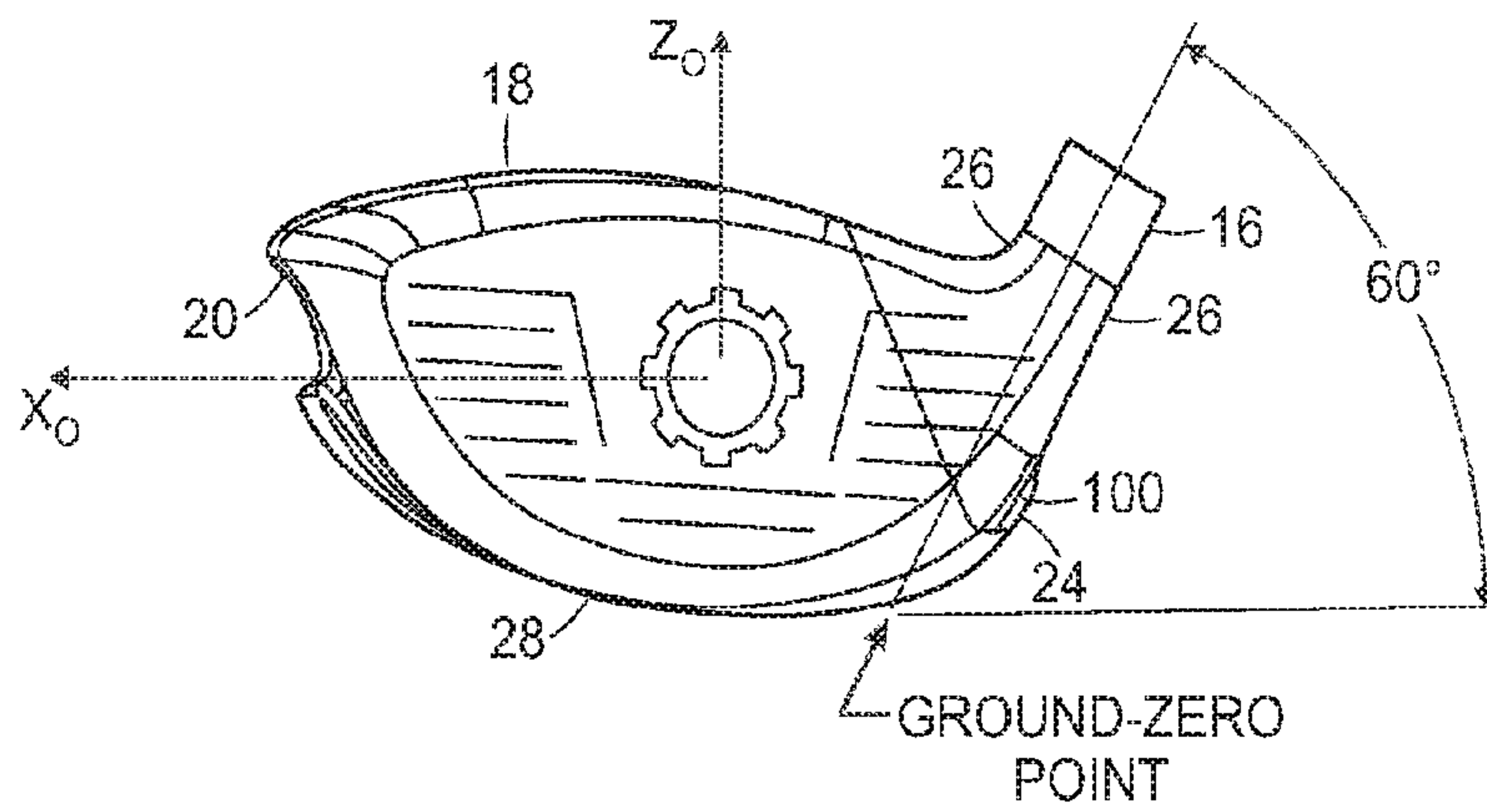
FIG. 28
