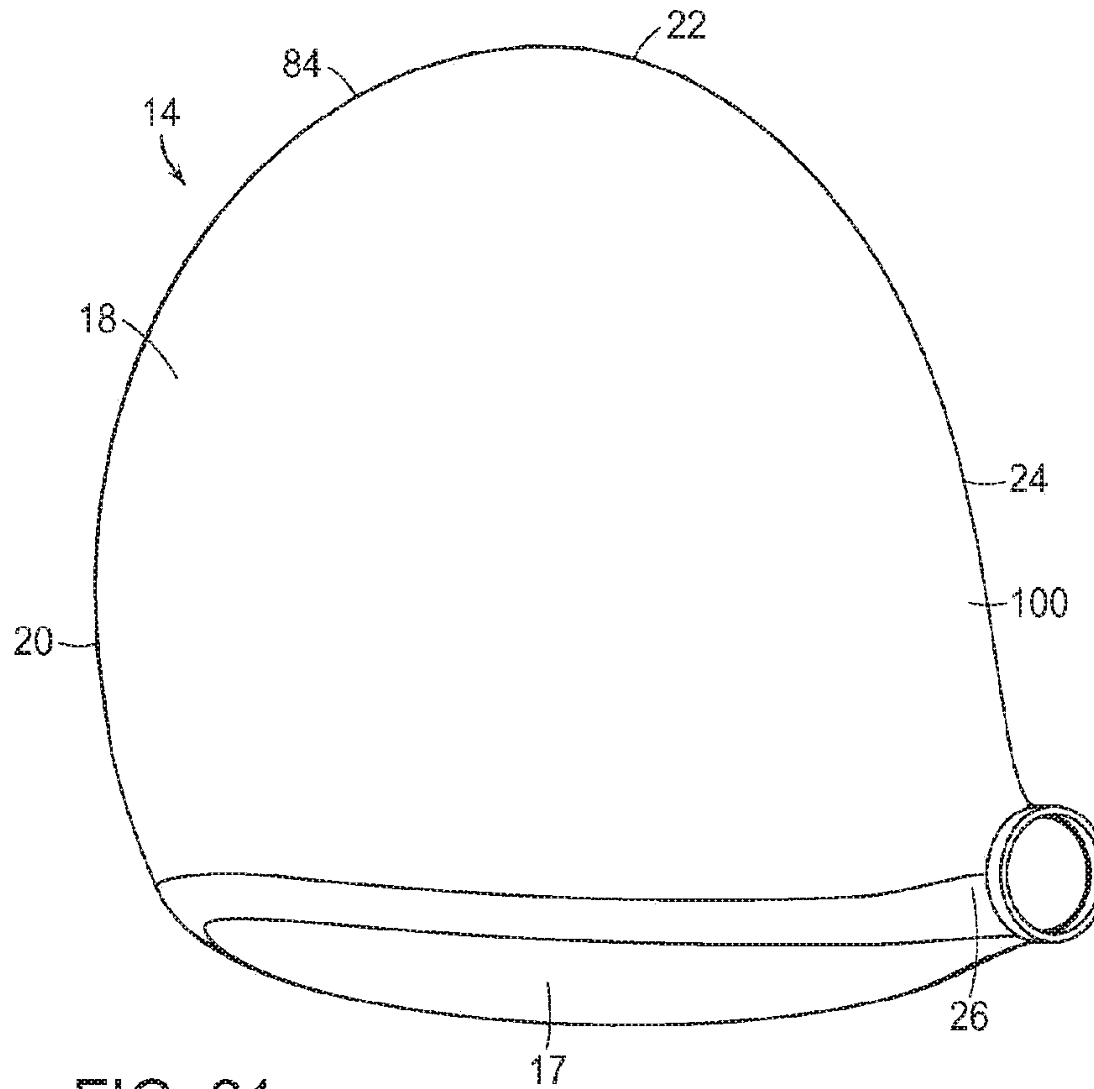
FIG. 21
