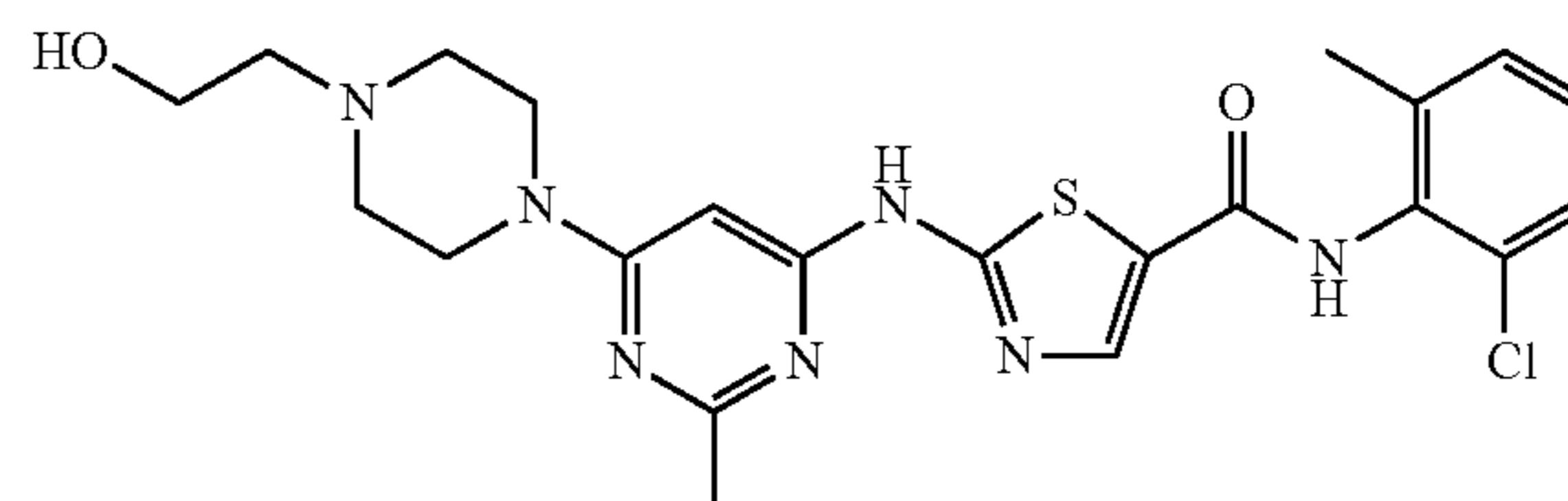
Dasatinib
