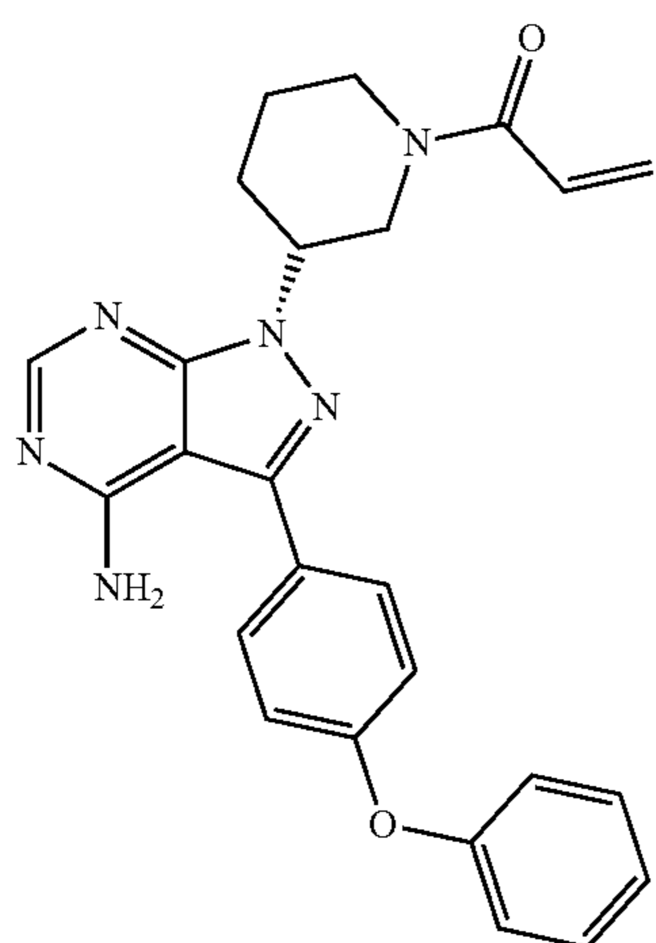
Ibrutinib
