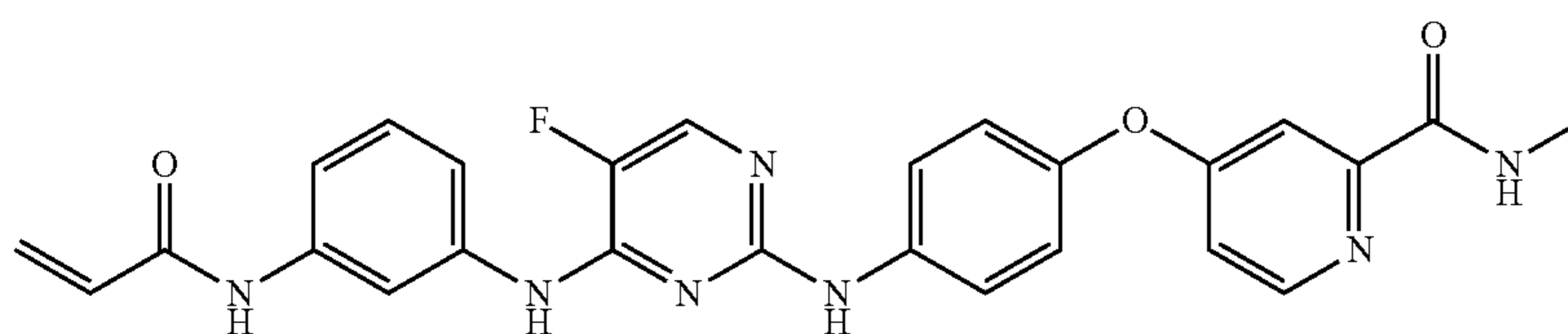
CNX-774
