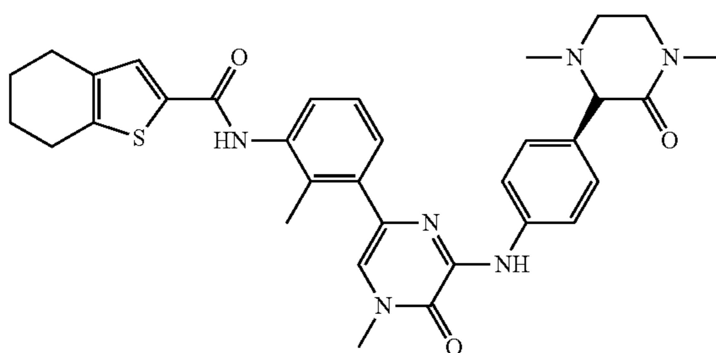
GDC-0834
