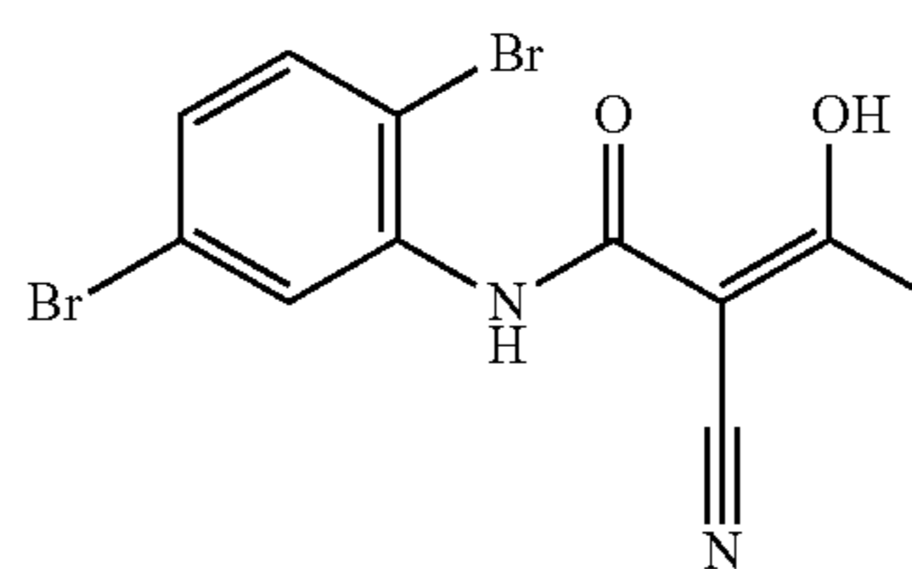
LFM-A13
