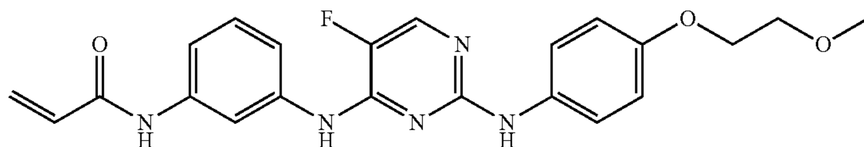
CC-292
