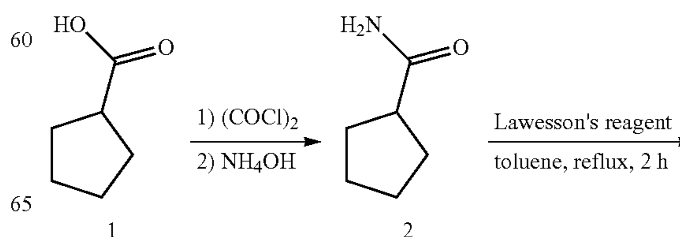
Scheme A-2
