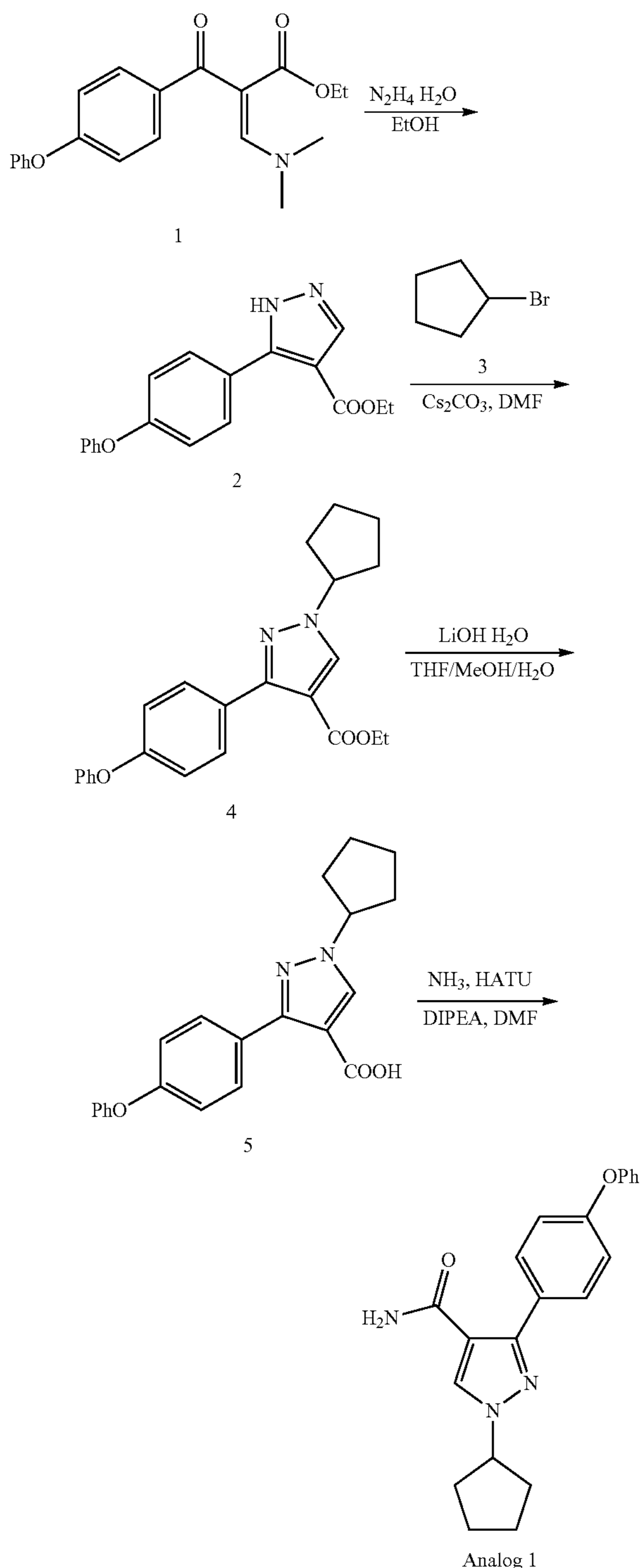
Scheme A-1
