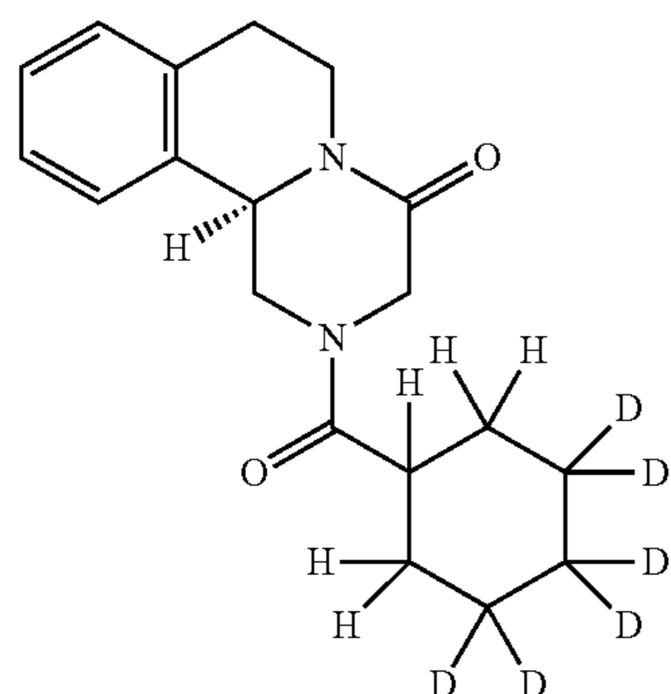
(R)-2-(3,3,4,4,5,5-d 6 -Cyclohexanecarbonyl)-2,3,6,7-tetrahydro-1H-pyrazino[2,1-a]isoquinolin-4(11bH)-one (109a)
