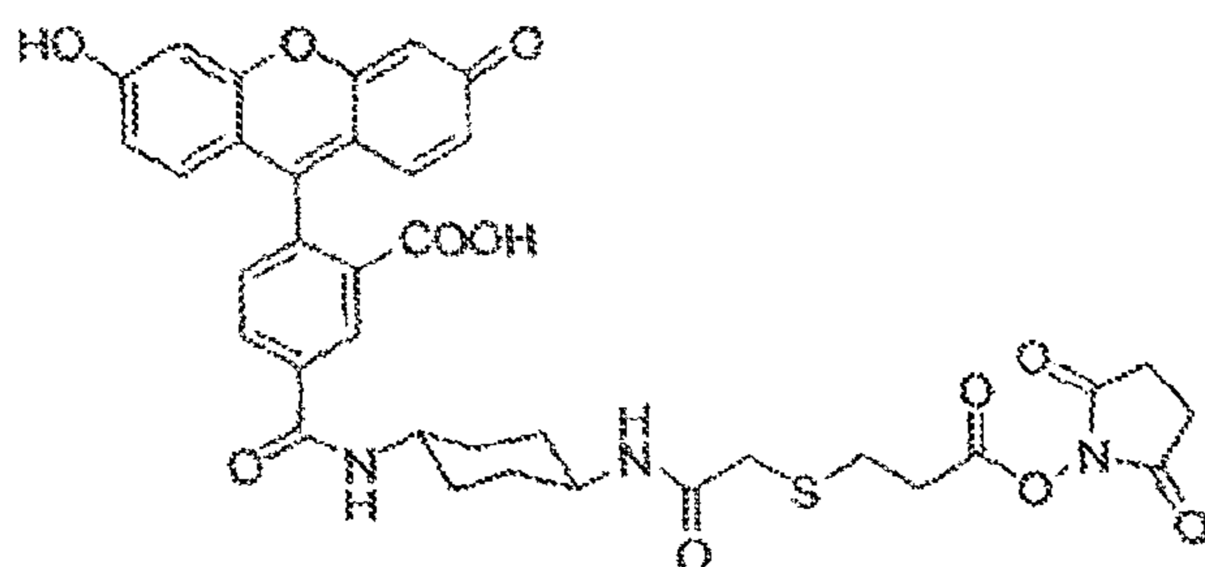
Pro18-NHS
