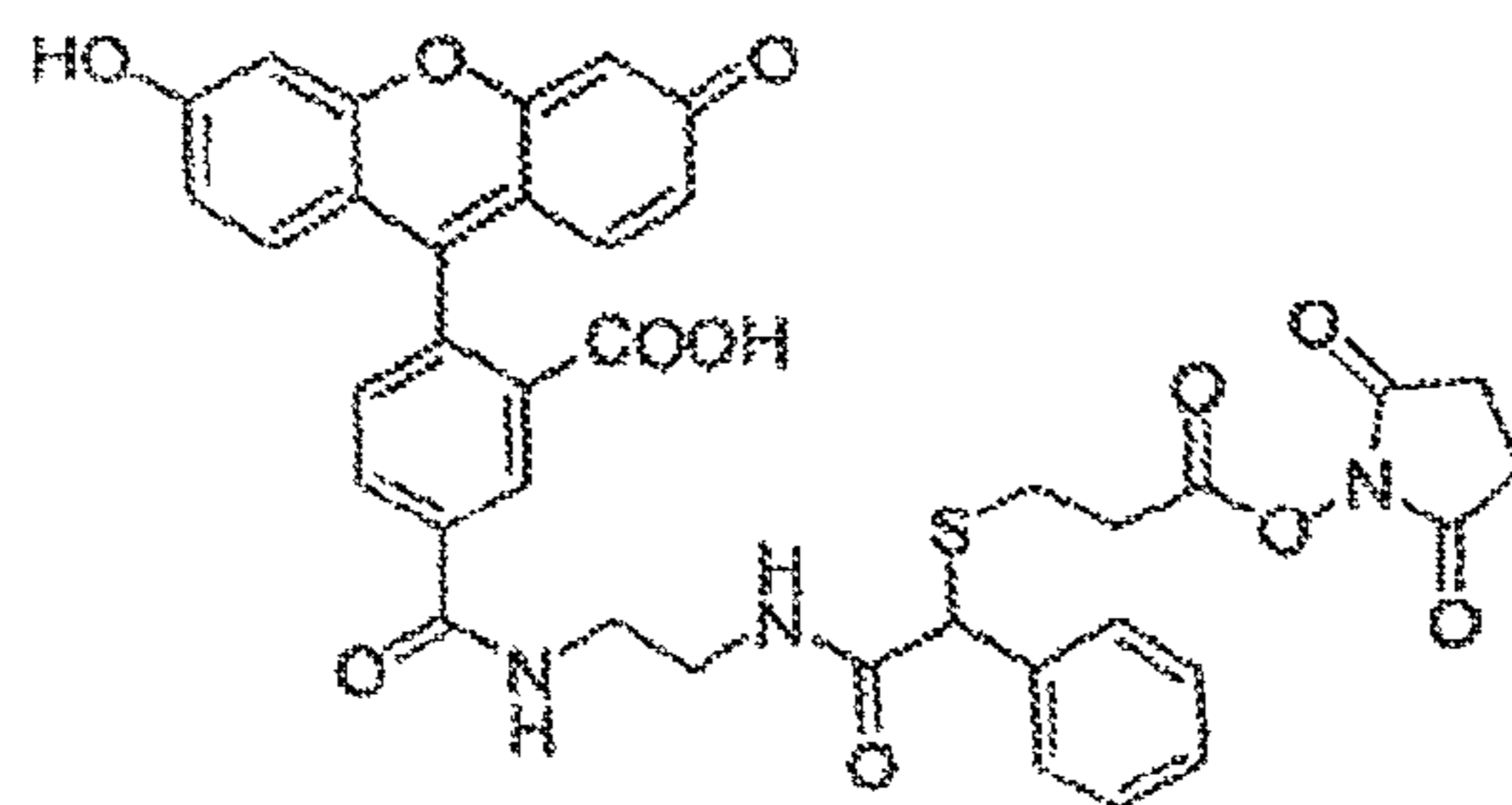
Pro32-NHS
