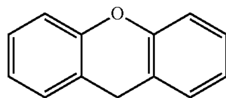
Xanthene
