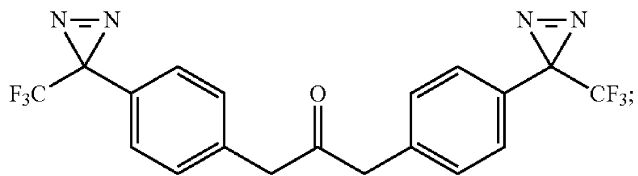
1,3-bis(4-(3-(trifluoromethyl)-3H-diazirin-3-yl)phenyl)propan-2-one
