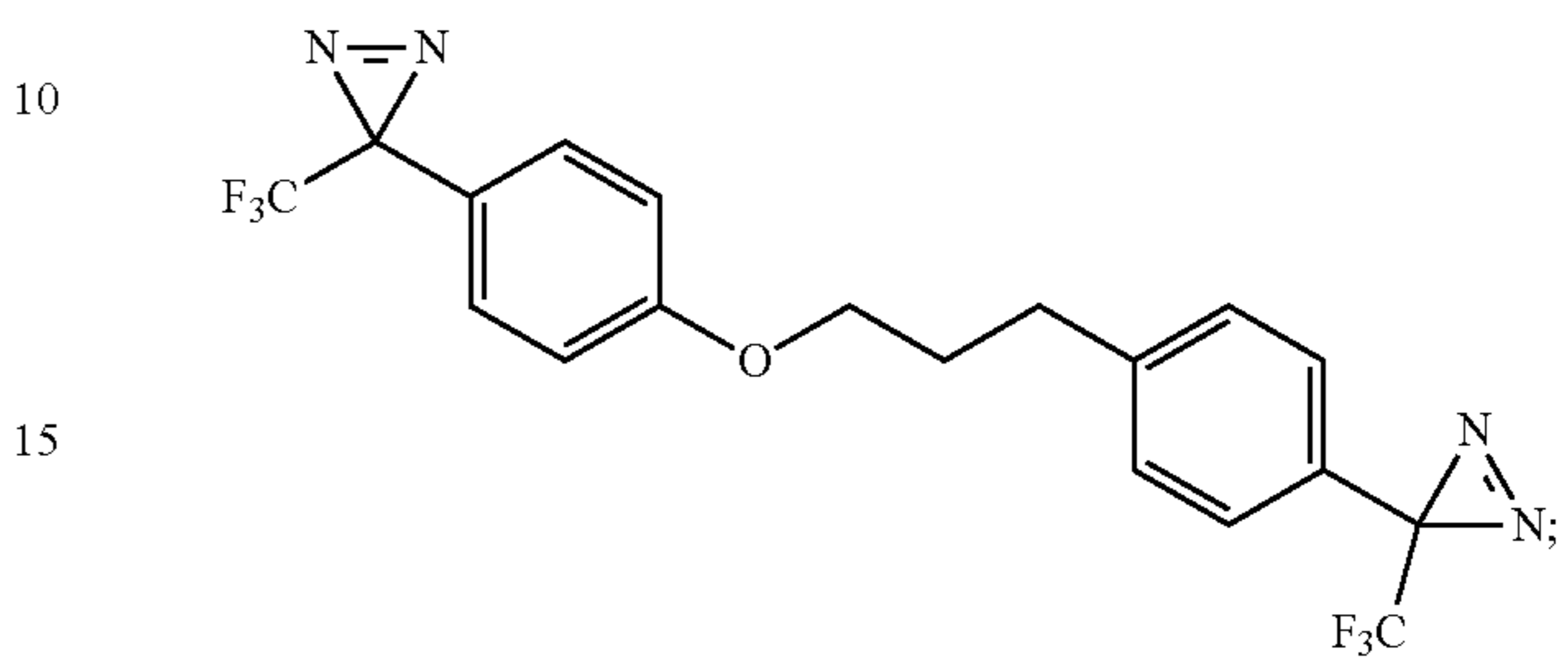
3-(trifluoromethyl)-3-(4-(3-(4-(3-(trifluoromethyl)-3H-diazirin-3-yl)phenoxy)propyl)phenyl)-3H-diazirine
