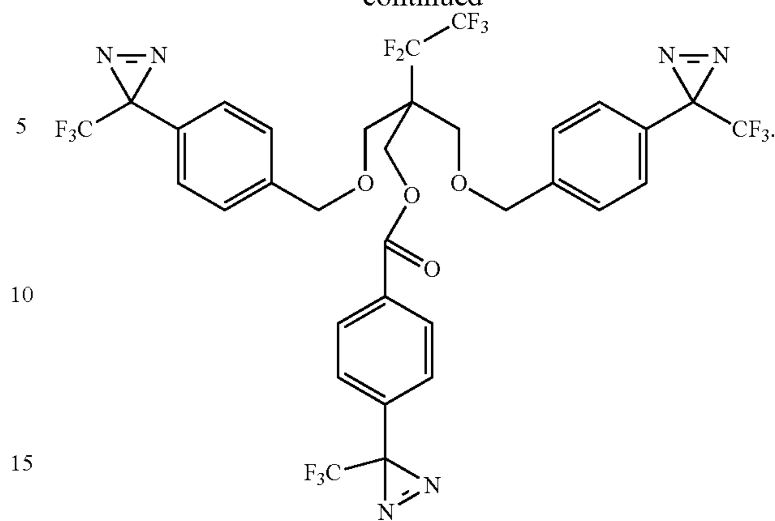
3,3'-(((2-(perfluoroethyl)-2-(((4-(3-(trifluoromethyl)-3H-diazirin-3-yl)benzyl)oxy)methyl)propane-1,3-diyl)bis(oxy))bis(methylene))bis(4,1-phenylene))bis(3-(trifluoromethyl)-3H-diazirine)
