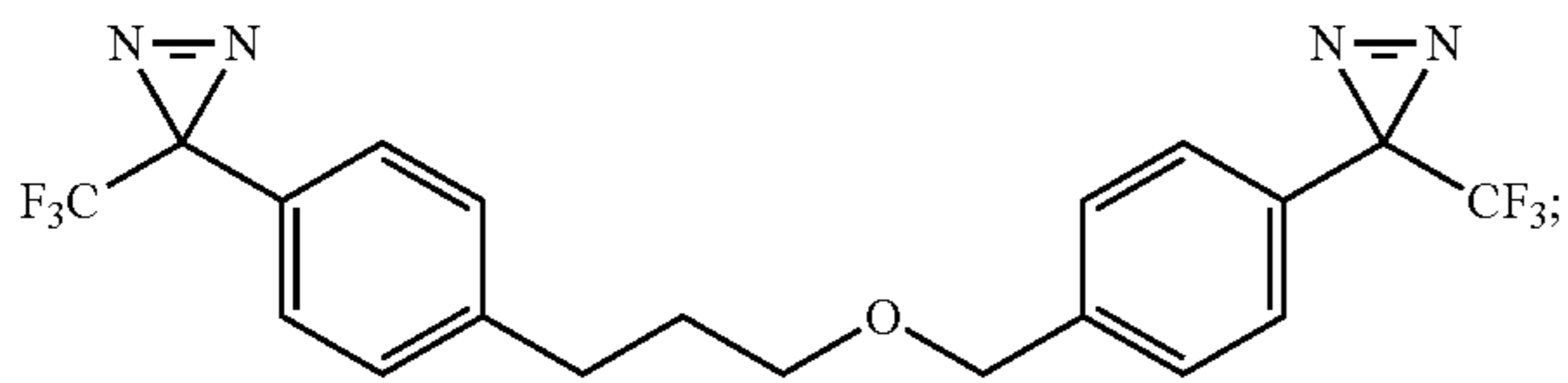
3-(trifluoromethyl)-3-(4-(3-((4-(3-(trifluoromethyl)-3H-diazirin-3-yl)benzyl)oxy)propyl)phenyl)-3H-diazirine
