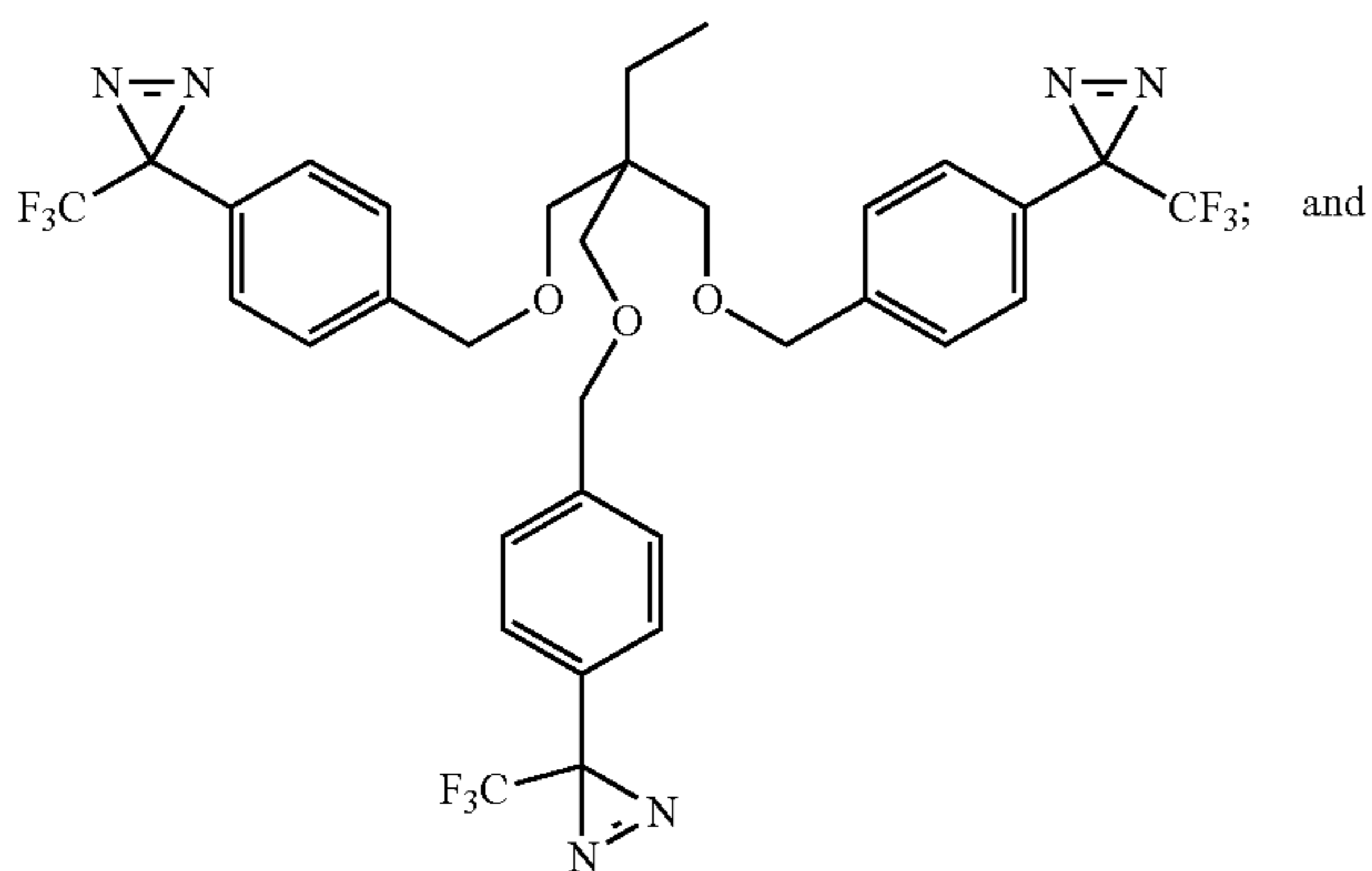
3,3'-(((2-ethyl-2-(((4-(3-(trifluoromethyl)-3H-diazirin-3-yl)benzyl)oxy)methyl)propane-1,3-diyl)bis(oxy))bis(methylene))bis(4,1-phenylene))bis(3-(trifluoromethyl)-3H-diazirine)
