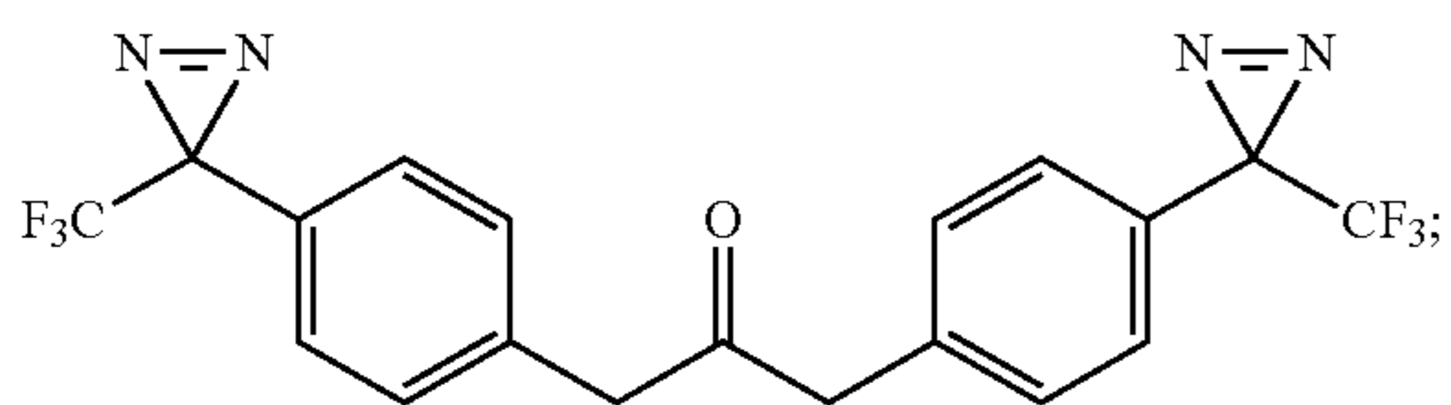
1,3-bis(4-(3-(trifluoromethyl)-3H-diazirin-3-yl)phenyl)propan-2-one
