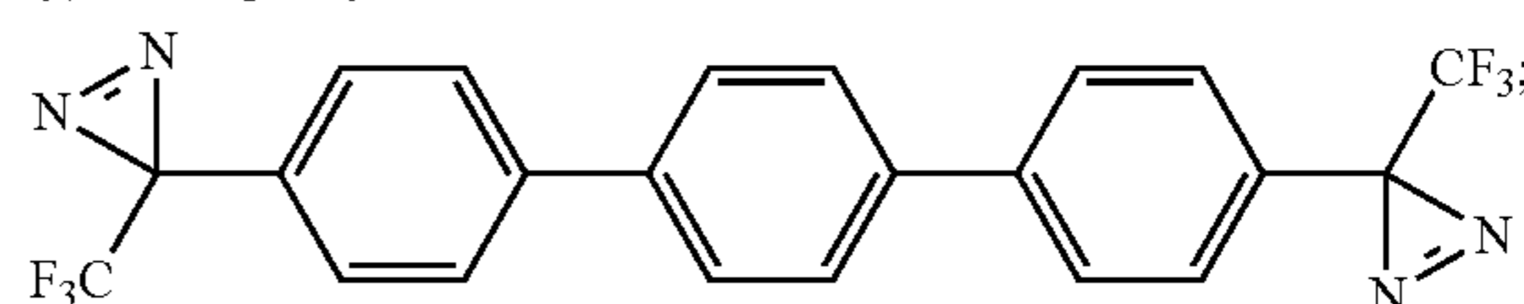
4,4''-bis(3-(trifluoromethyl)-3H-diazirin-3-yl)-1,1':4',1''-terphenyl
