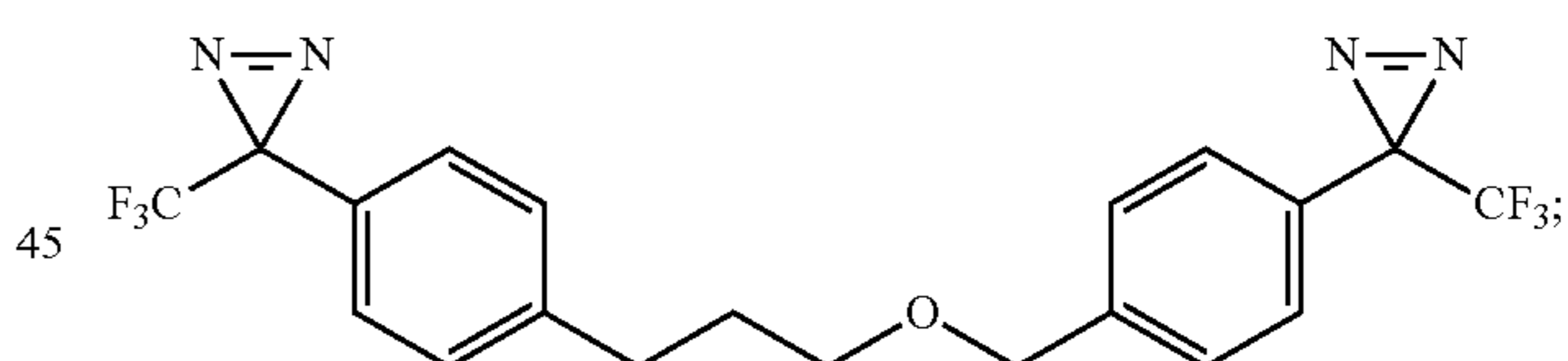
3-(trifluoromethyl)-3-(4-(3-((4-(3-(trifluoromethyl)-3H-diazirin-3-yl)benzyl)oxy)propyl)phenyl)-3H-diazirine
