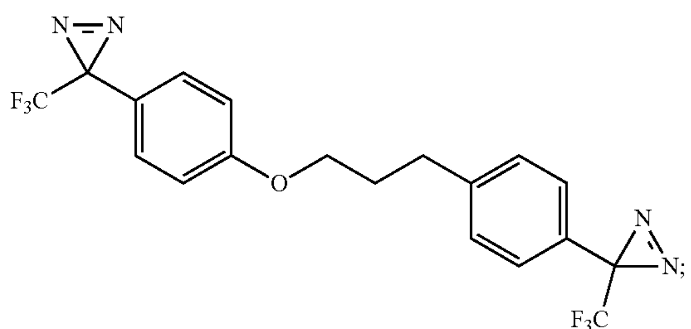
3-(trifluoromethyl)-3-(4-(3-(4-(3-(trifluoromethyl)-3H-diazirin-3-yl)phenoxy)propyl)phenyl)-3H-diazirine
