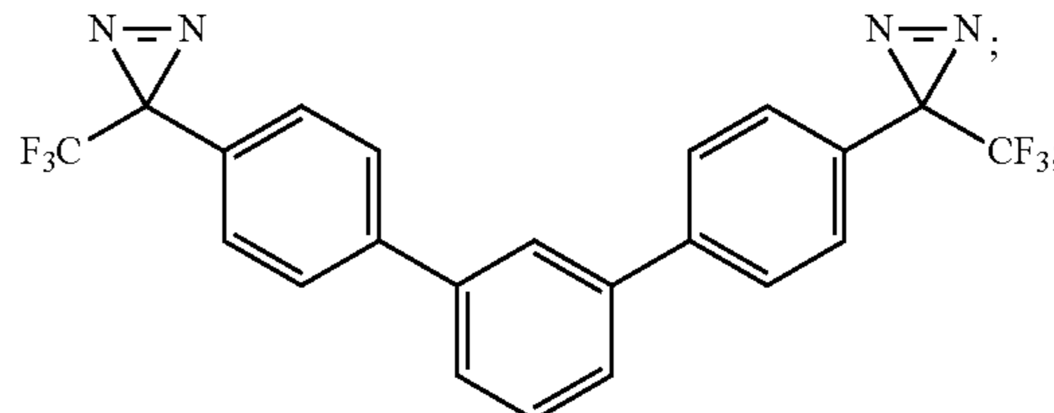
4,4''-bis(3-(trifluoromethyl)-3H-diazirin-3-yl)-1,1':3',1''-terphenyl
