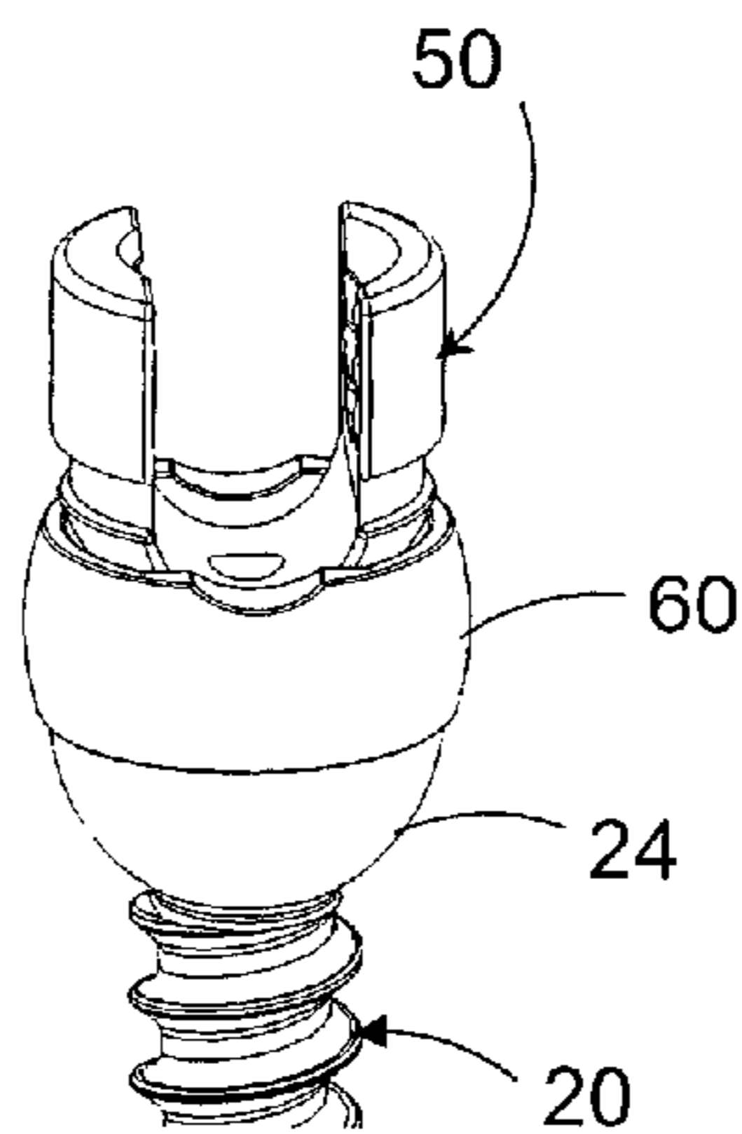
FIG. 8e
