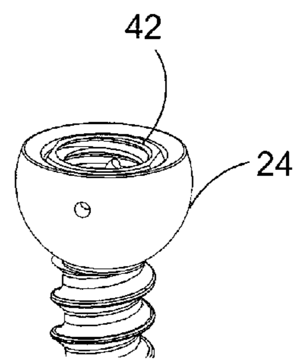
FIG. 8c
