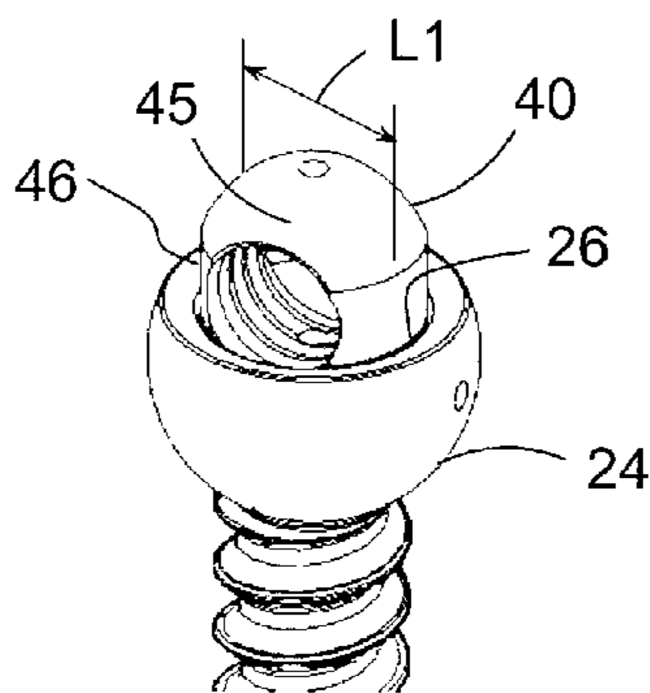
FIG. 8b
