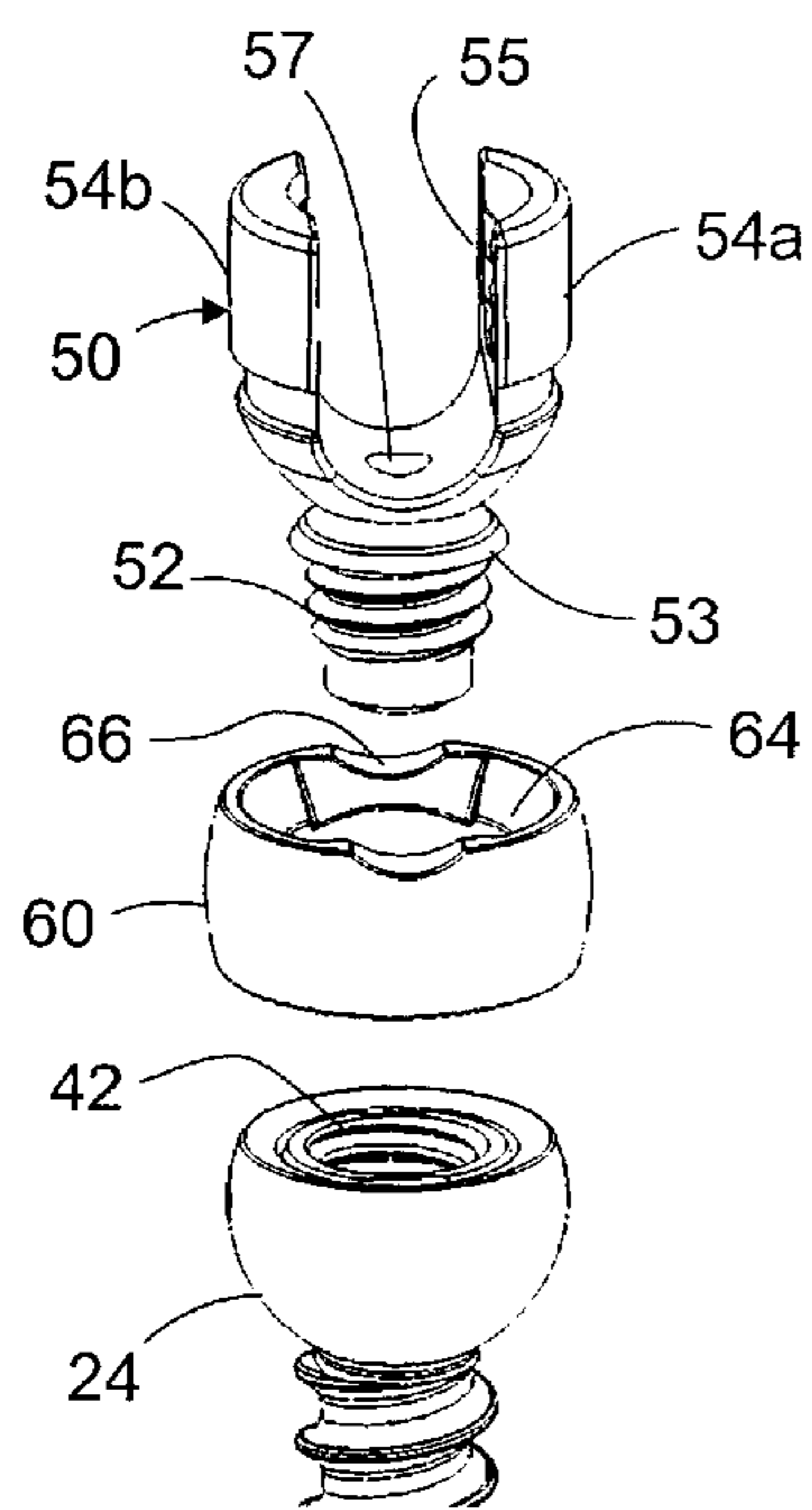
FIG. 8d
