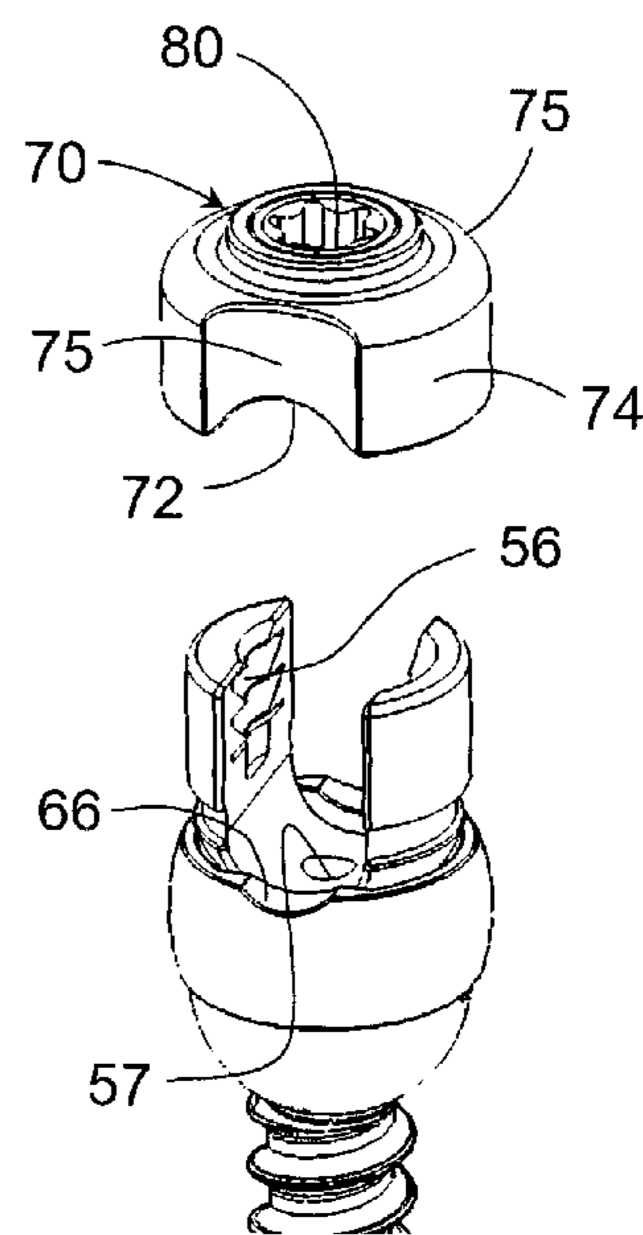
FIG. 8f
