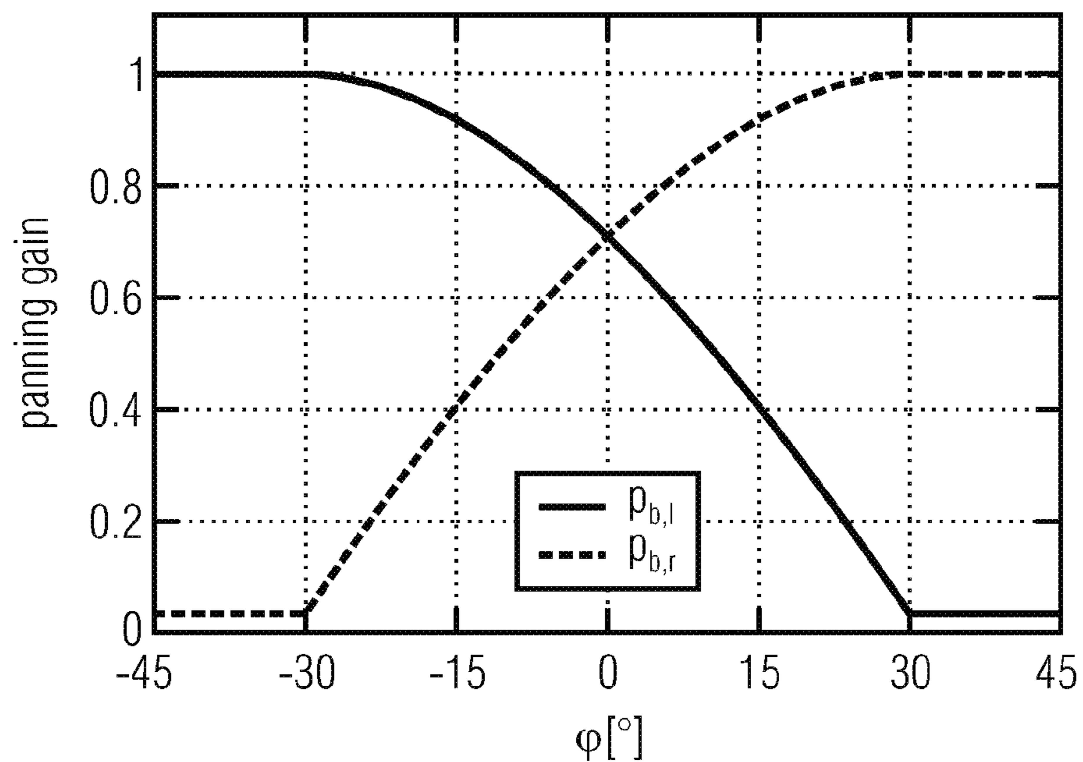
VBAF panning function
