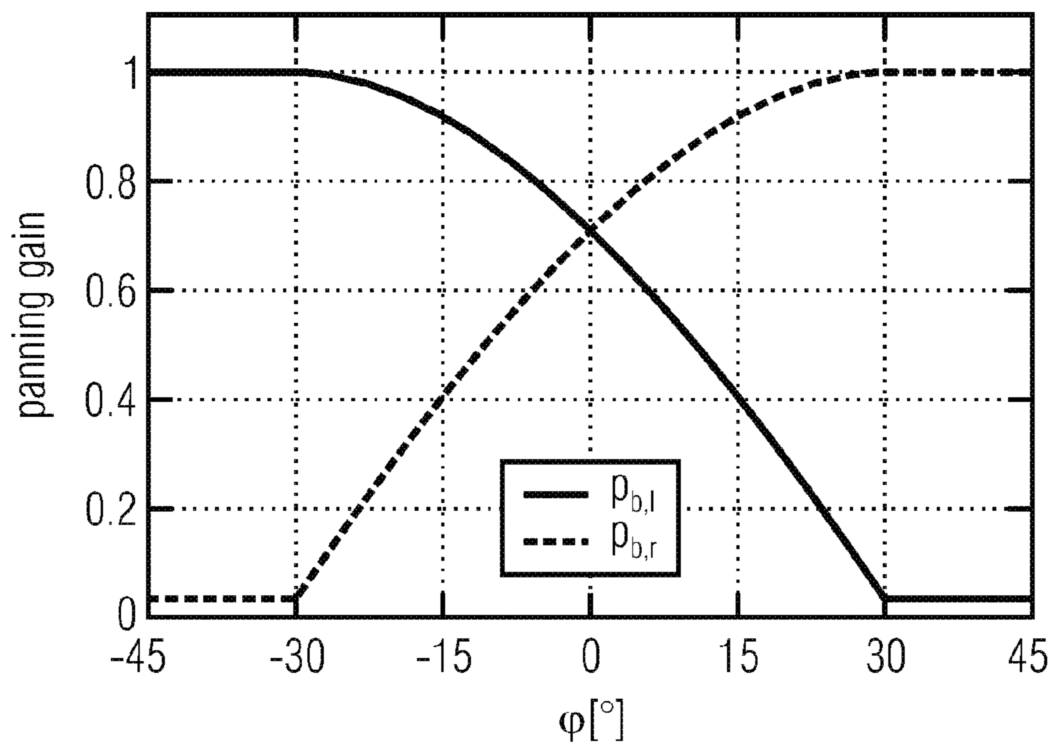
VBAF panning function
