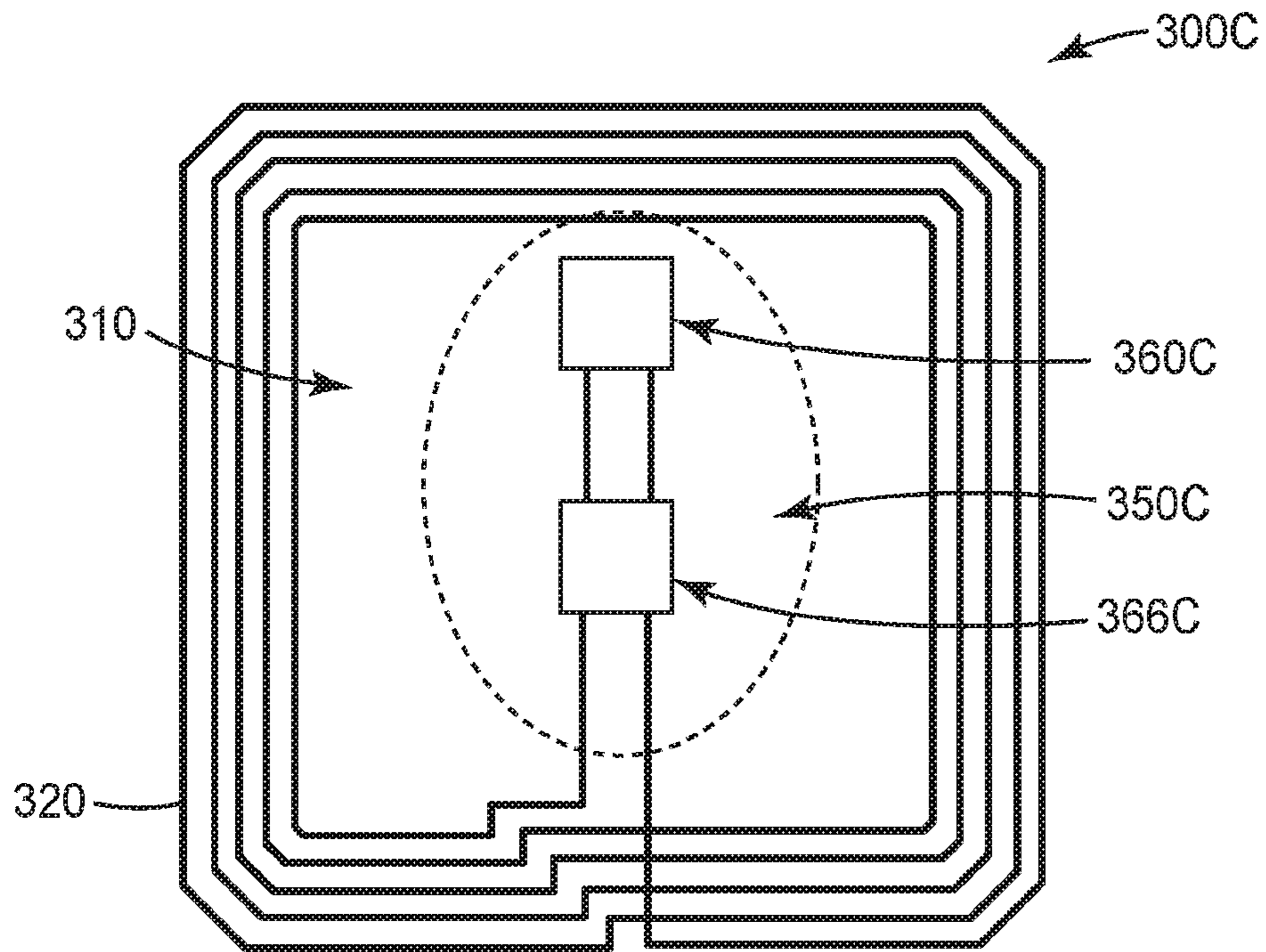
FIG. 3C
