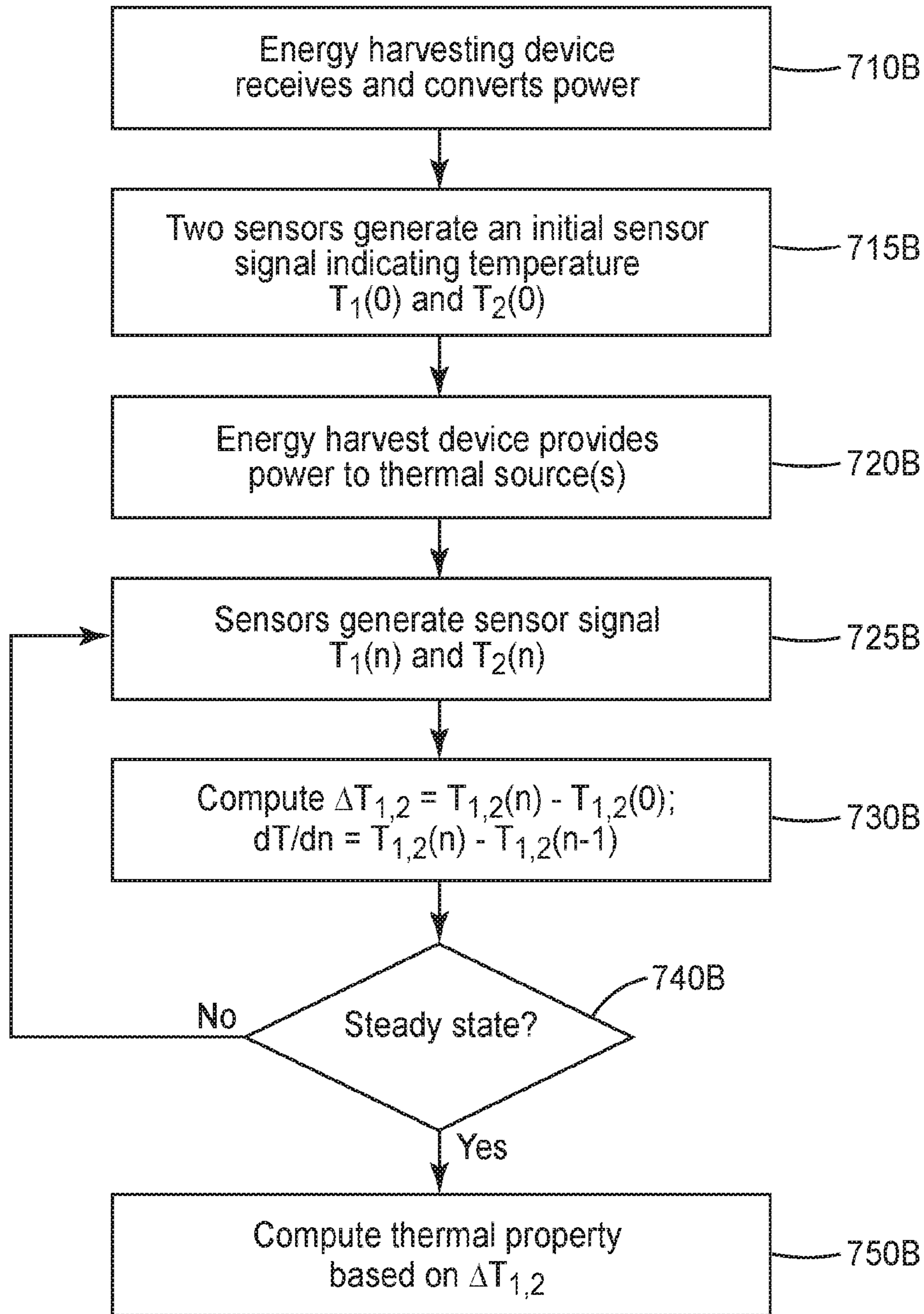
FIG. 7B
