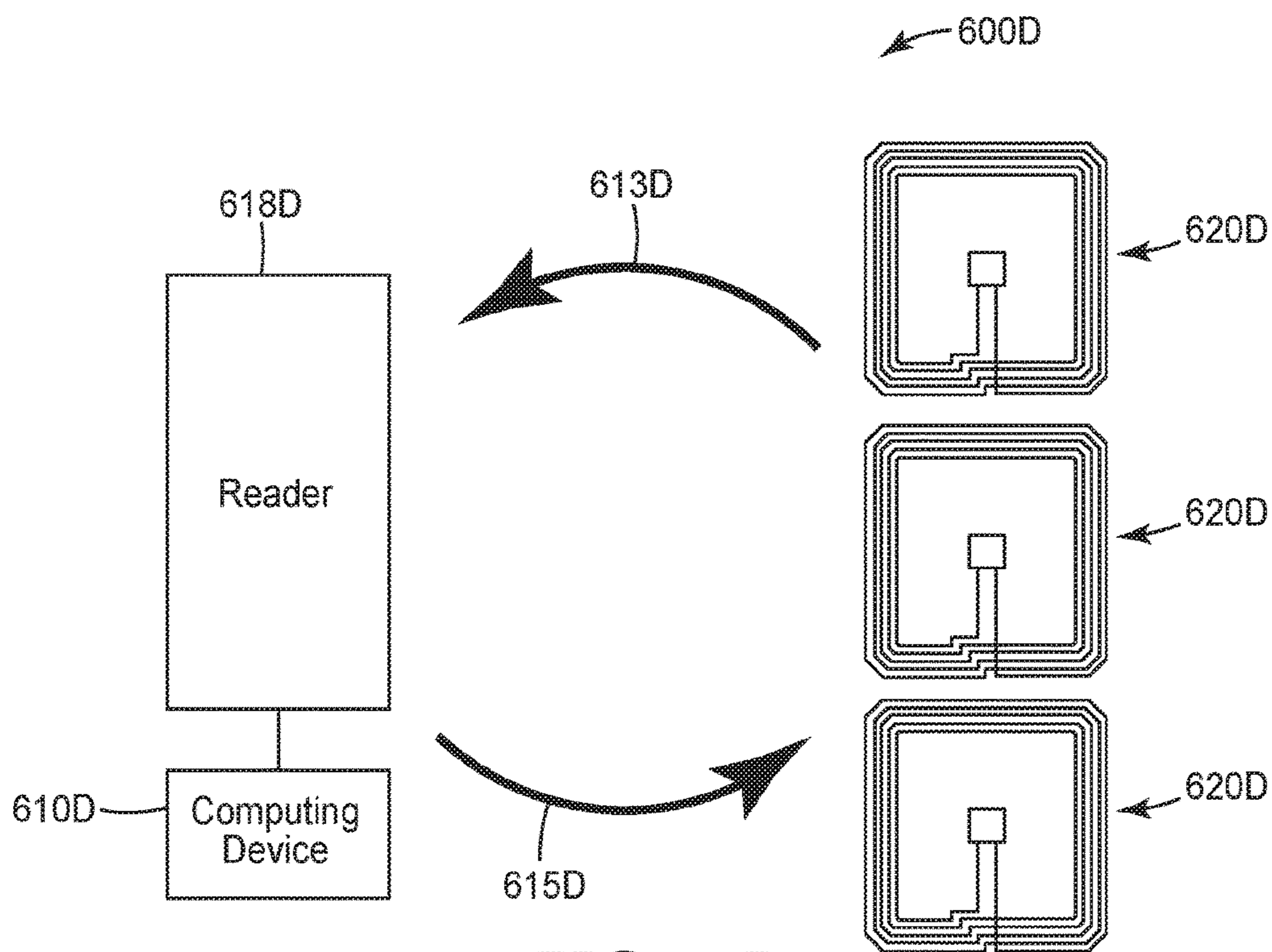
FIG. 6D
