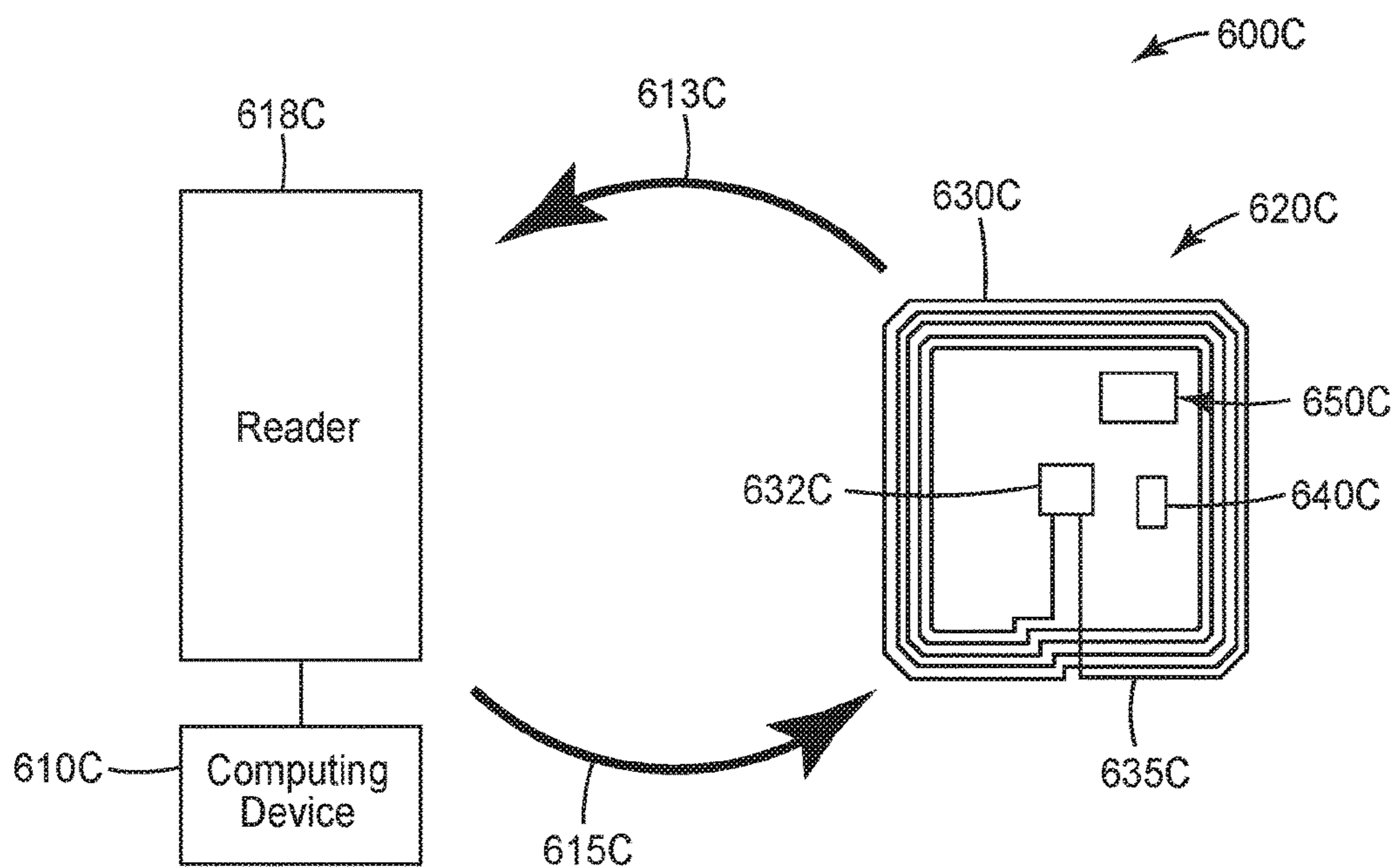
FIG. 6C
