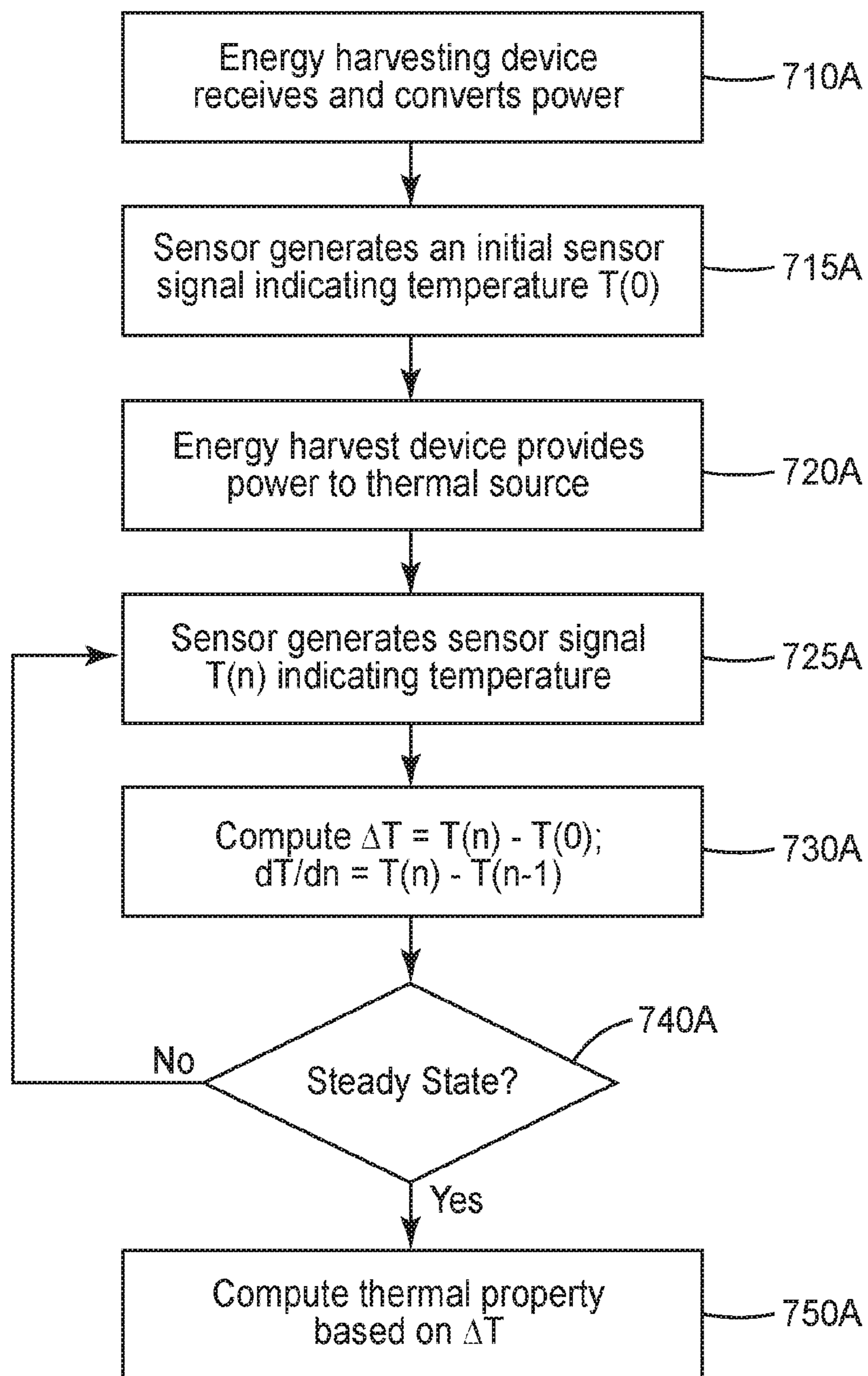
FIG. 7A
