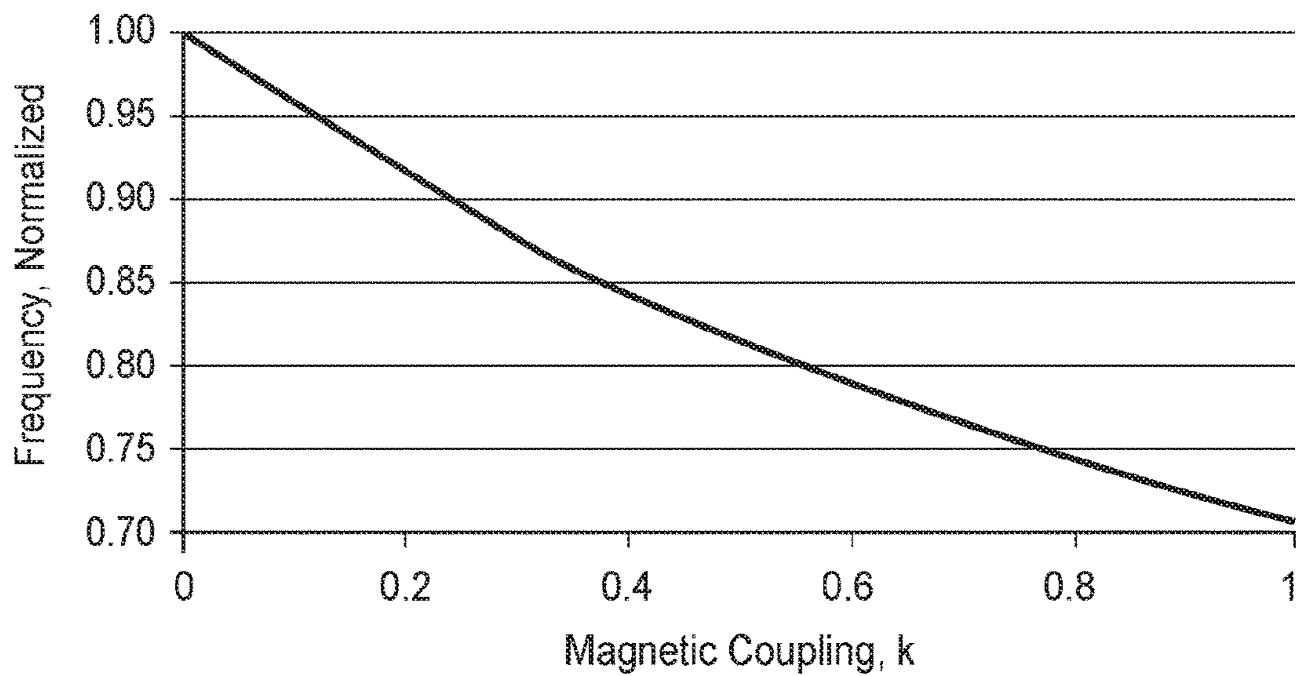
FIG. 8A
