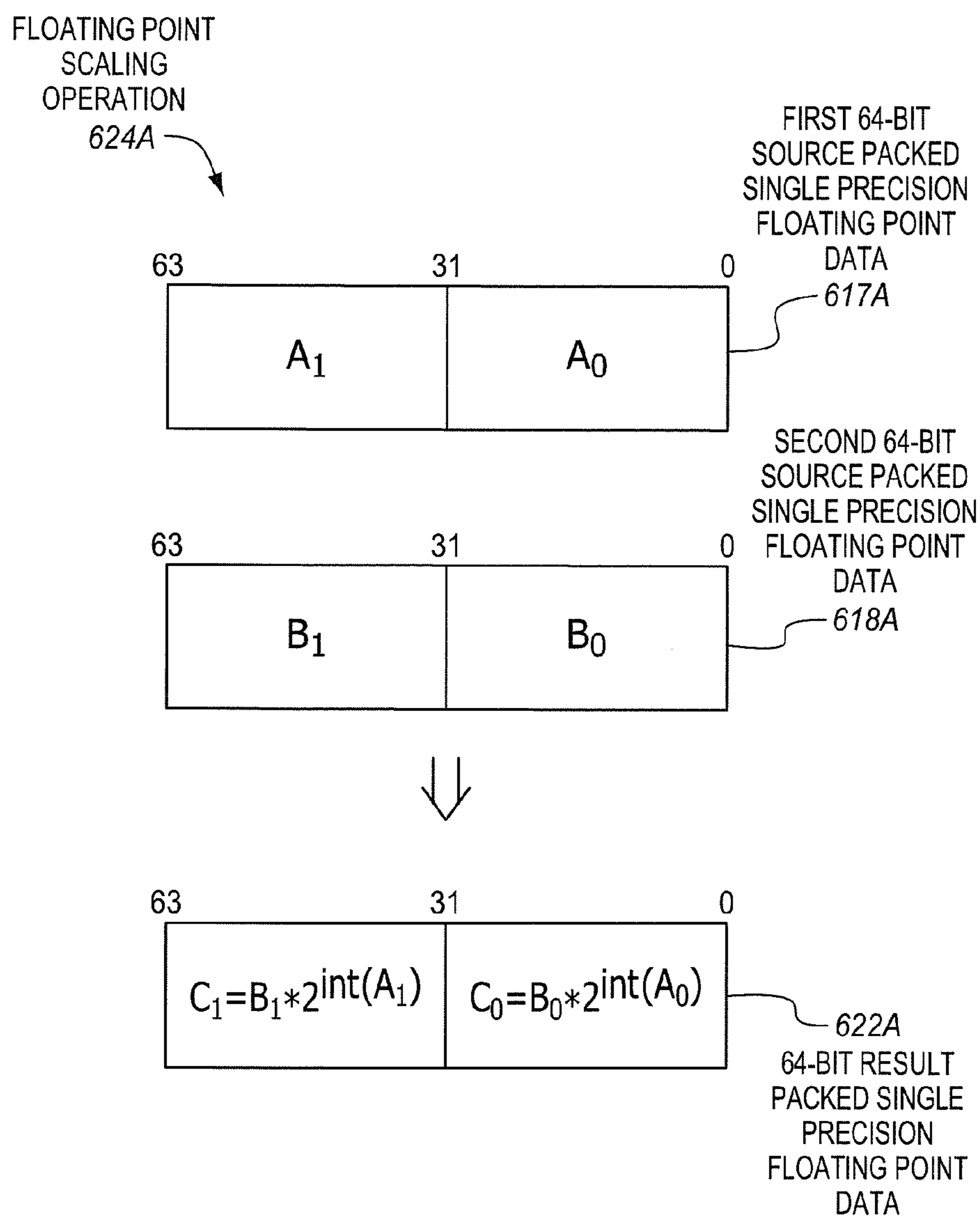
FIG. 6A
