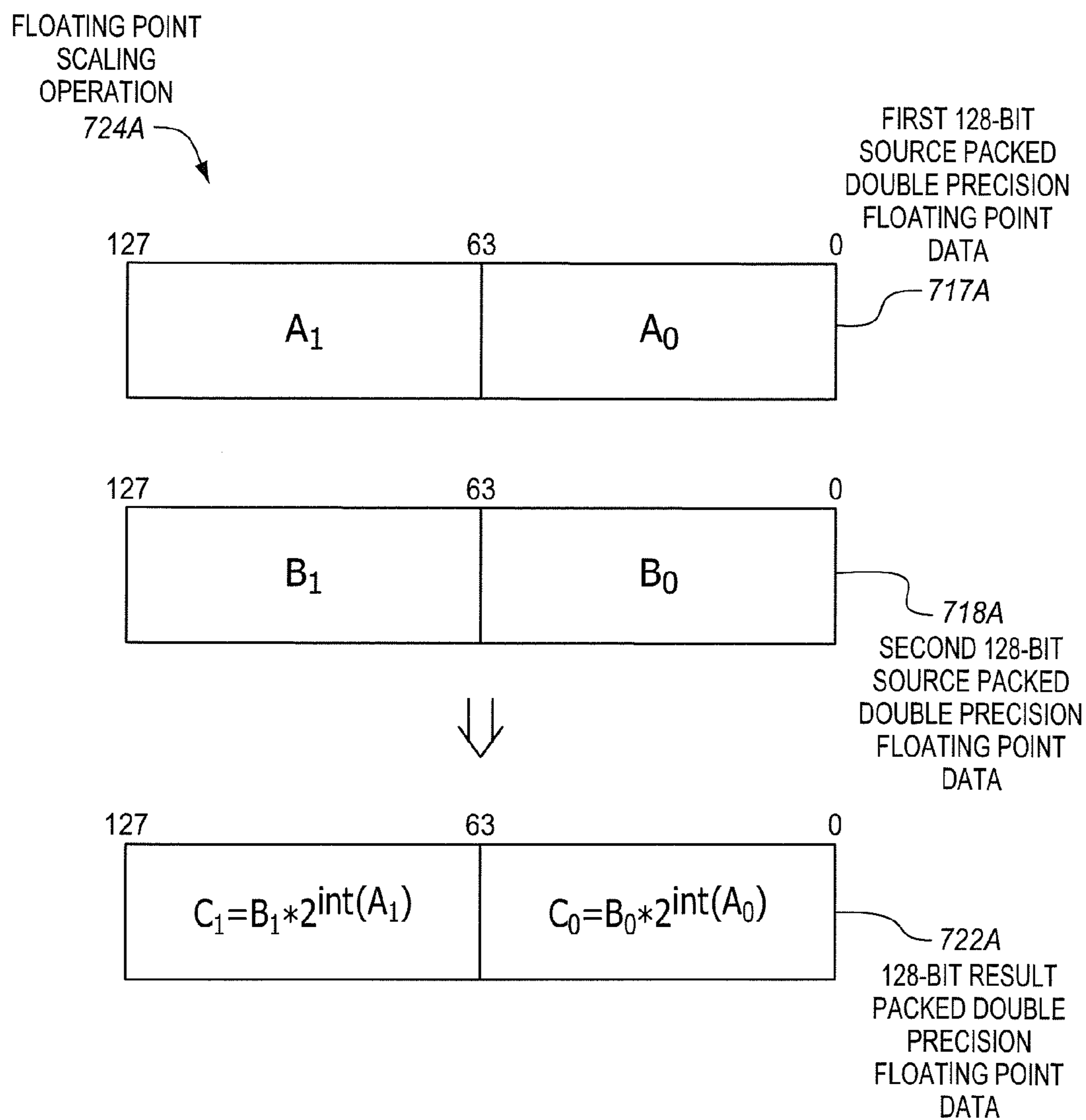
FIG. 7A
