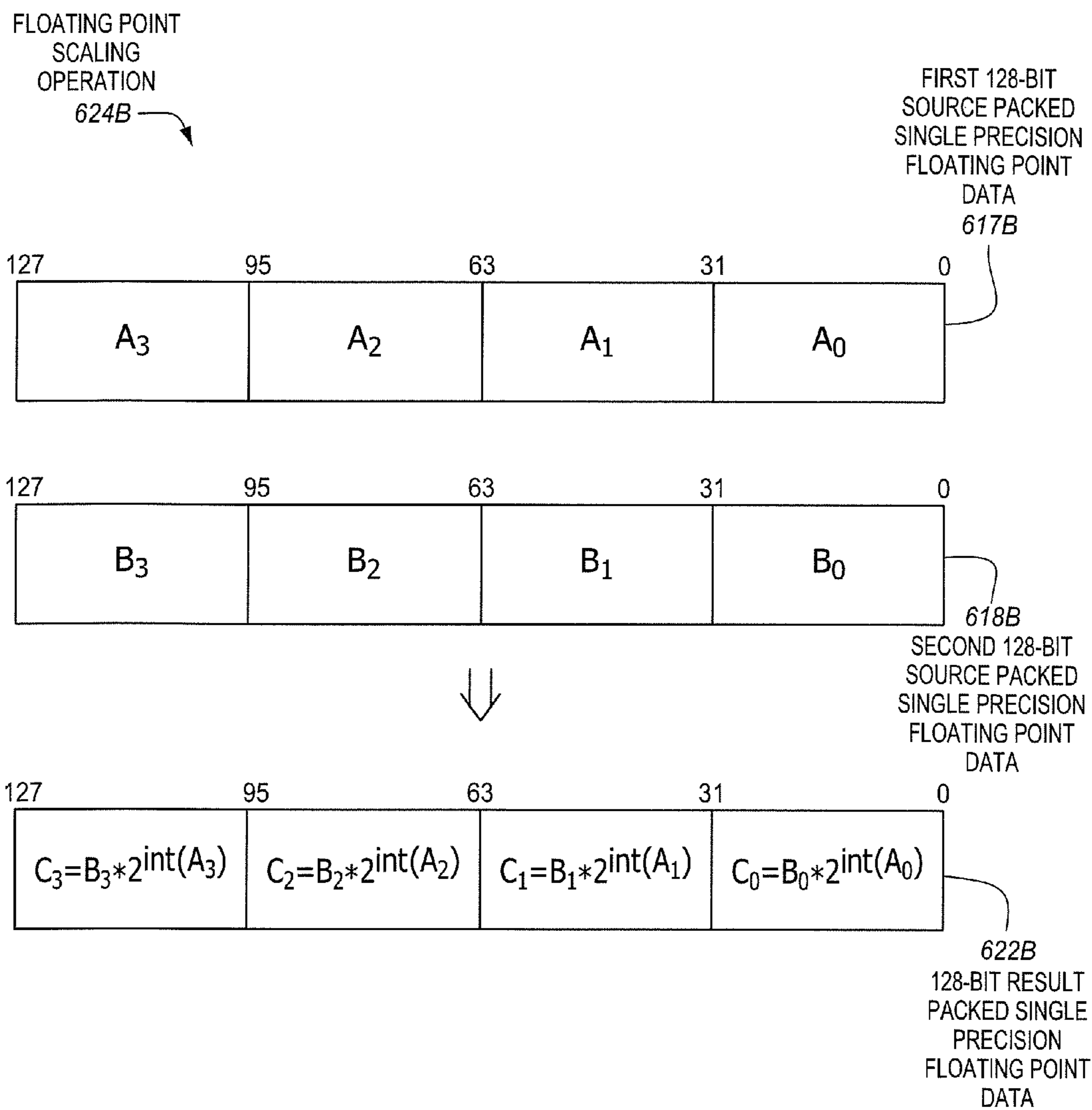
FIG. 6B
