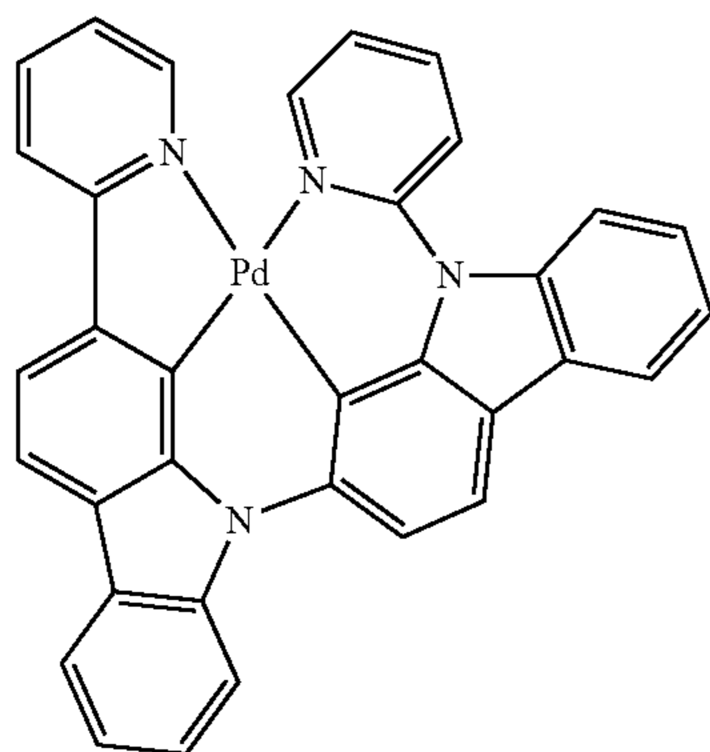
PdN3N
