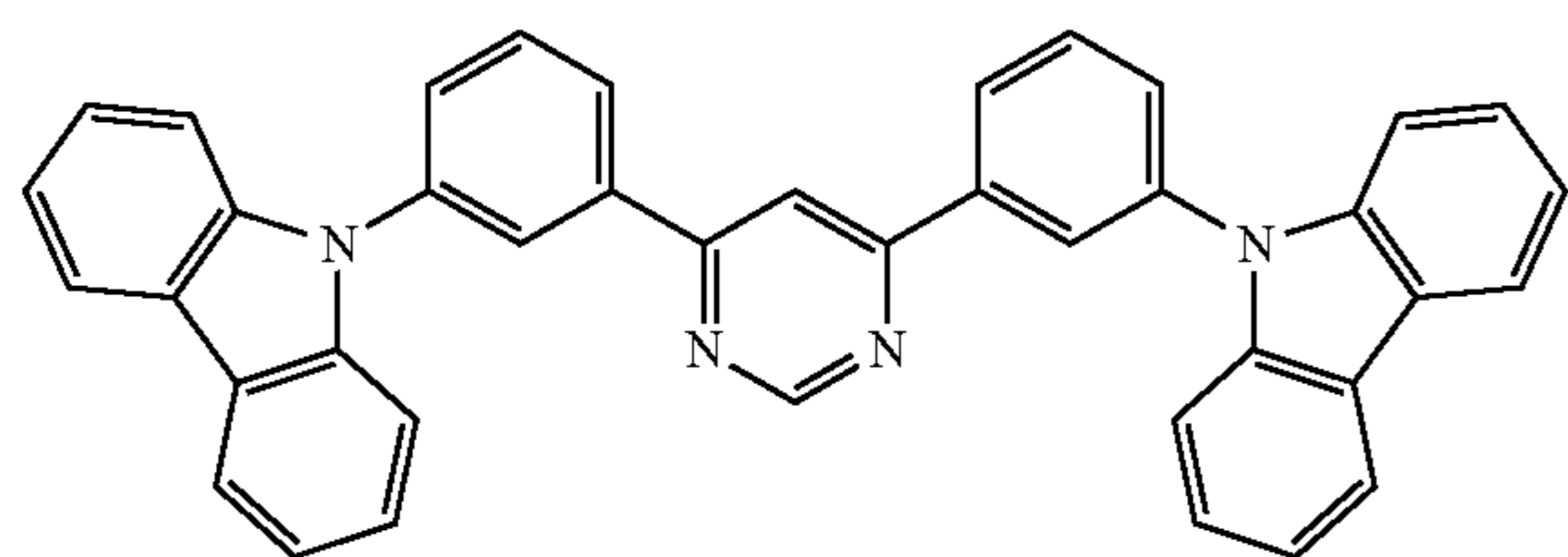
4,6mCzP2Pm
