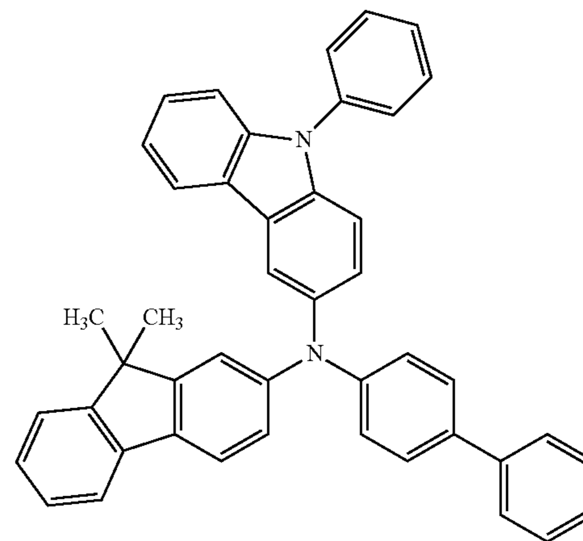
PCBIF
