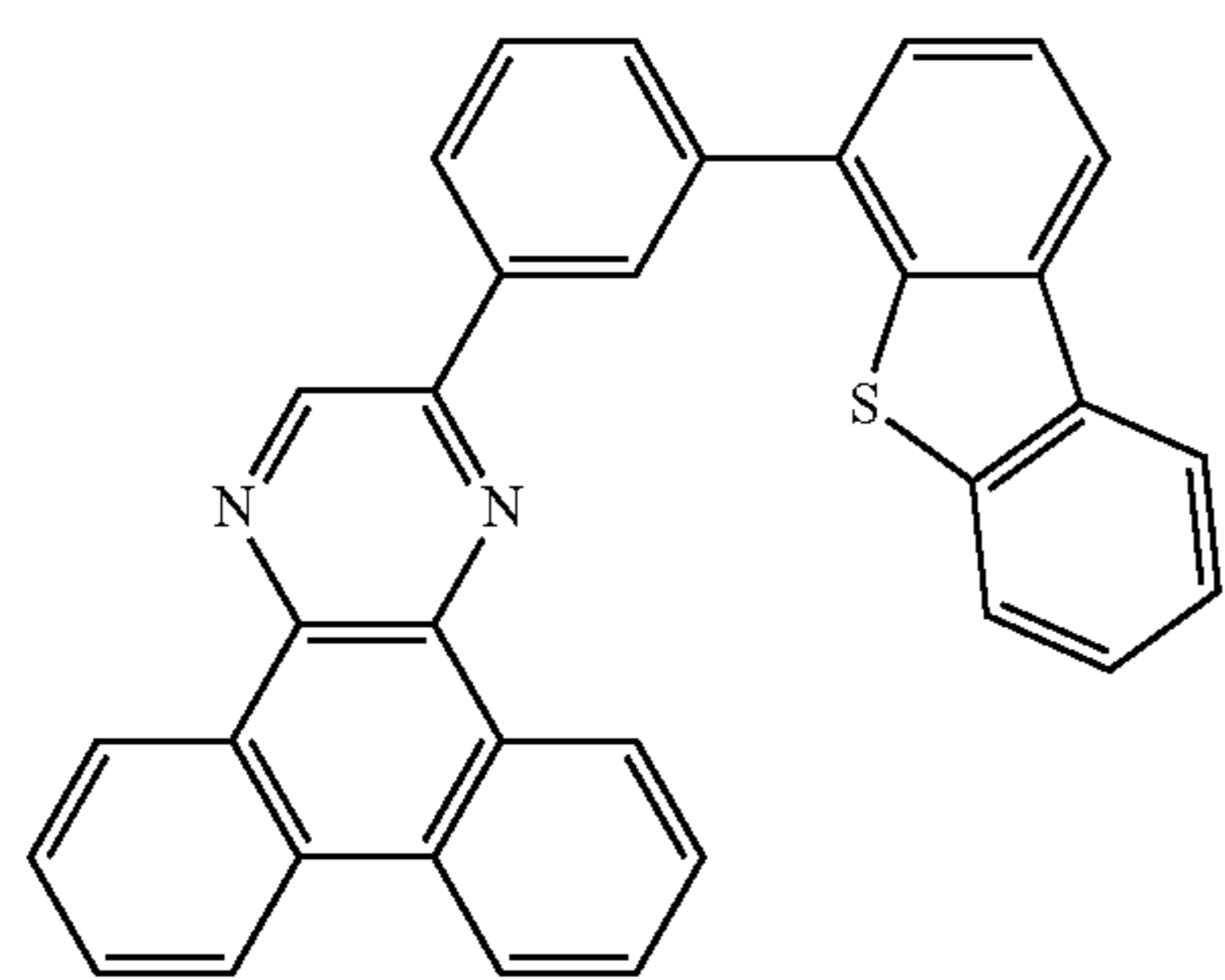
2mDBTPDBq-II
