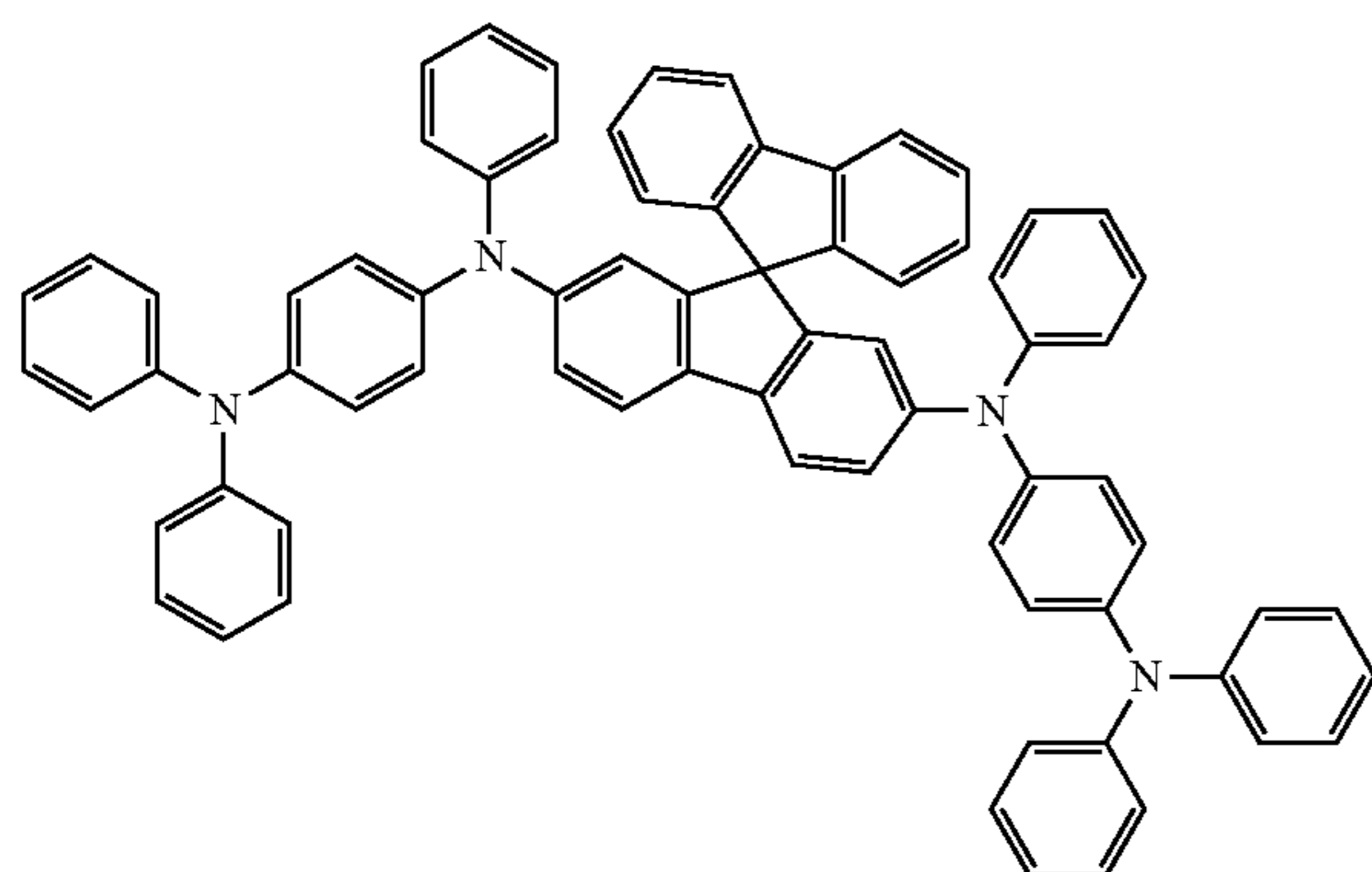
DPA2SF
