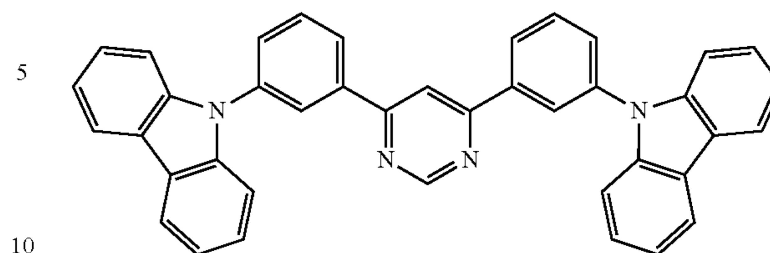
4,6mCzP2Pm
