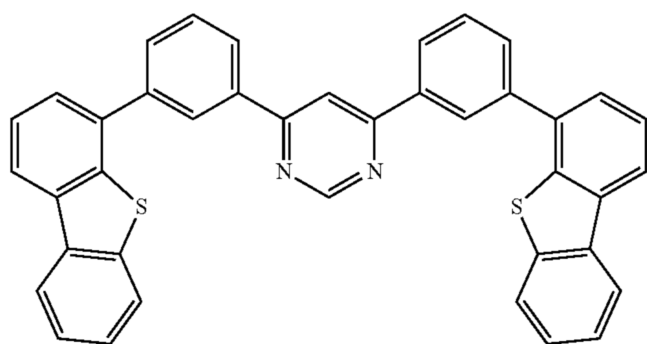
4,6mDBTP2Pm-II
