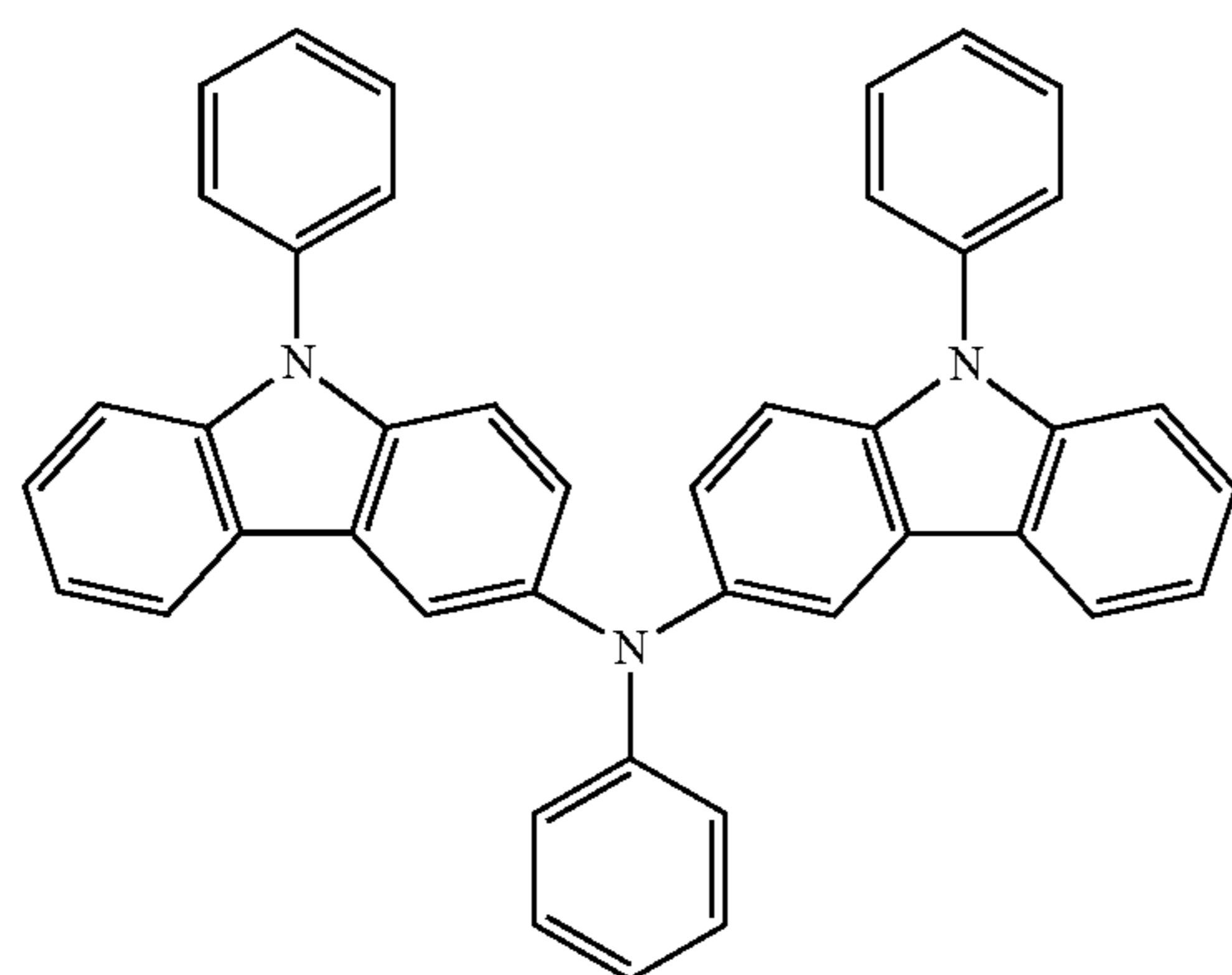
PCzPCA1
