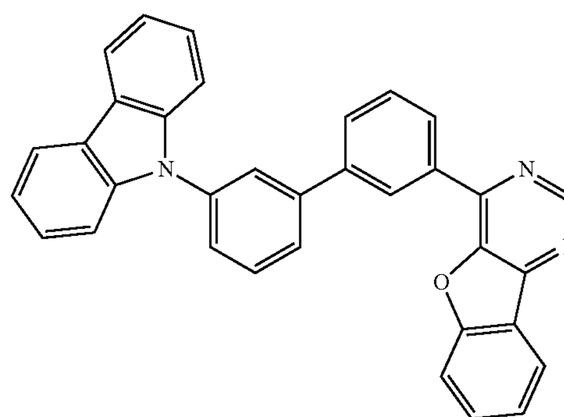
4mCzBPBfPm
