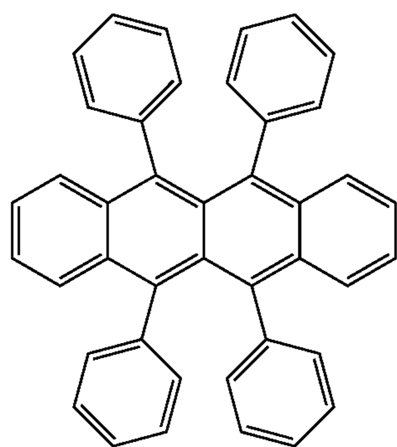
Rubrene
