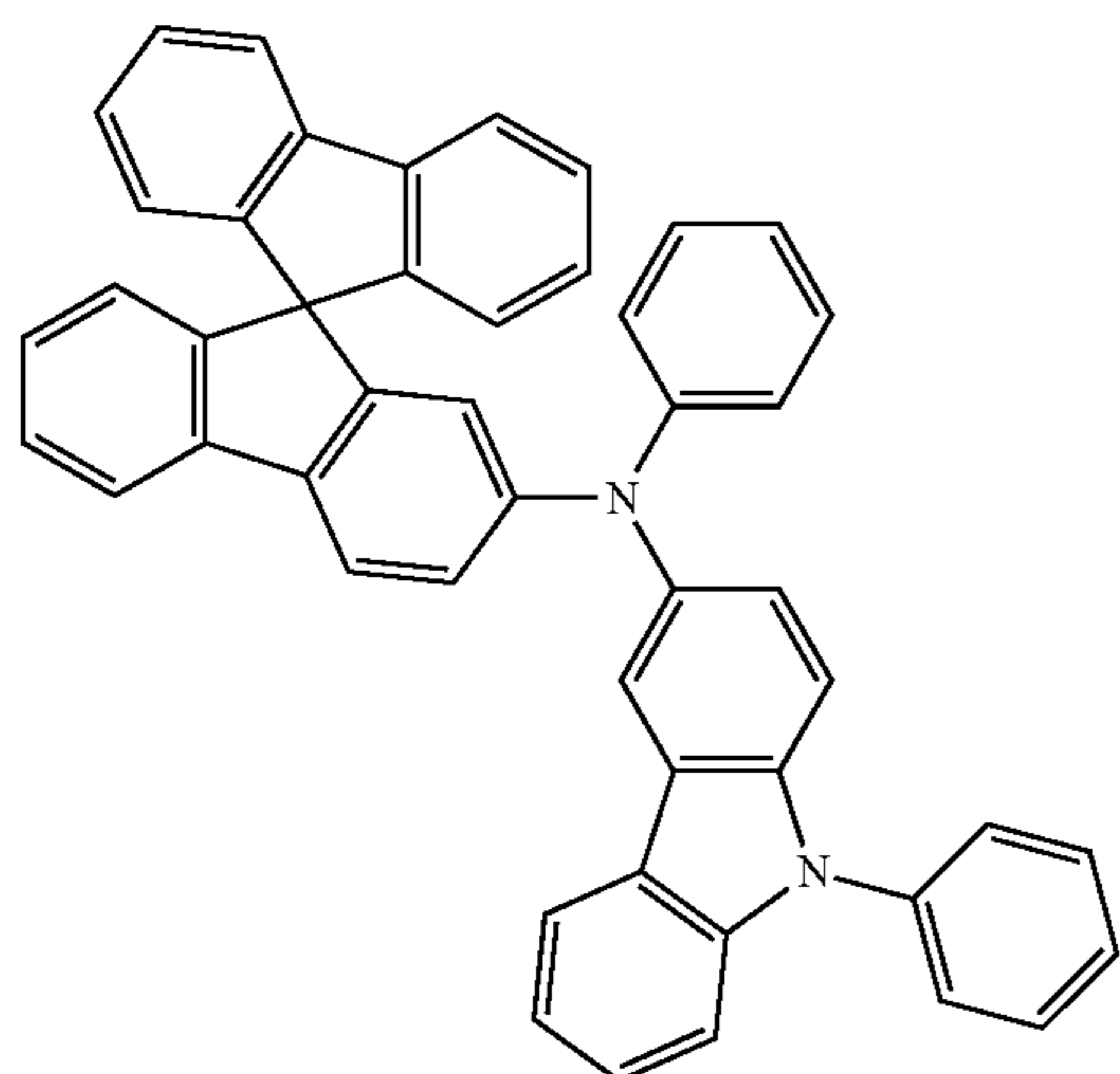
PCASF
