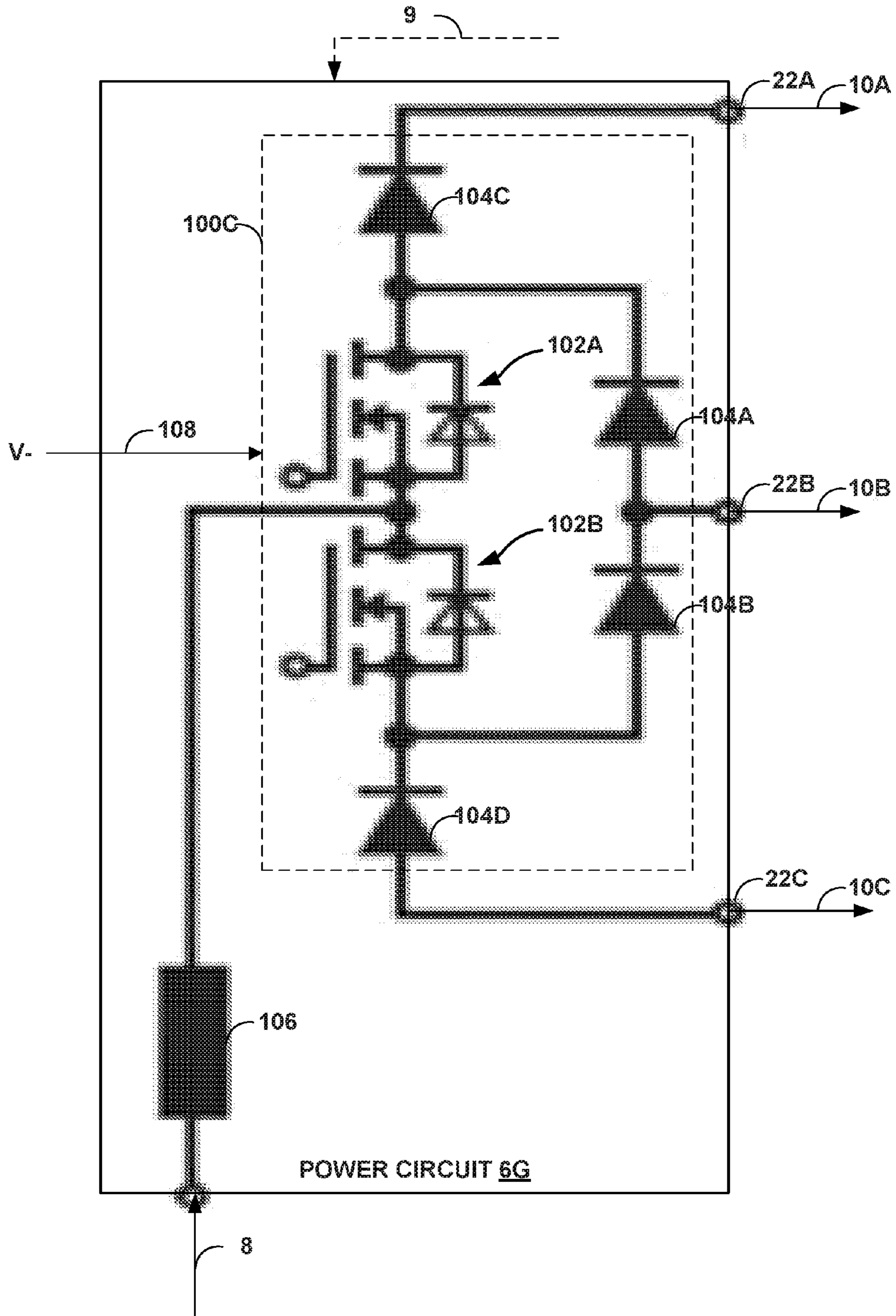
FIG. 8C
