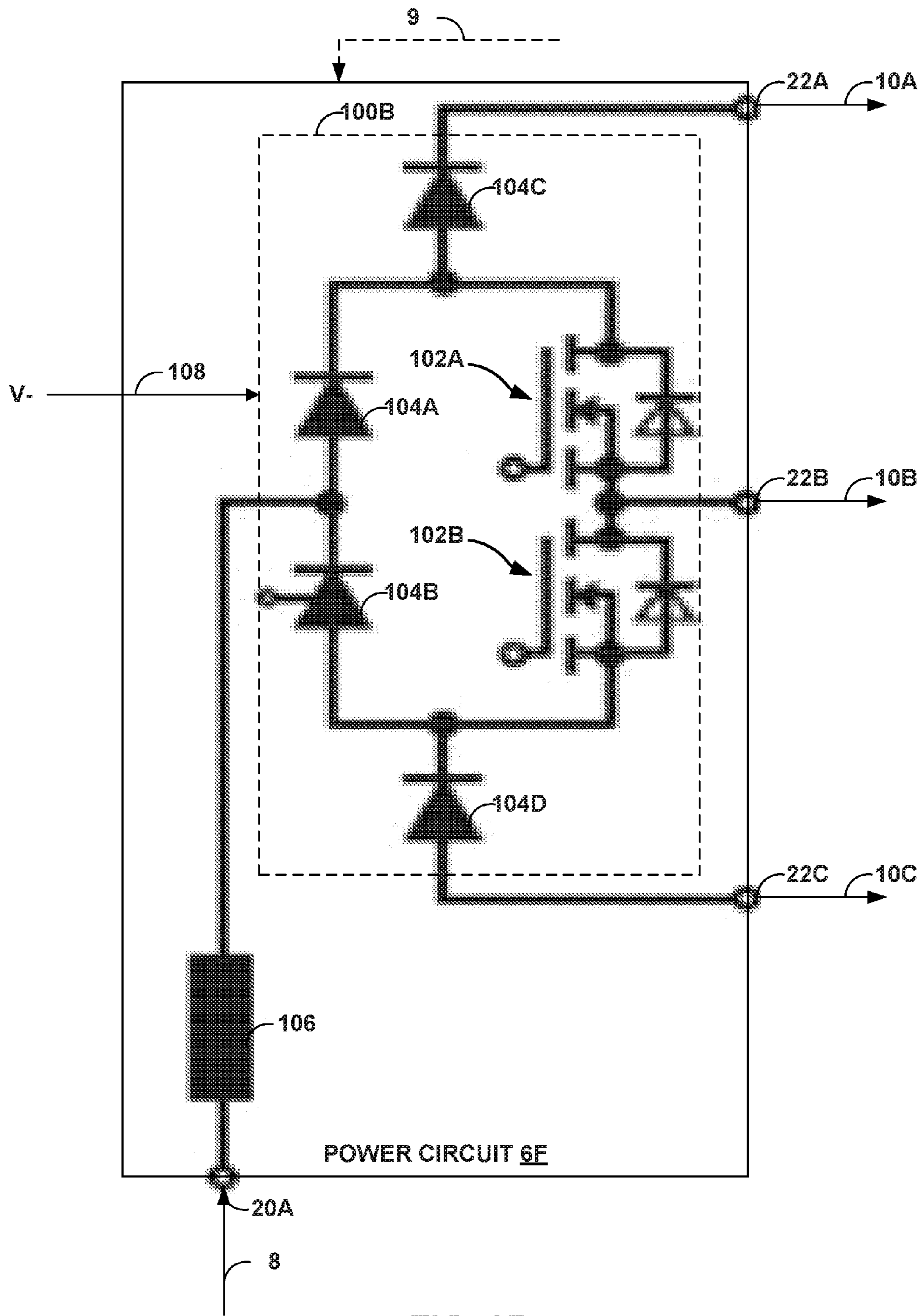
FIG. 8B
