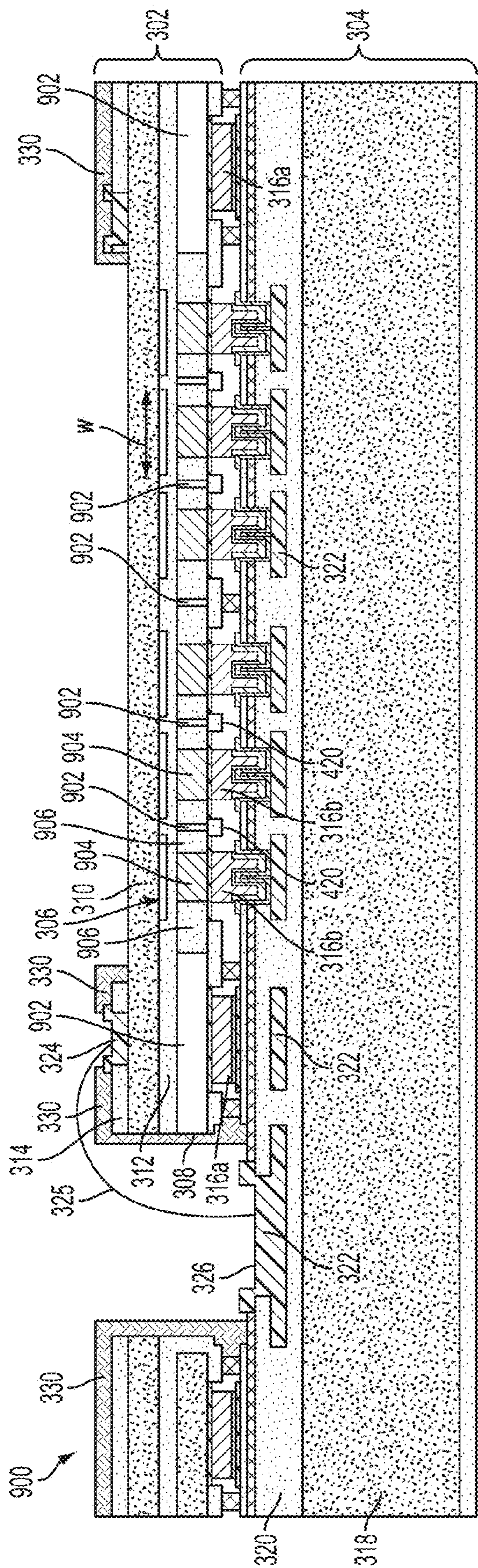
FIG. 9
