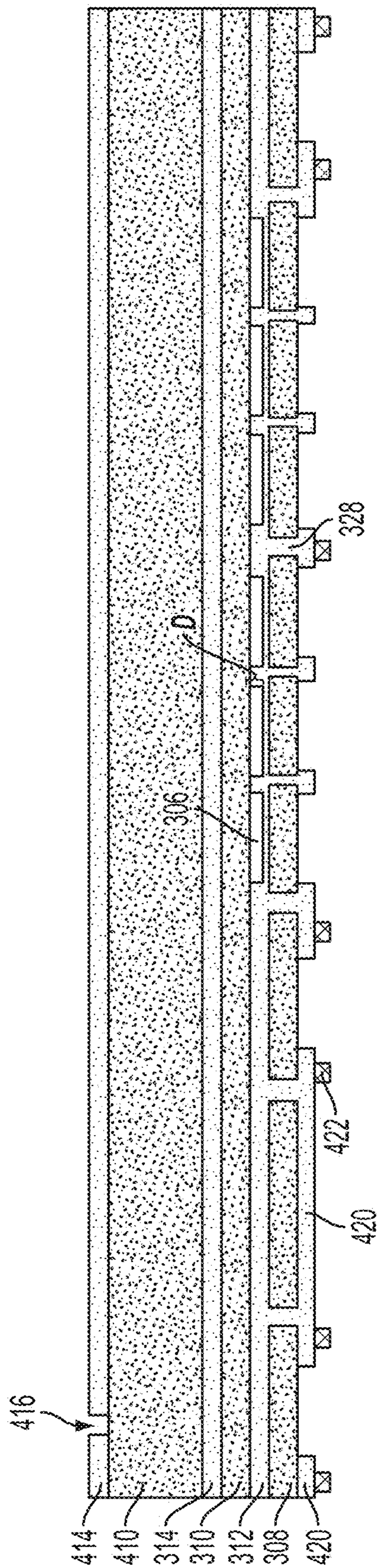
FIG. 4J
