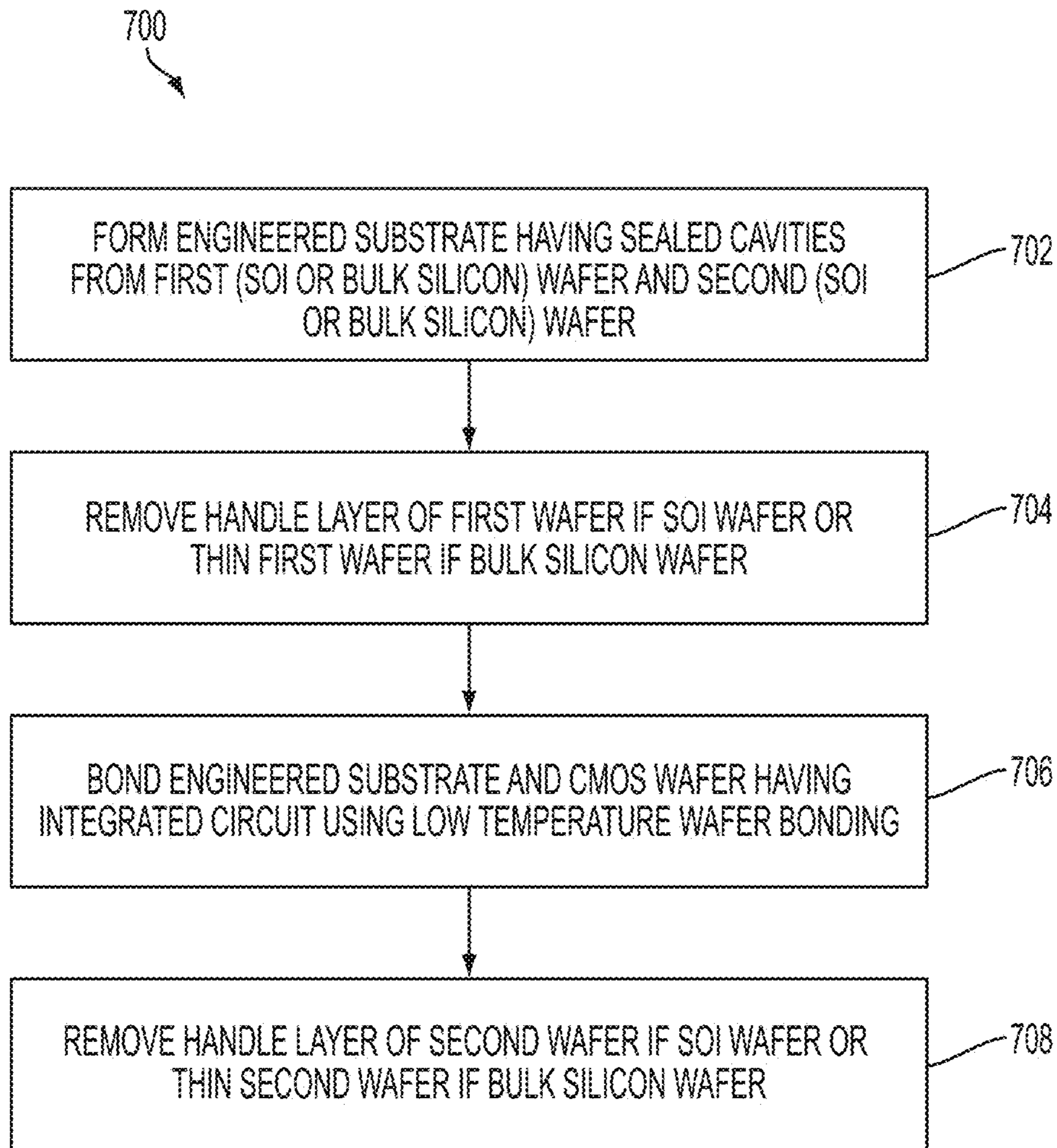
FIG. 7
