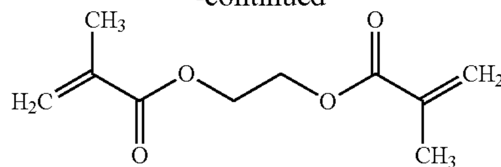
EGDMA
