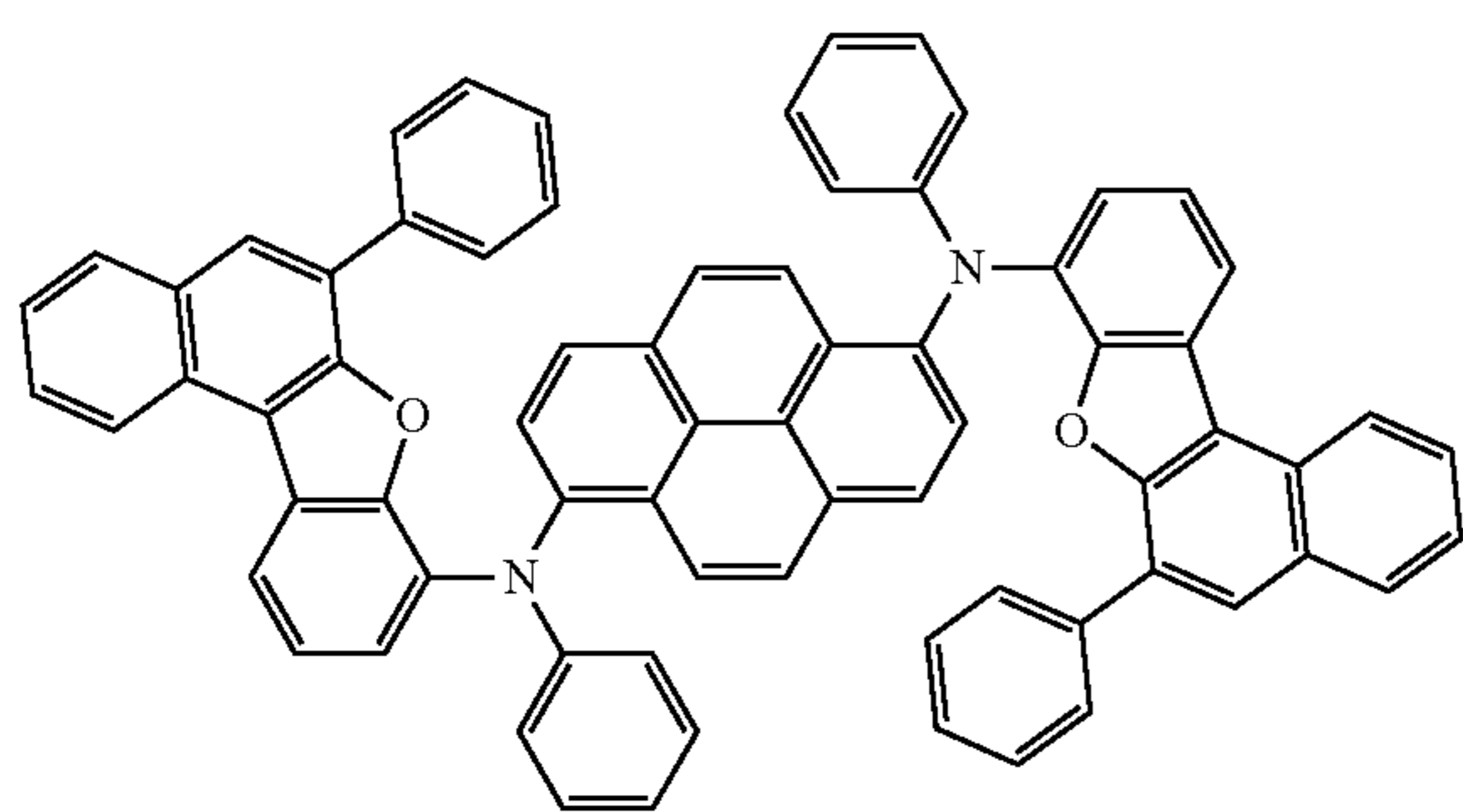
1,6BnfAPrn-03
