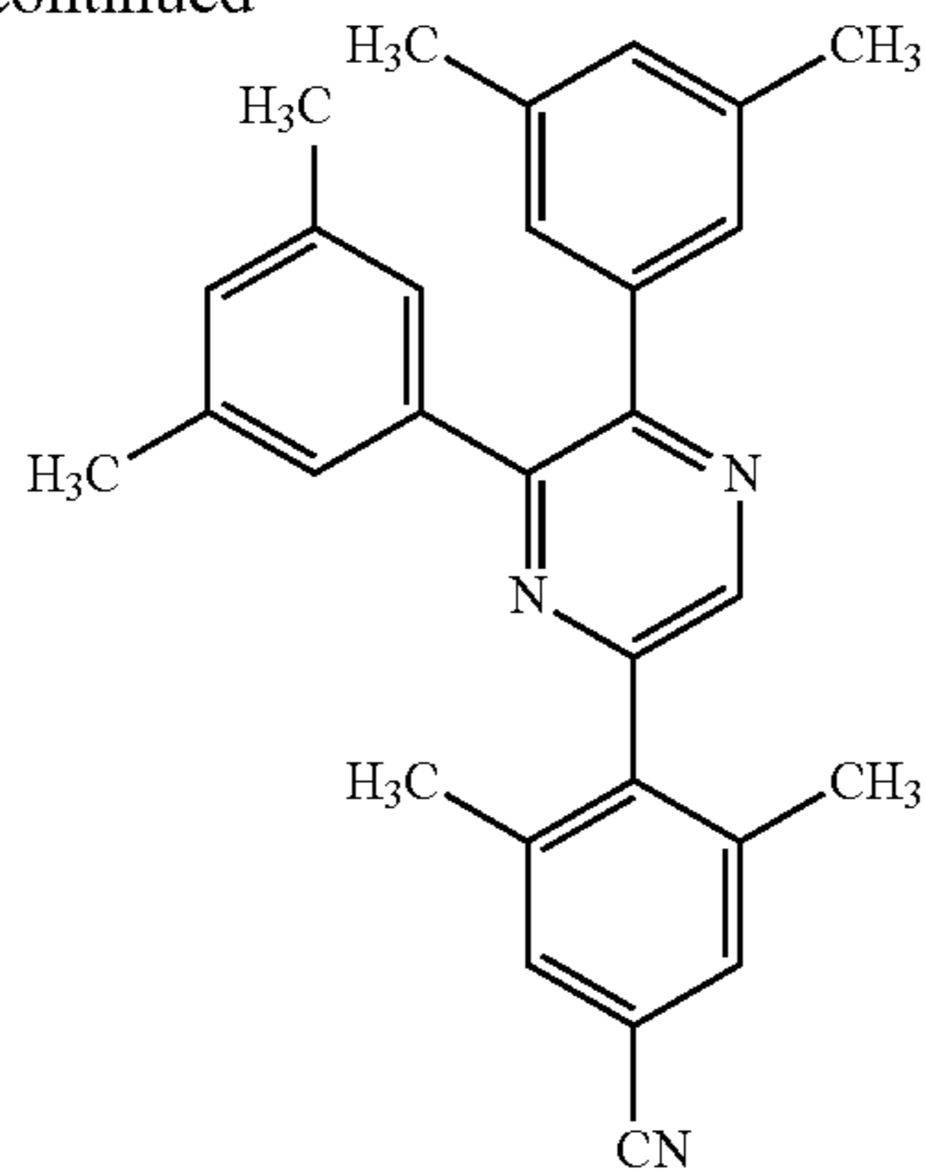
Hdmdppr-dmCP (a-3)
