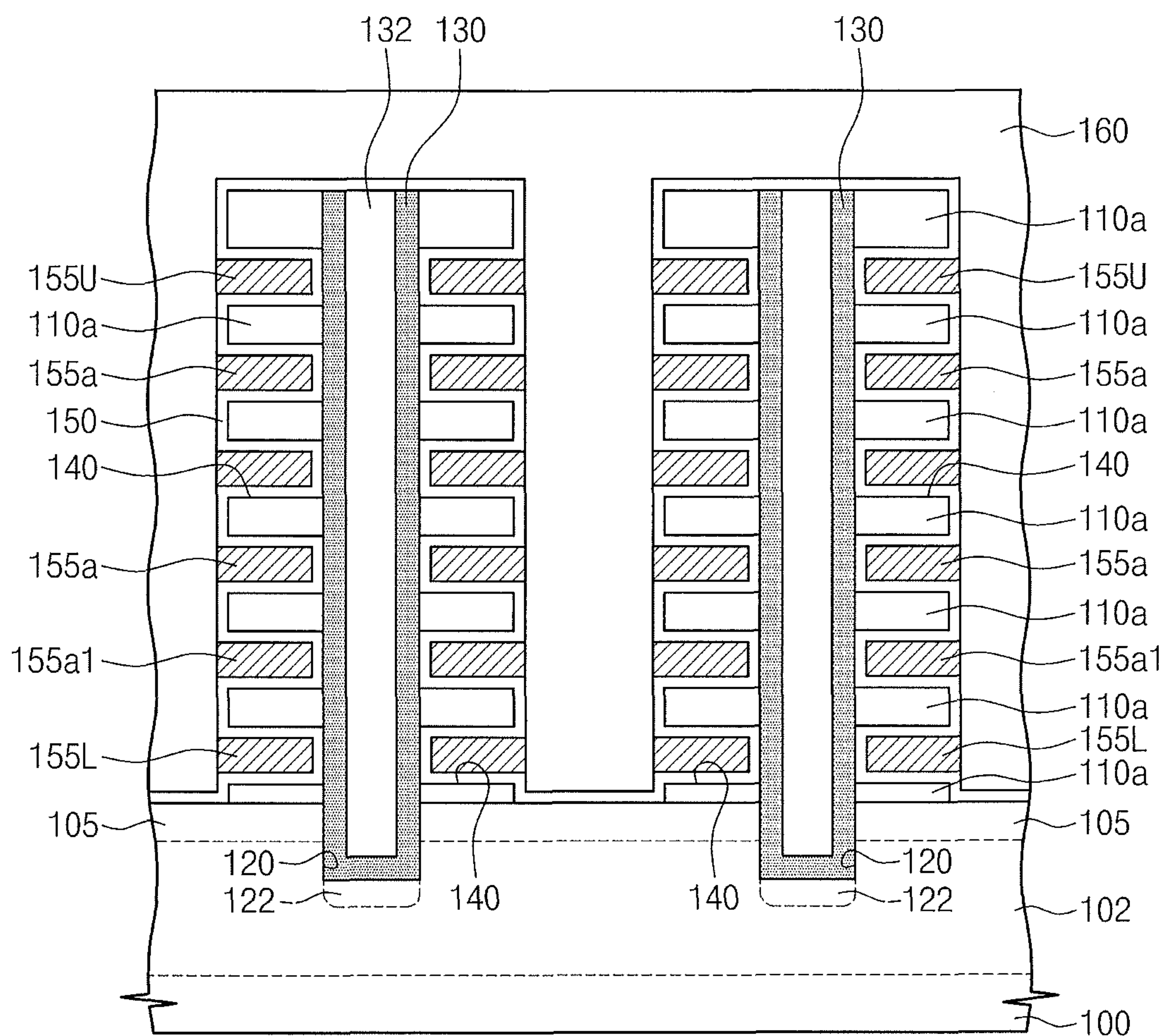
Fig. 6G
