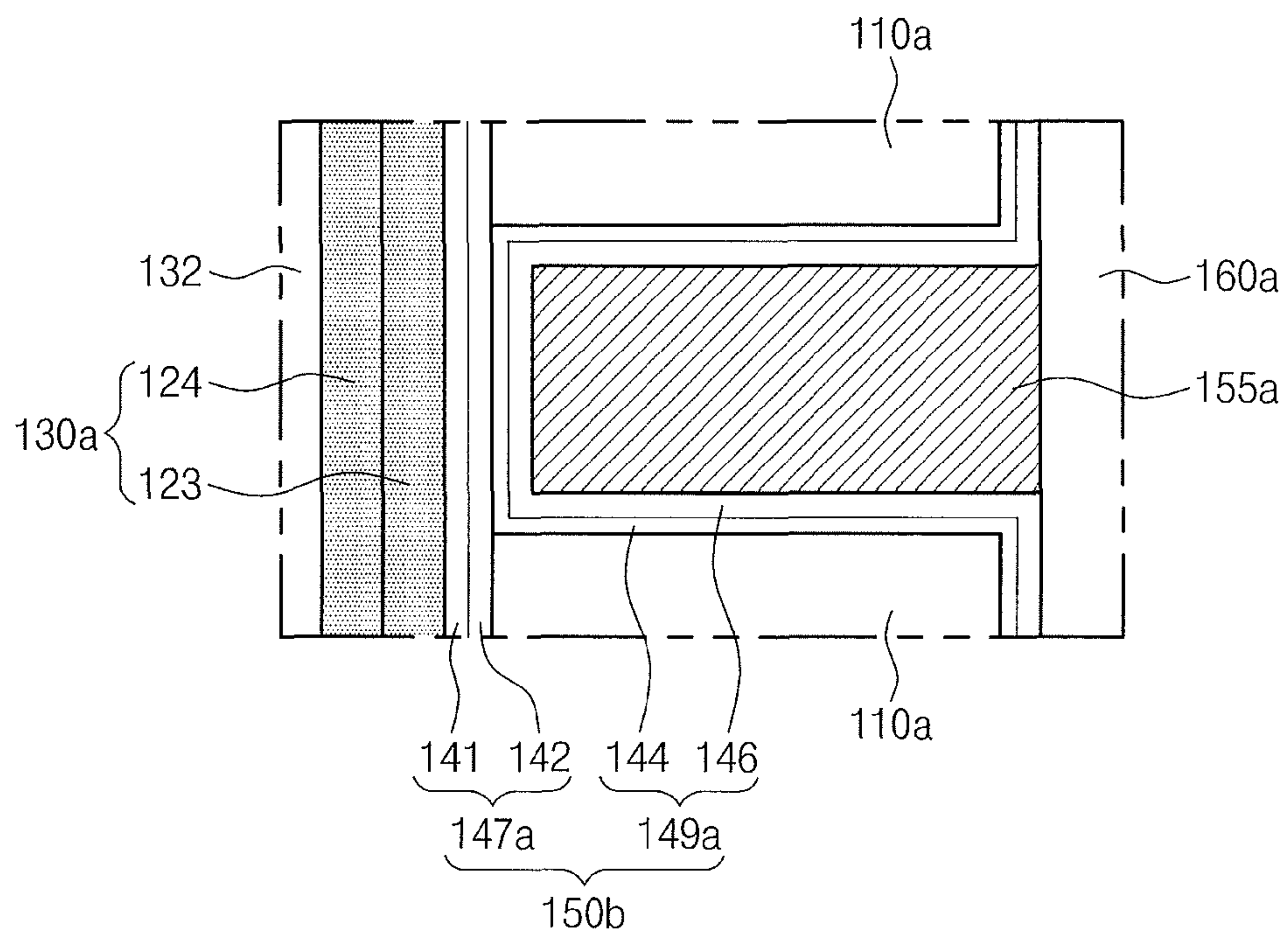
Fig. 3C
