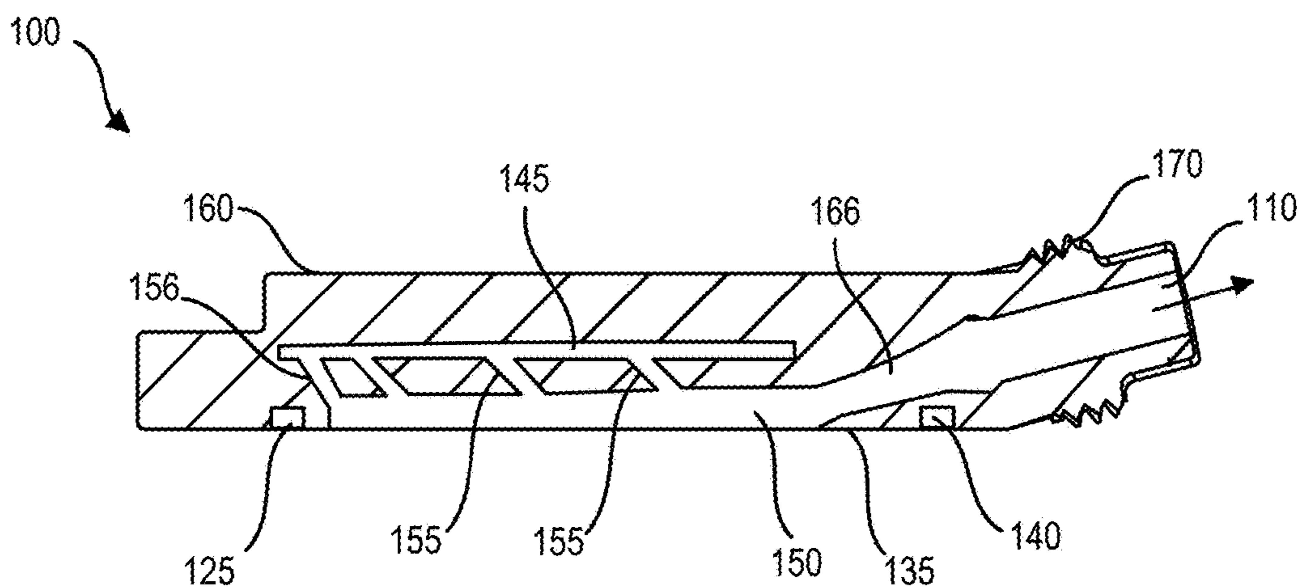
SECTION A-A
