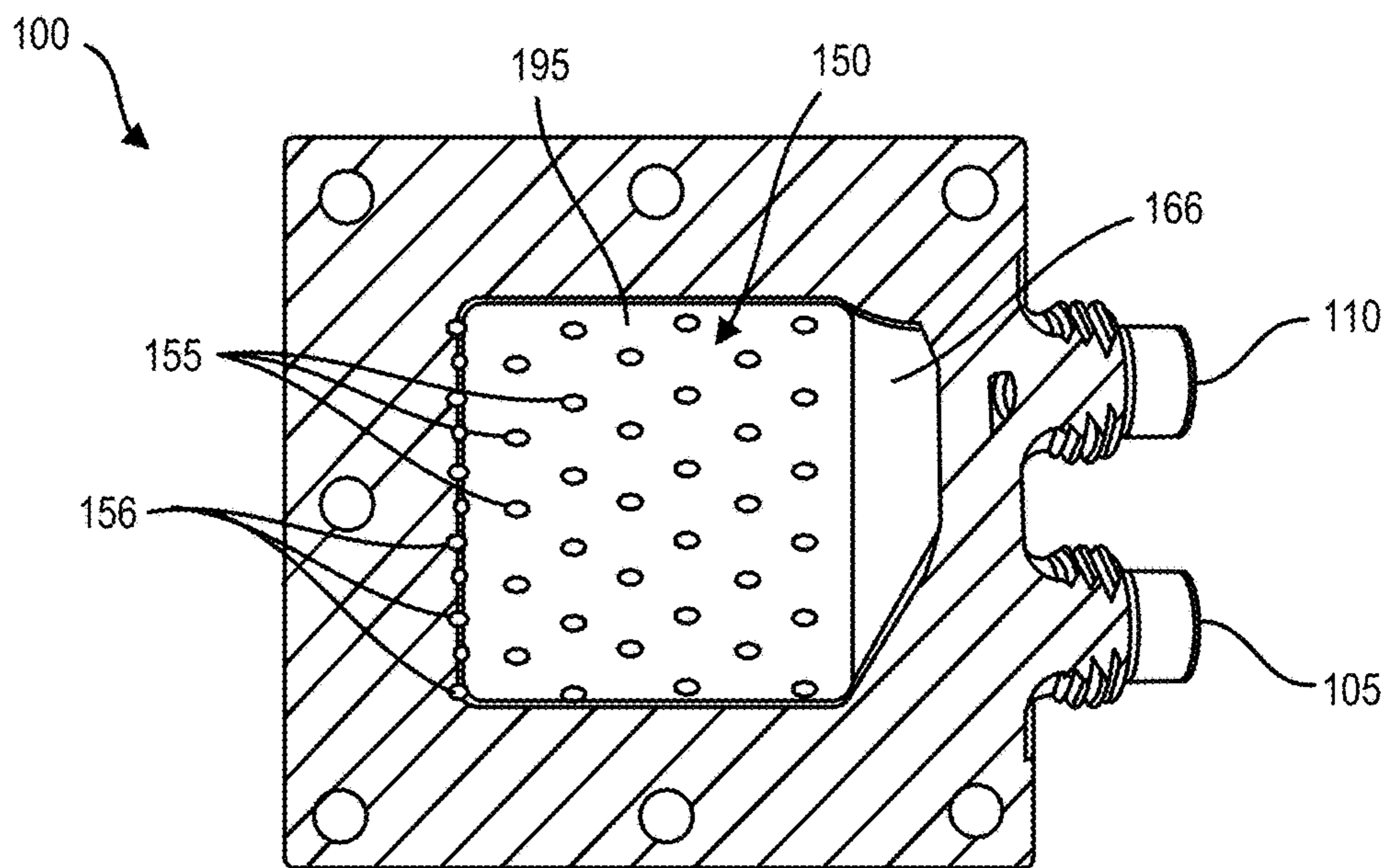
SECTION D-D
