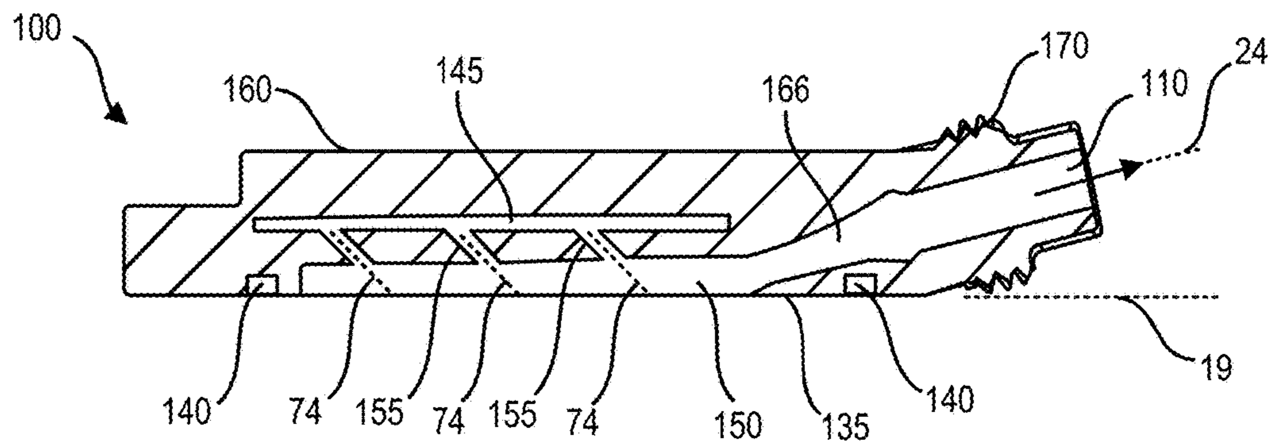
SECTION A-A
