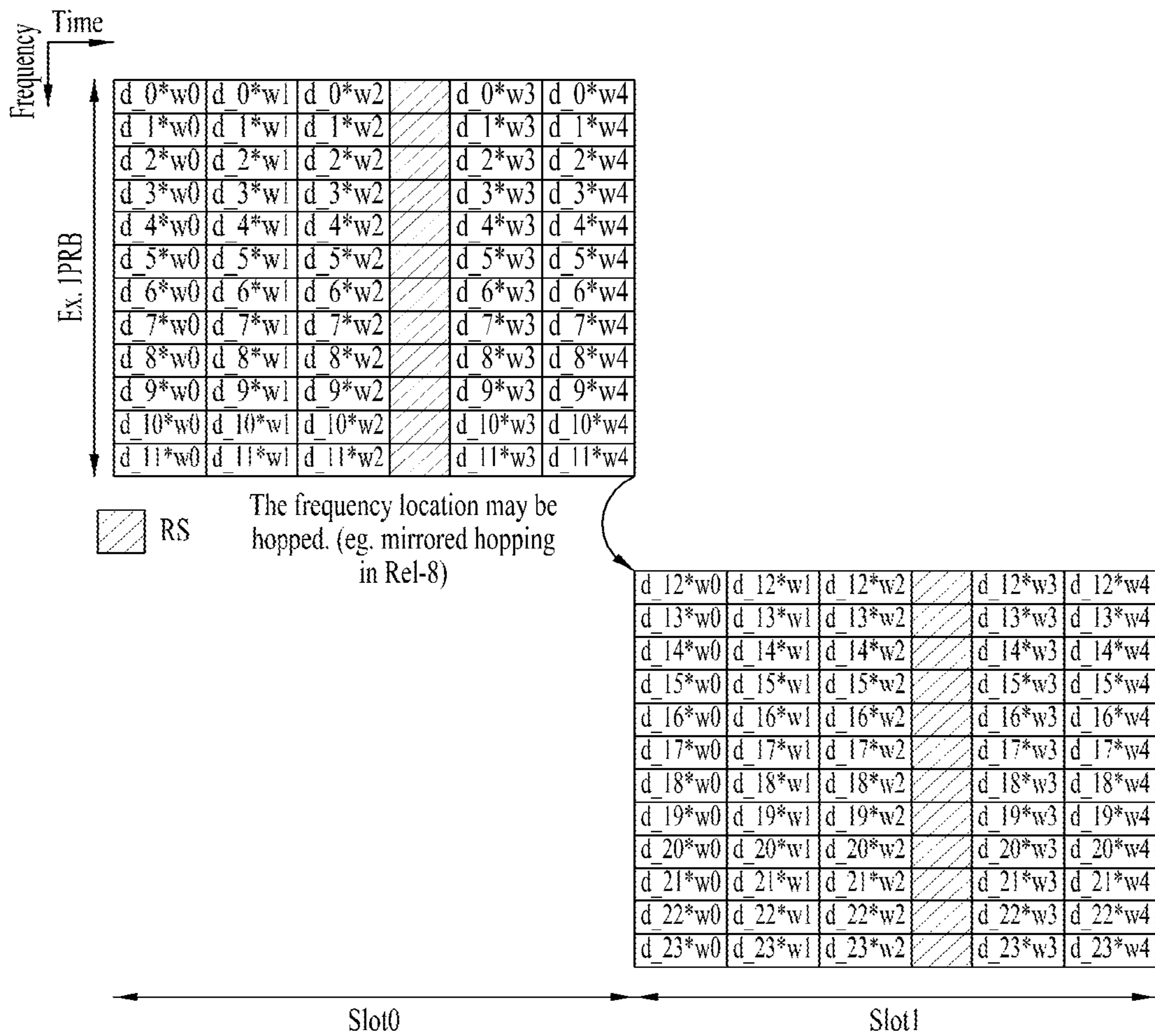
Reuse of LTE PUCCH format 2 structure (extended CP case)
