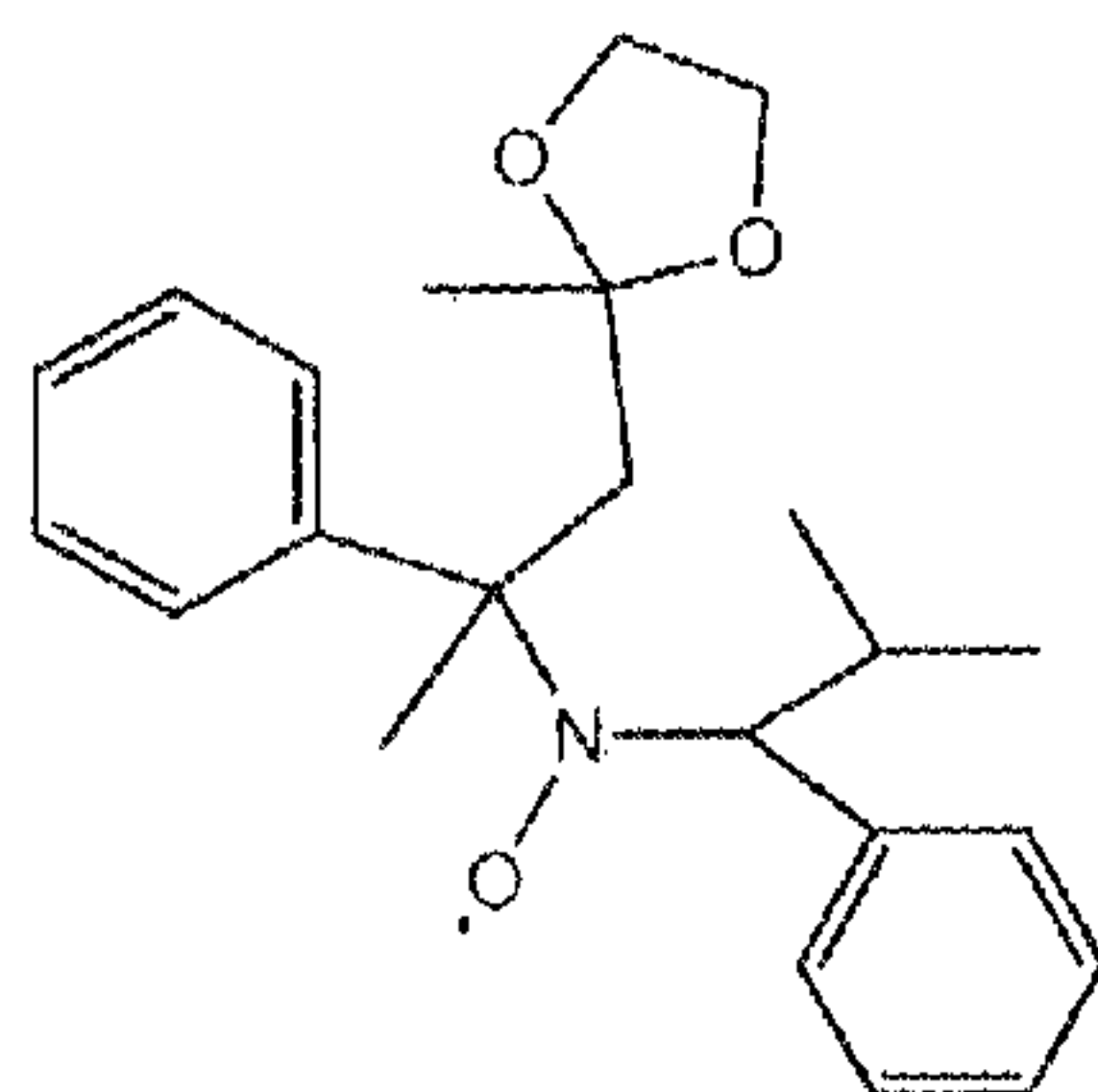
TIPNO-3, LogP=4.8
