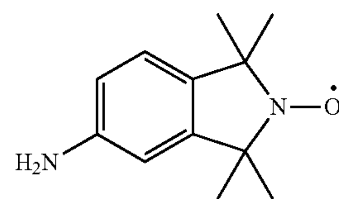
5-amino-TMIO
