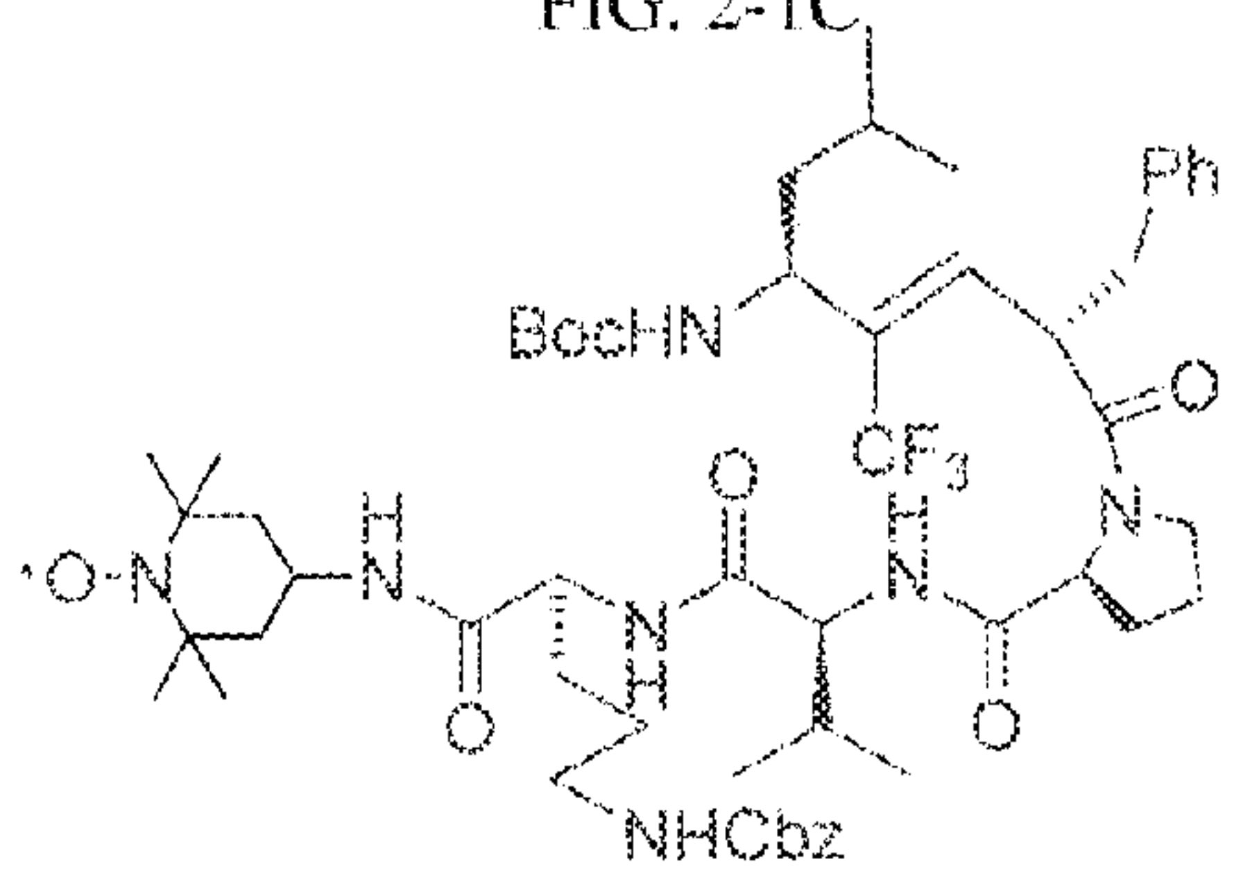
XJB-7-55
