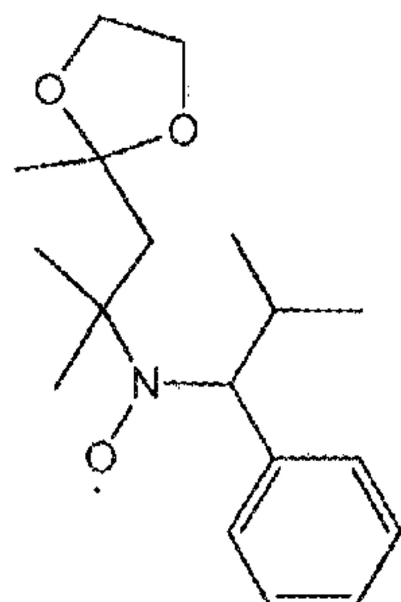
TIPNO-2, LogP=3.6
