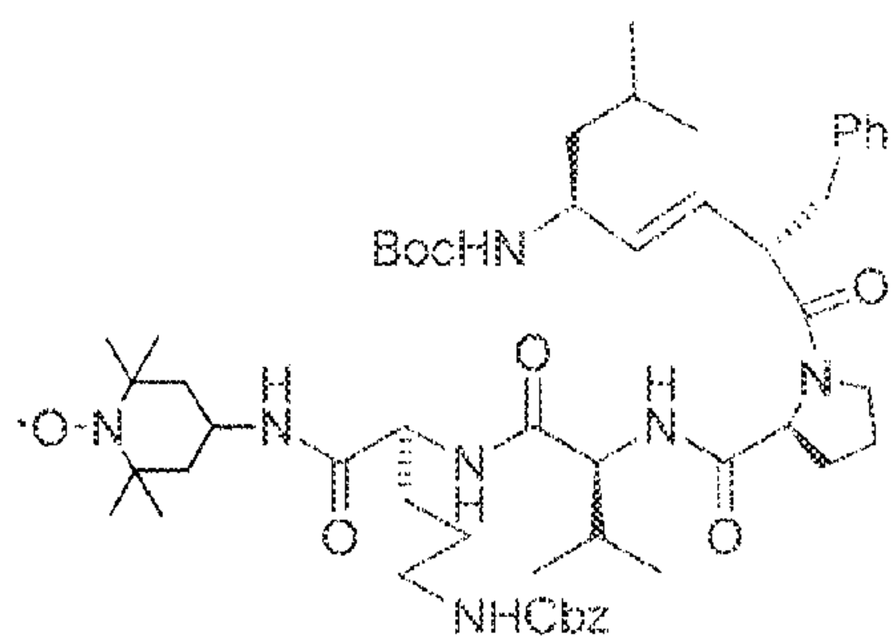
XJB-5-131
