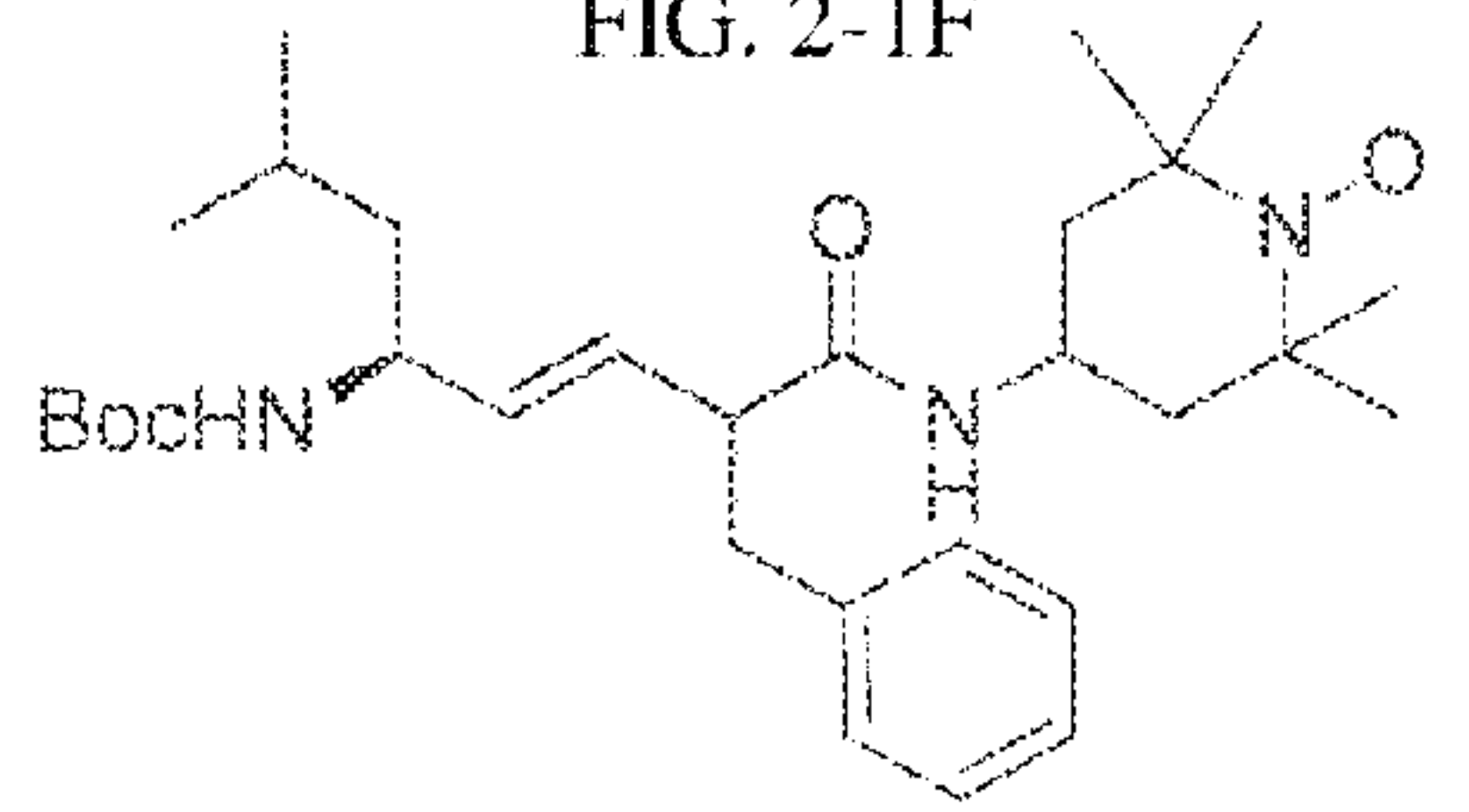
JP4-049
