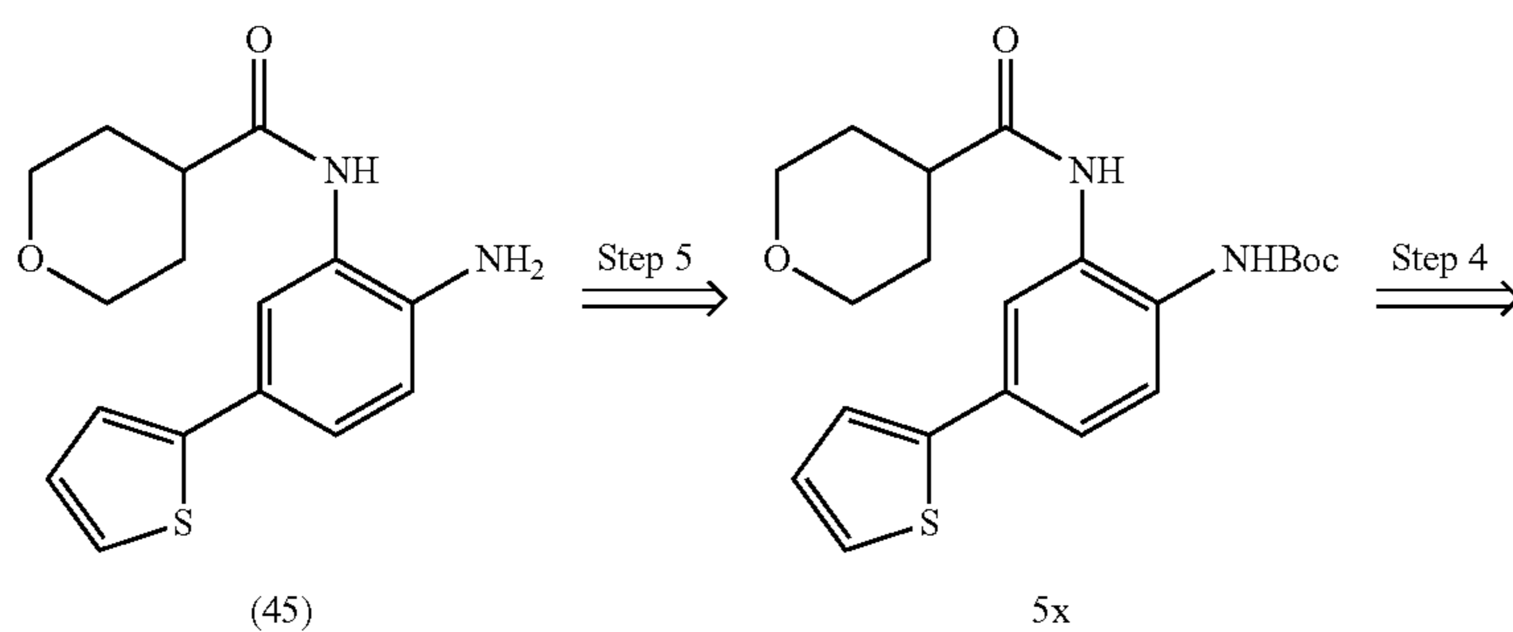
Scheme 1A
