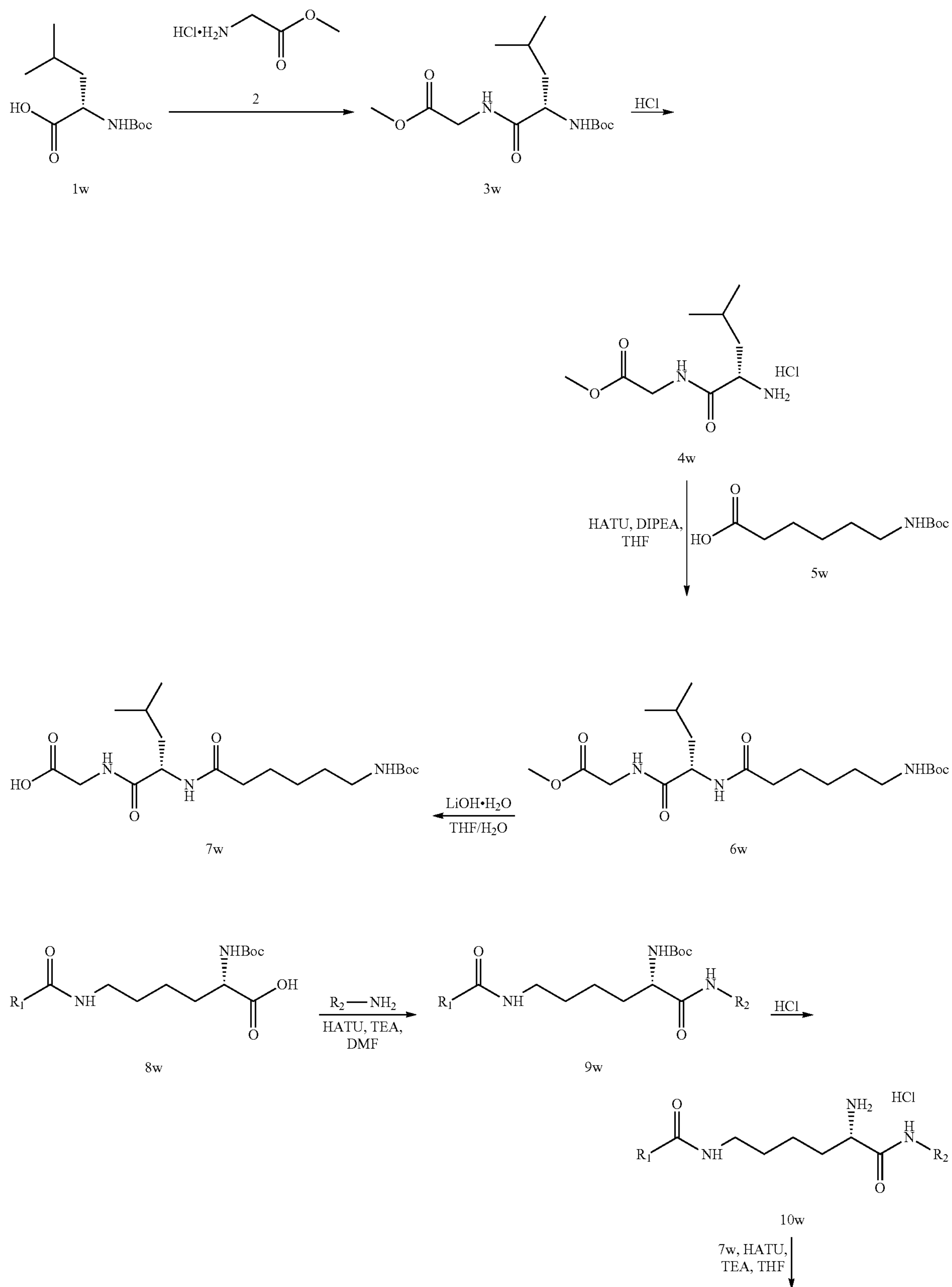
Scheme 1X
