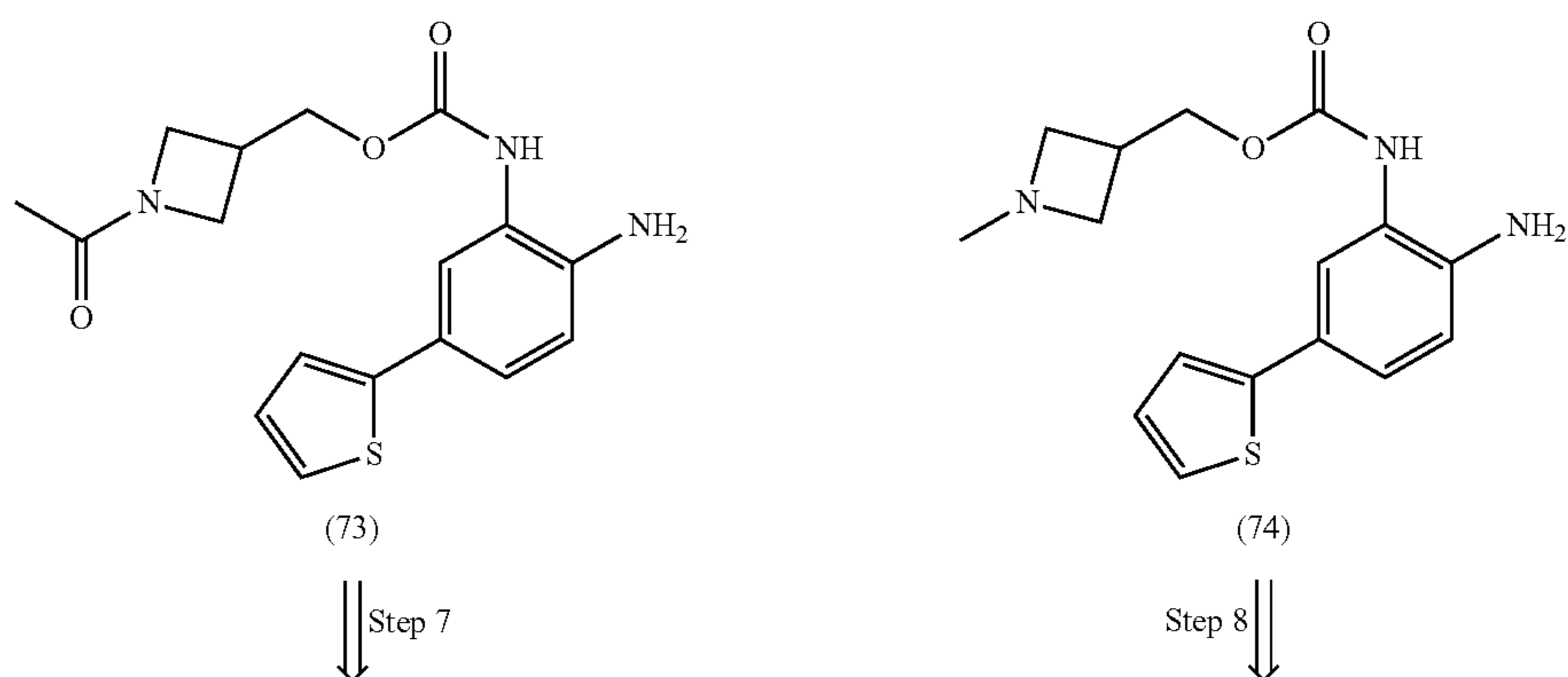
Scheme 2A
