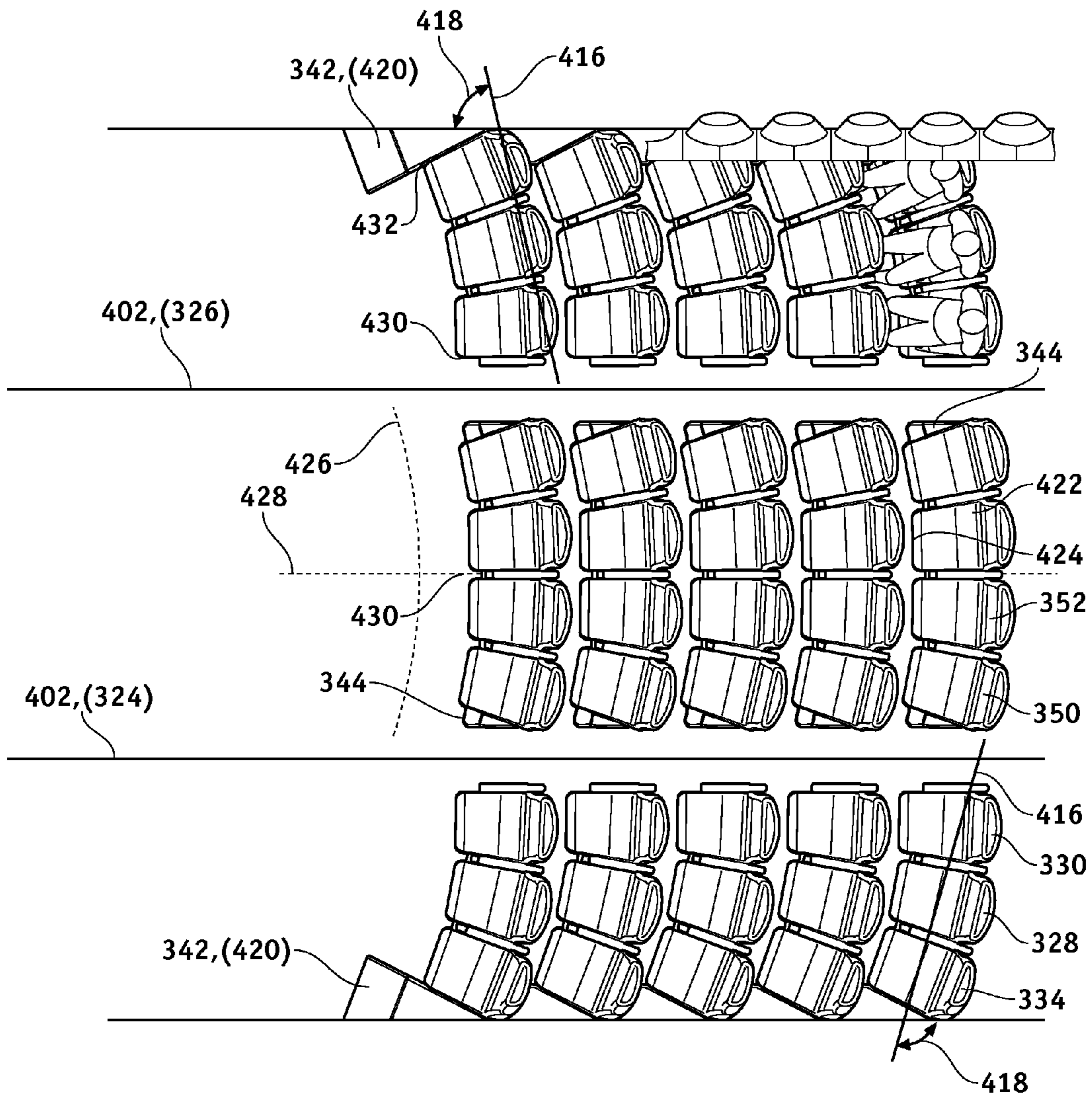
FIG. 4A
