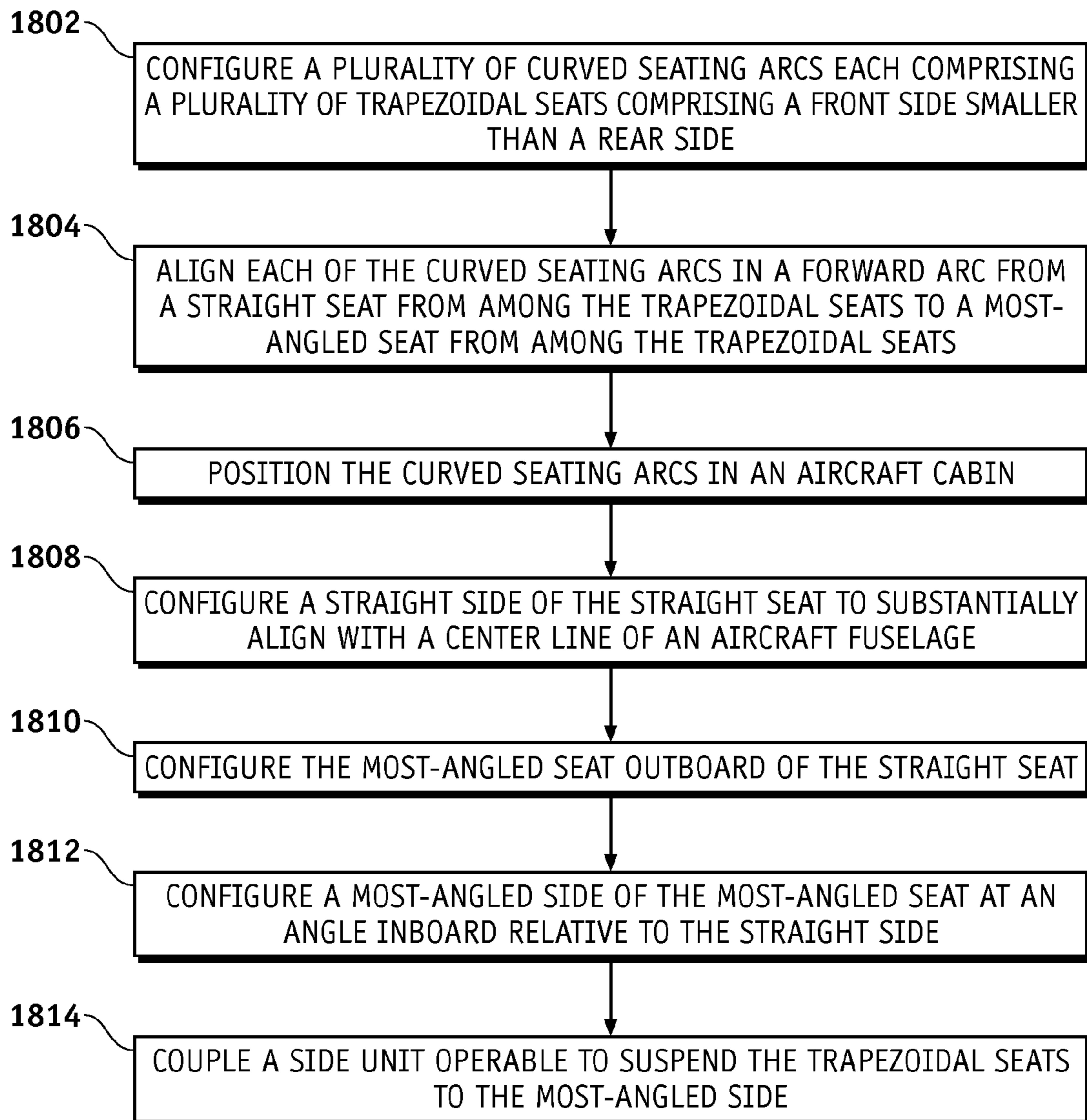
FIG. 18
