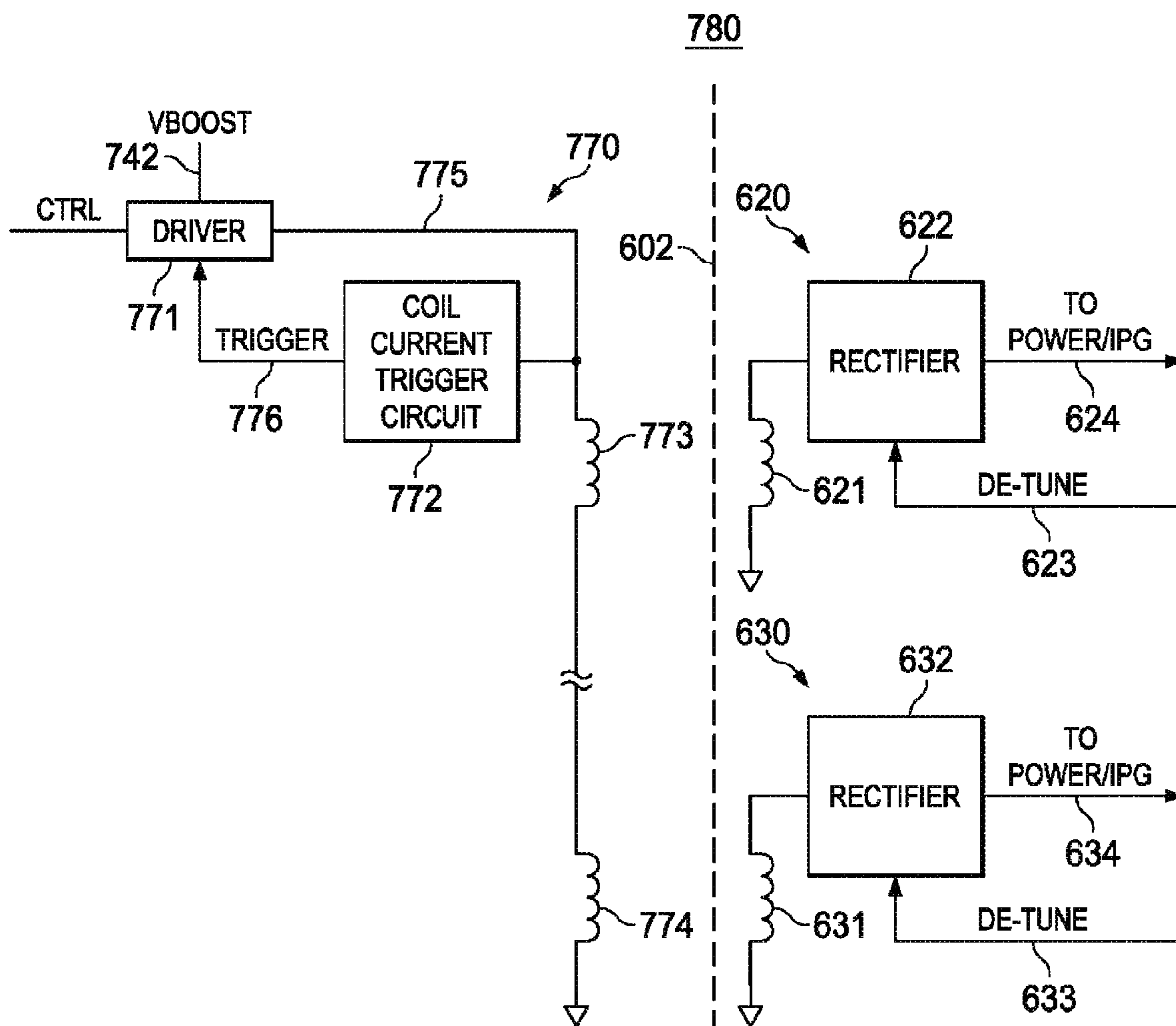
FIG. 16A
