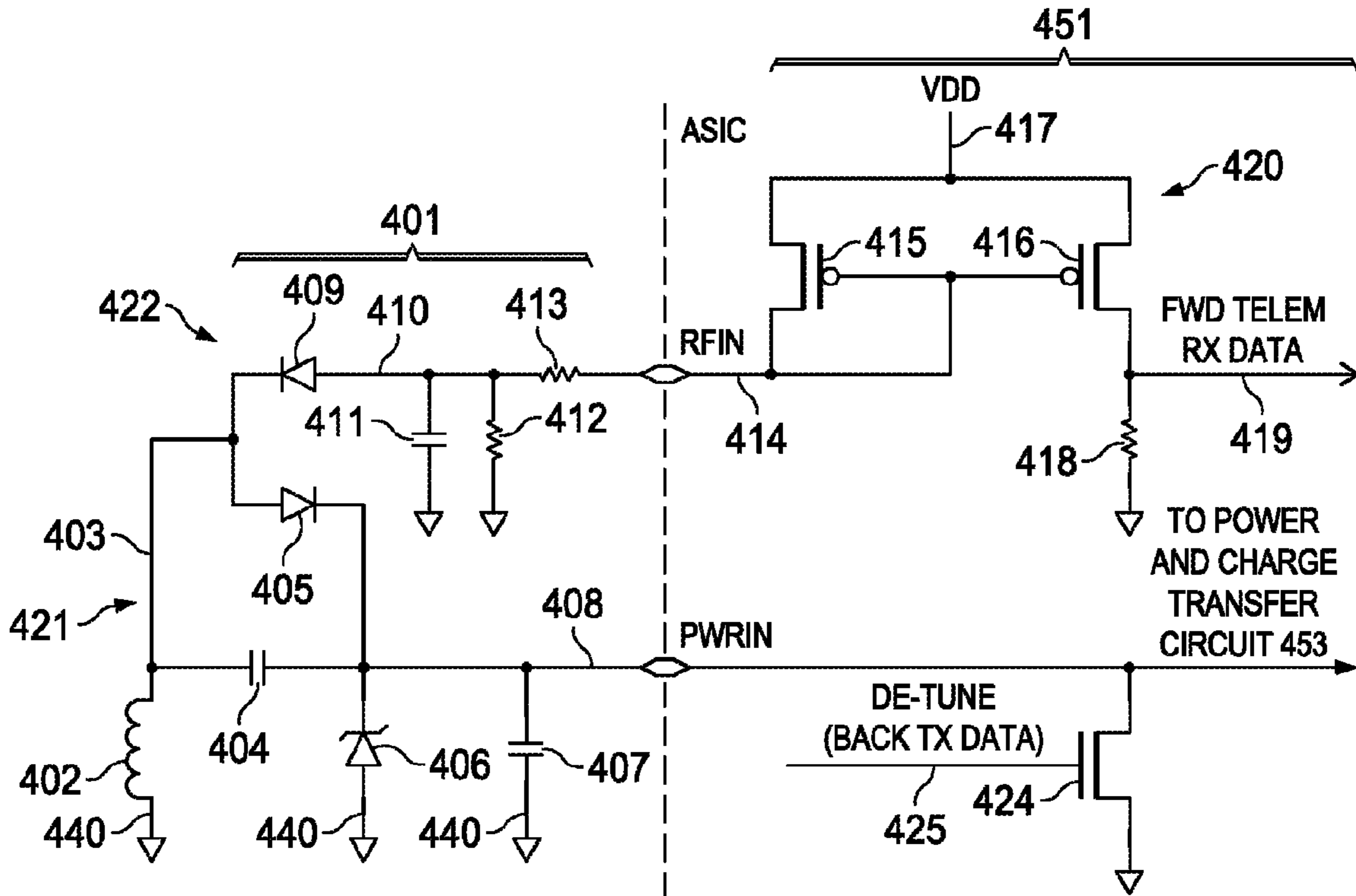
FIG. 23A
