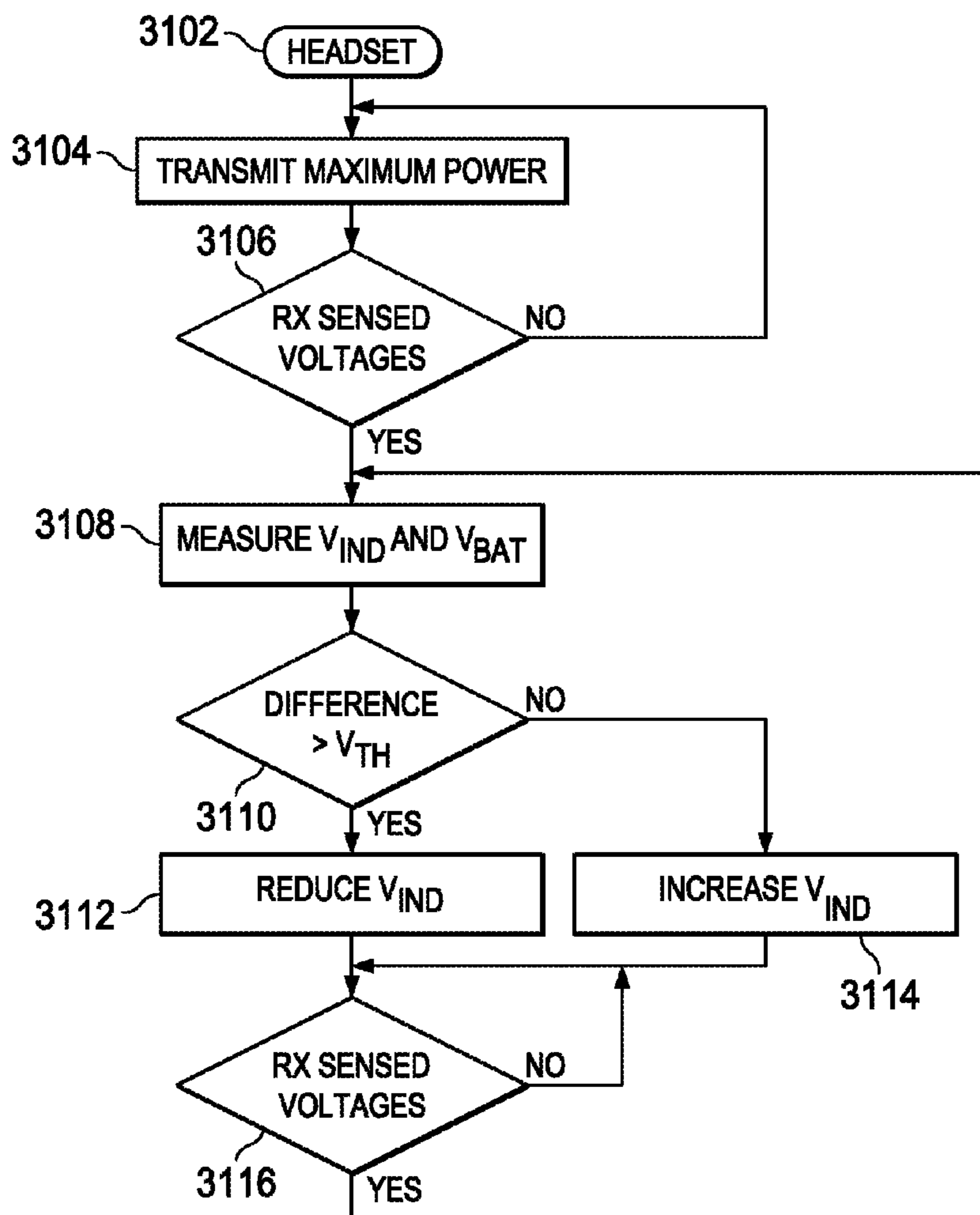
FIG. 31
