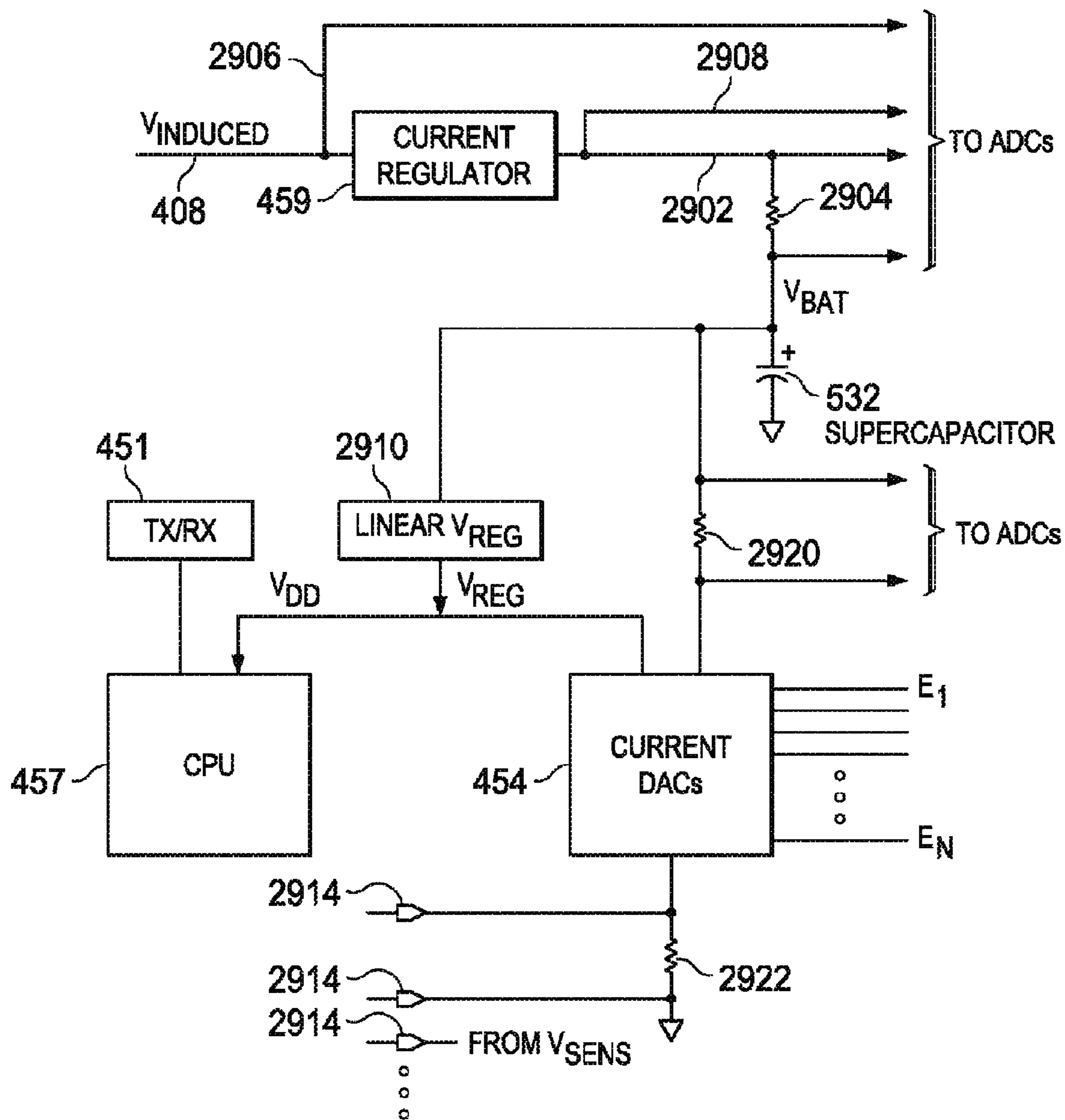
FIG. 29
