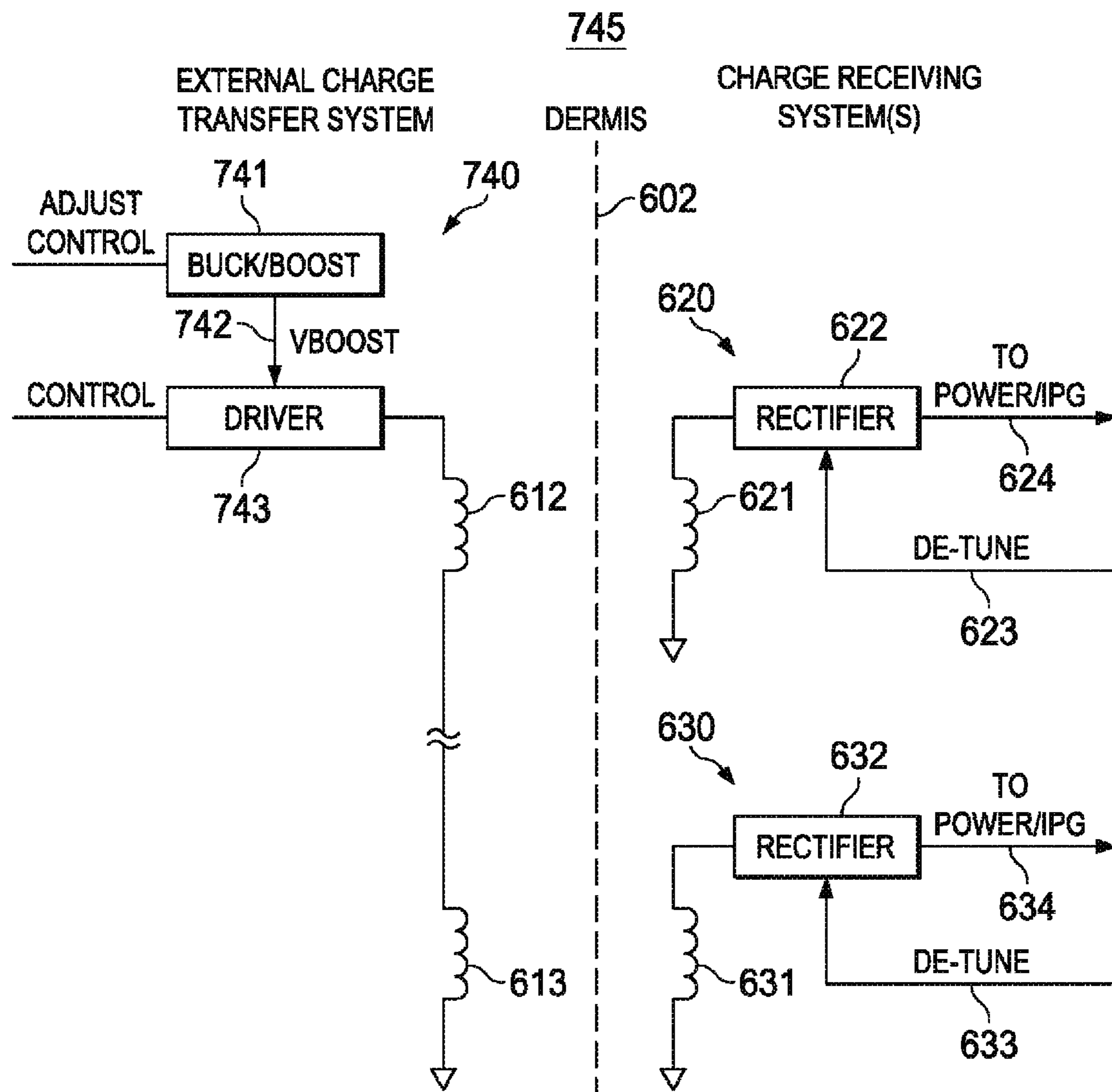
FIG. 15
