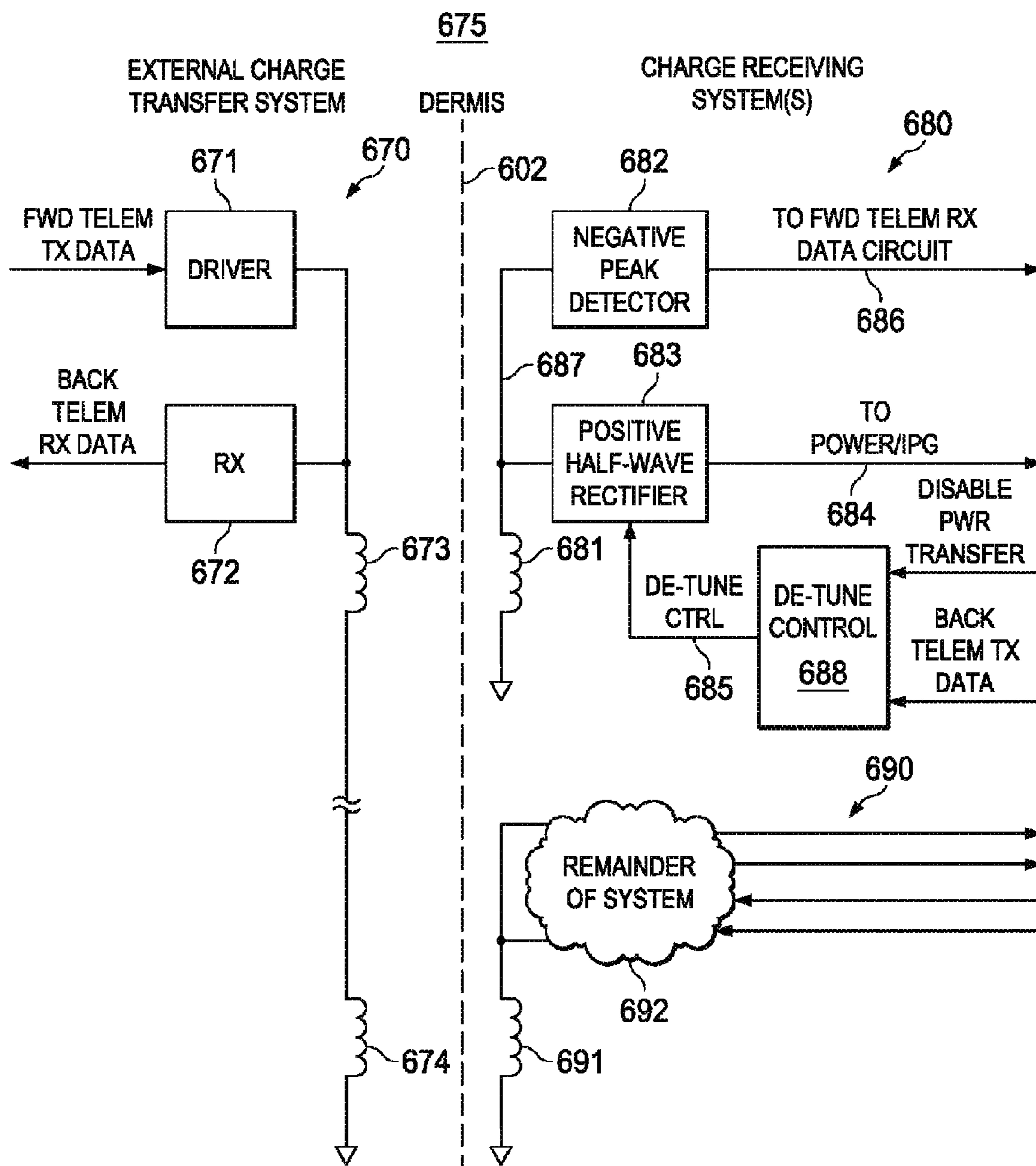
FIG. 13A
