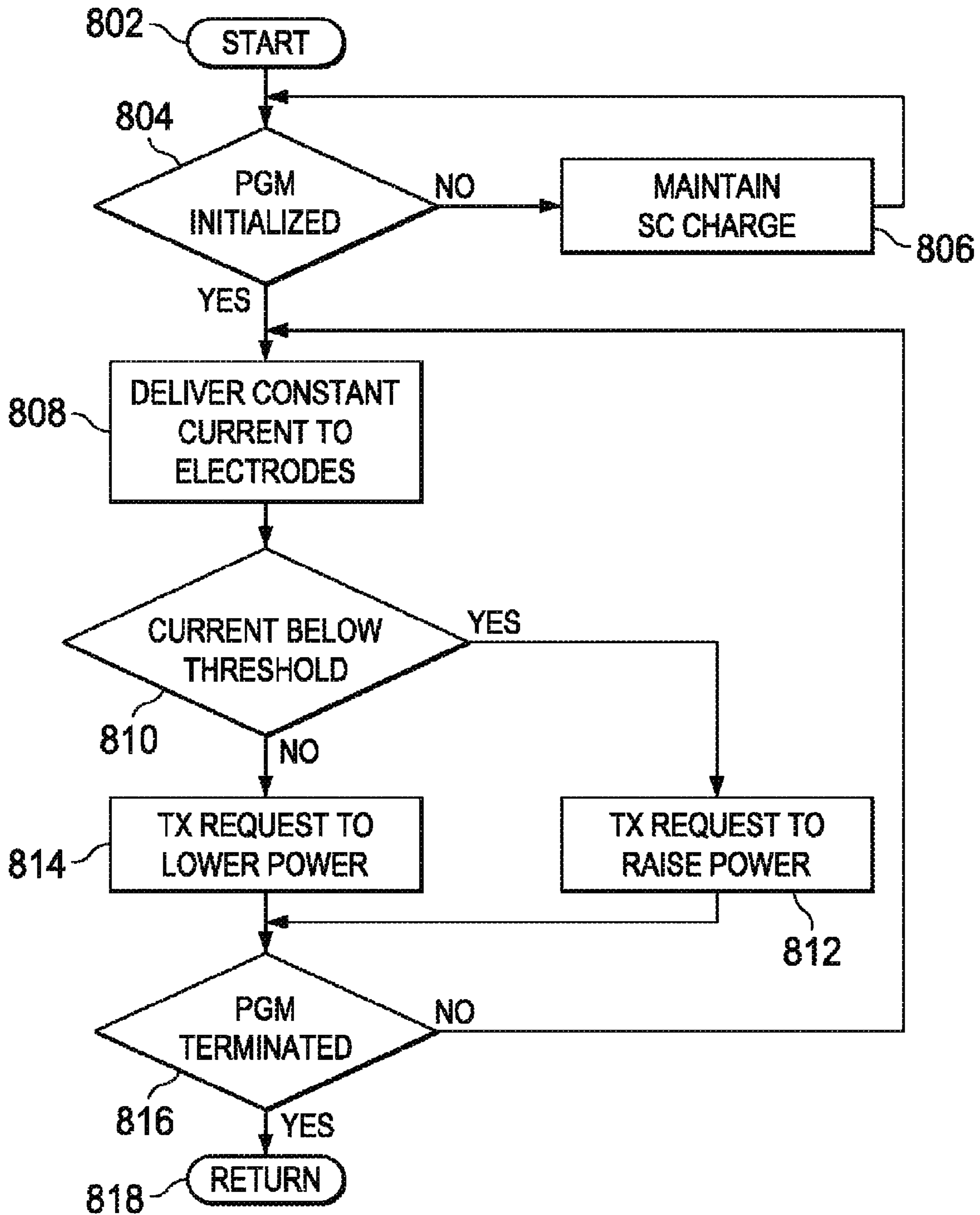
FIG. 22B
