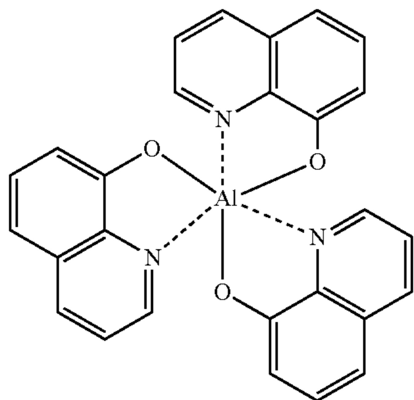
Alq 3
