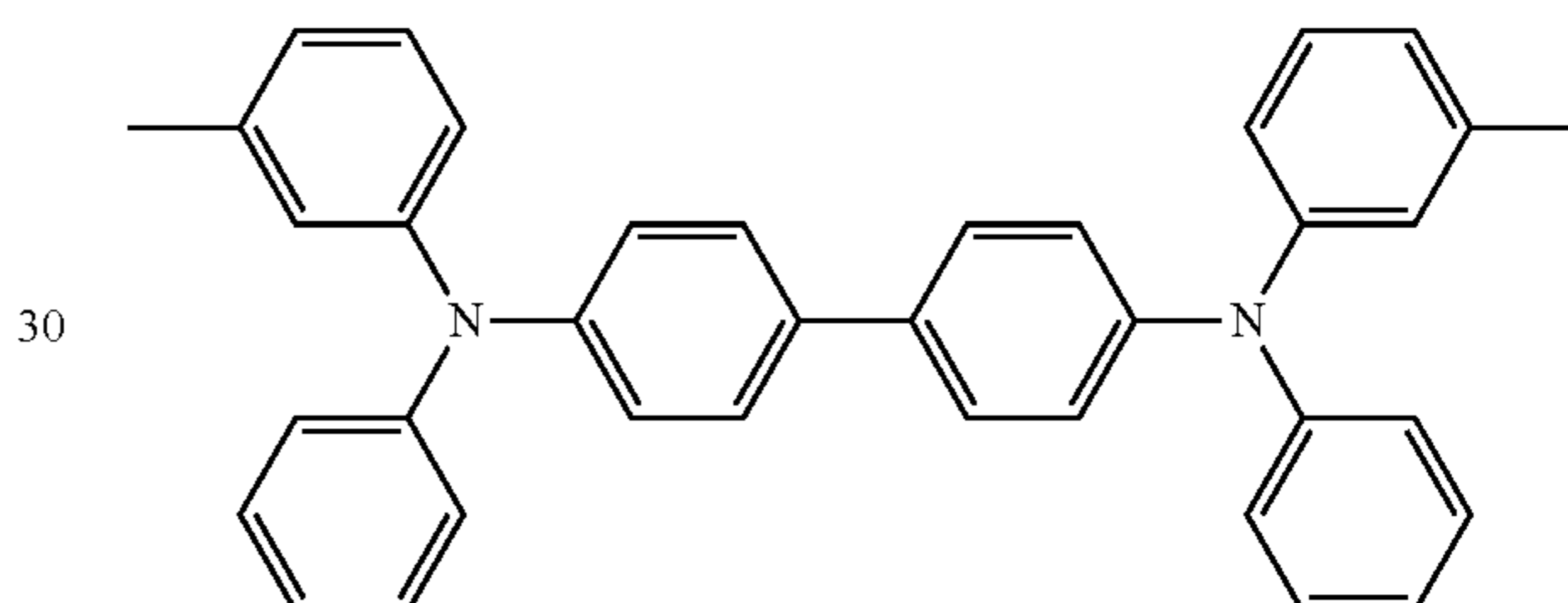
TPD
