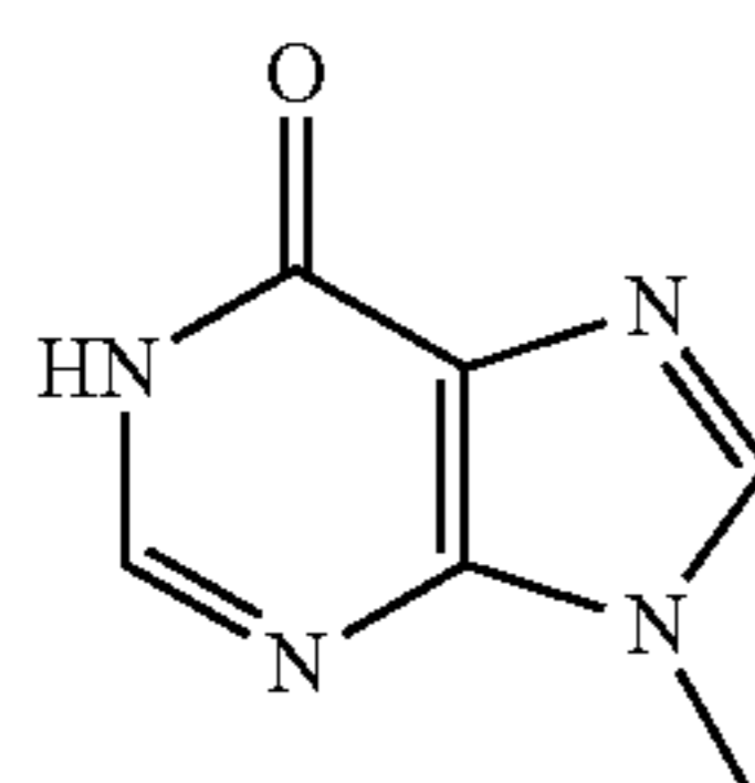
Inosine
