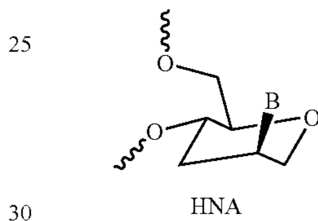
2'-AP
