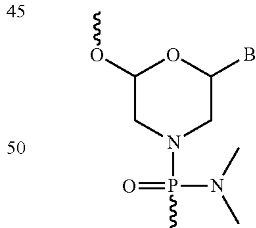
Morpholino
