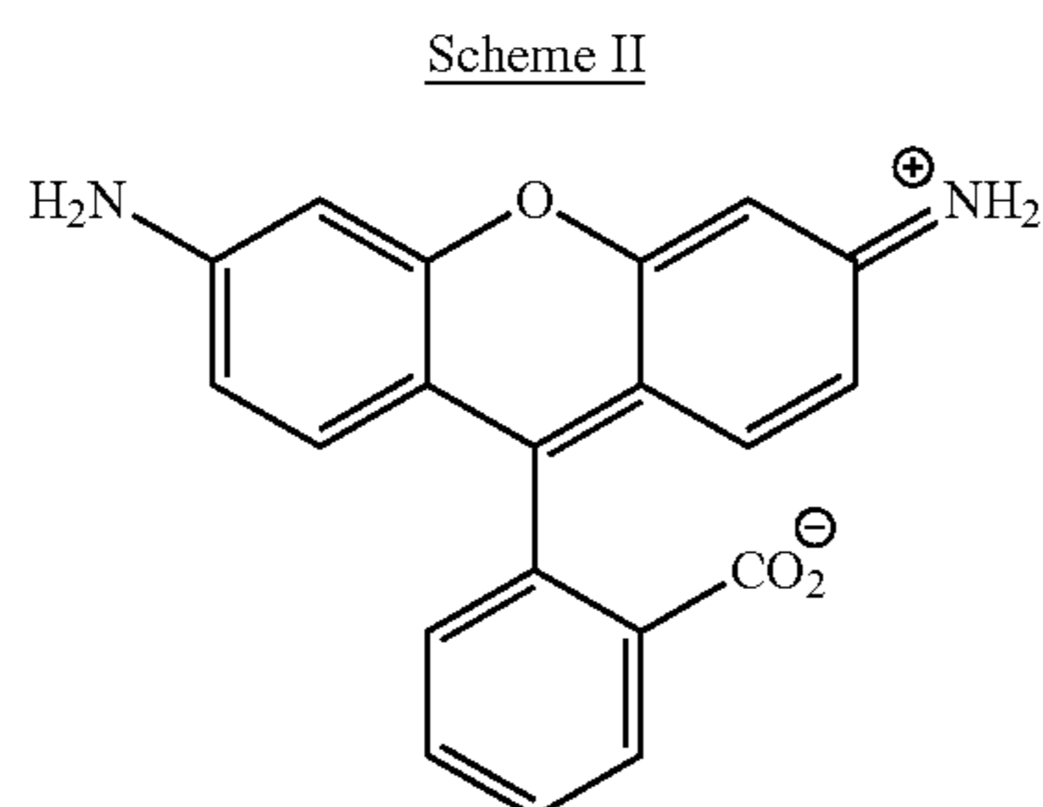
Rhodamine 110
