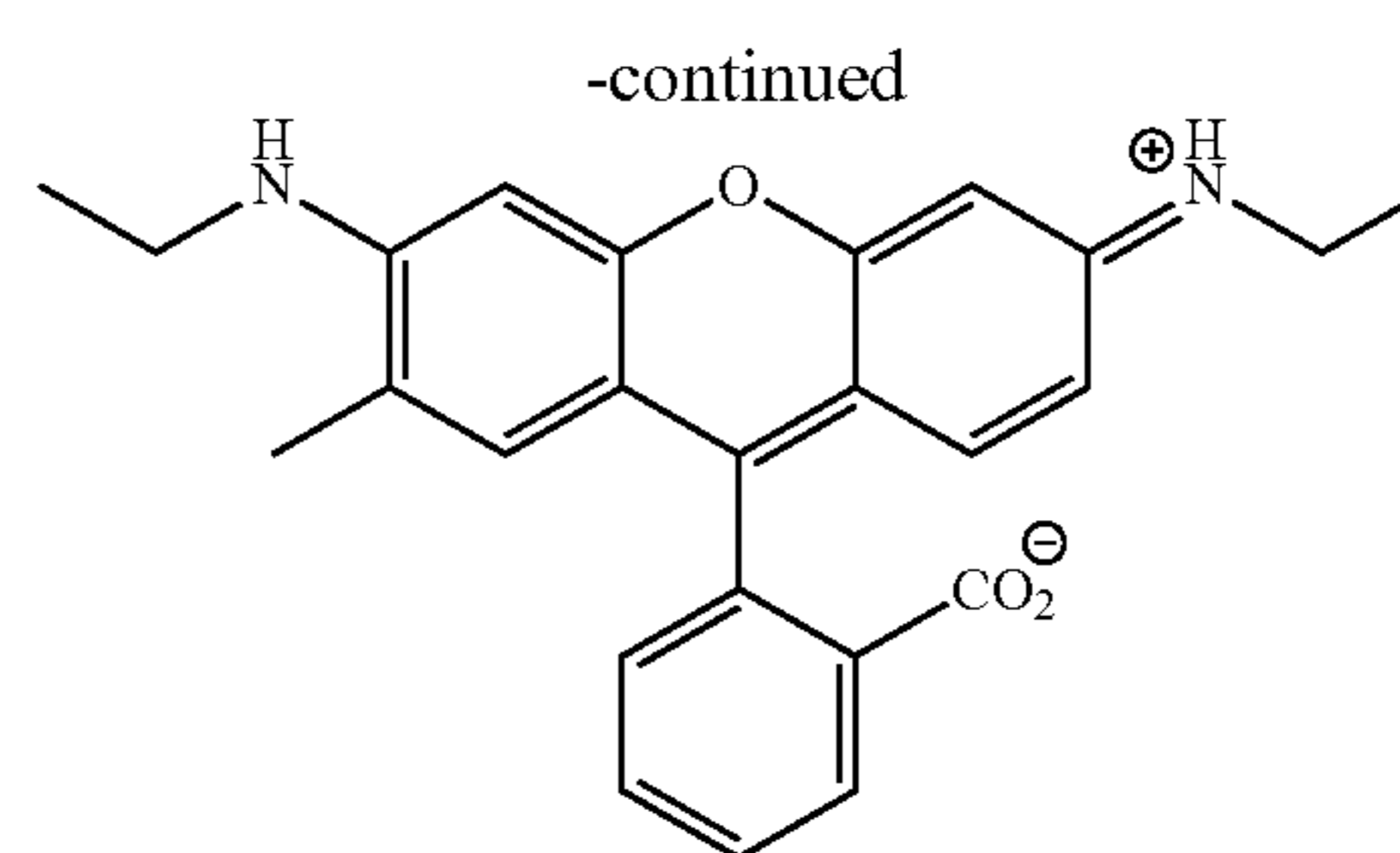
Rhodamine 575
