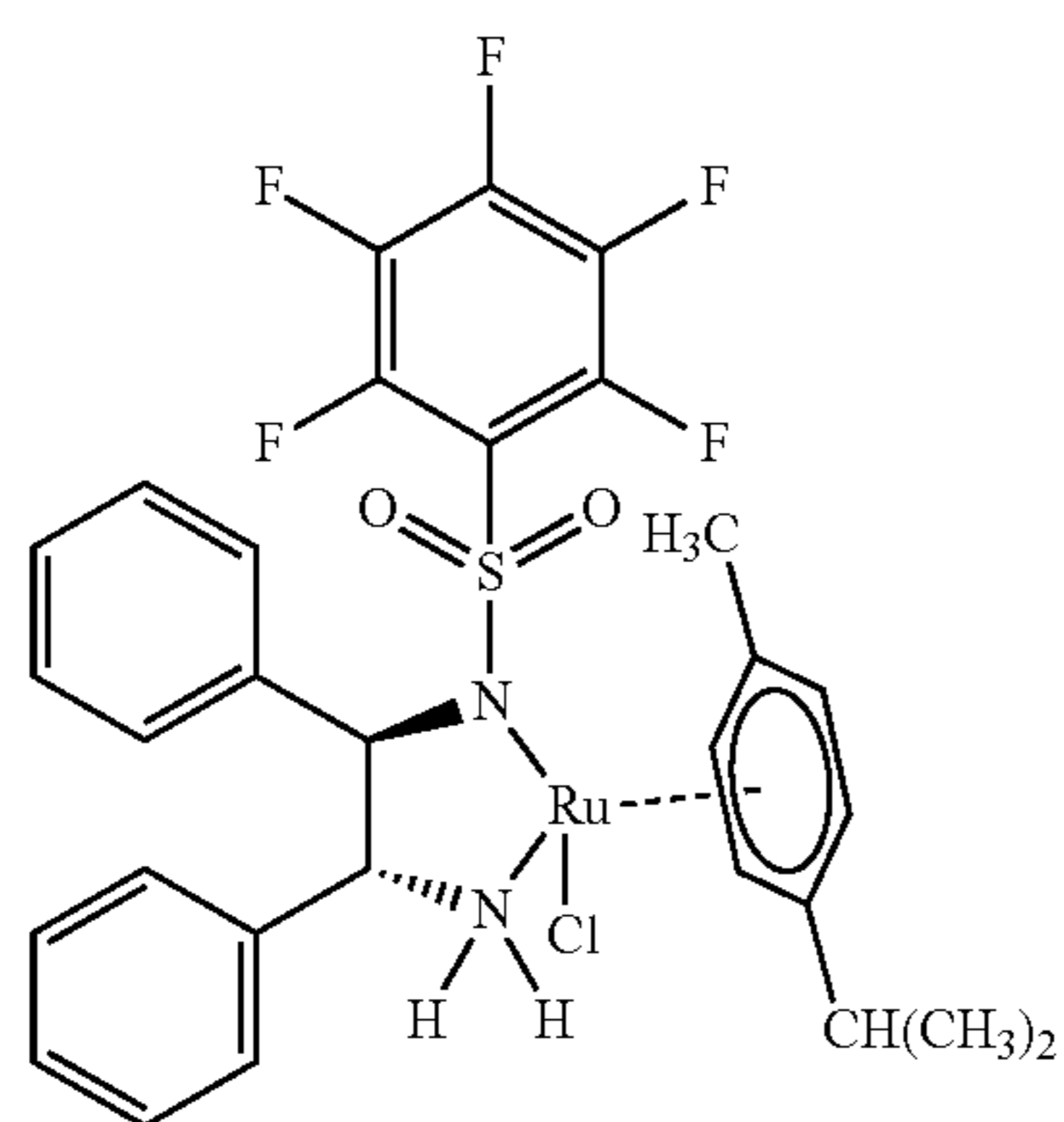
RuCl(FsDPEN)(p-cymene)
