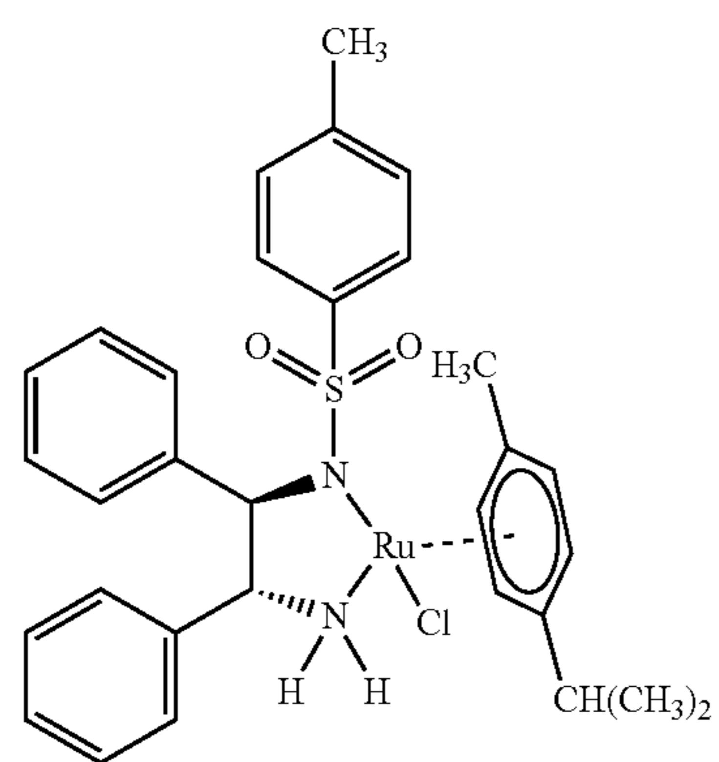
RuCl(TsDPEN)(p-cymene)
