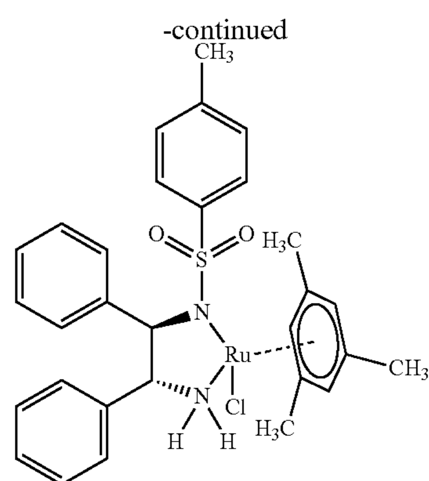
RuCl(TsDPEN)(mesitylene)
