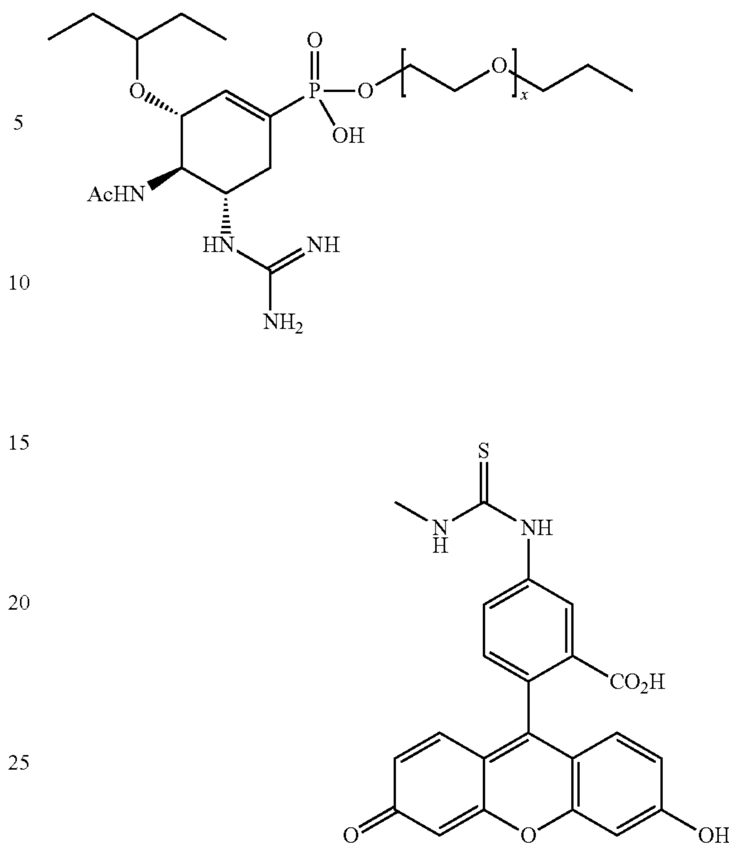
BM 8: PhosphaZanamivir-(Ethylene Glycol Linker)-Fluorescein
