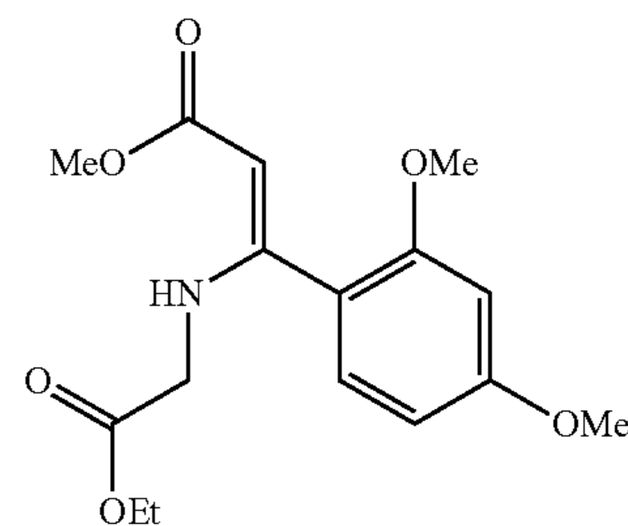
(Z)-Methyl 3-(2,4-dimethoxyphenyl)-3-((2-ethoxy-2-oxoethyl)amino)acrylate
