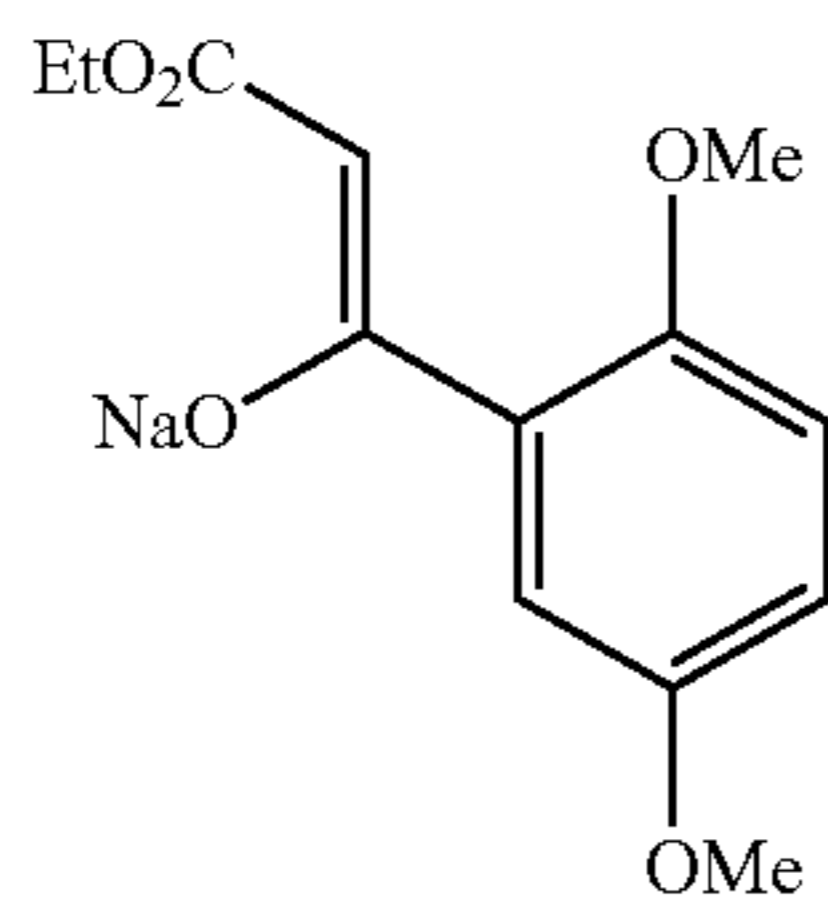
Sodium 1-(2,5-dimethoxyphenyl)-3-ethoxy-3-oxo-prop-1-en-1-olate
