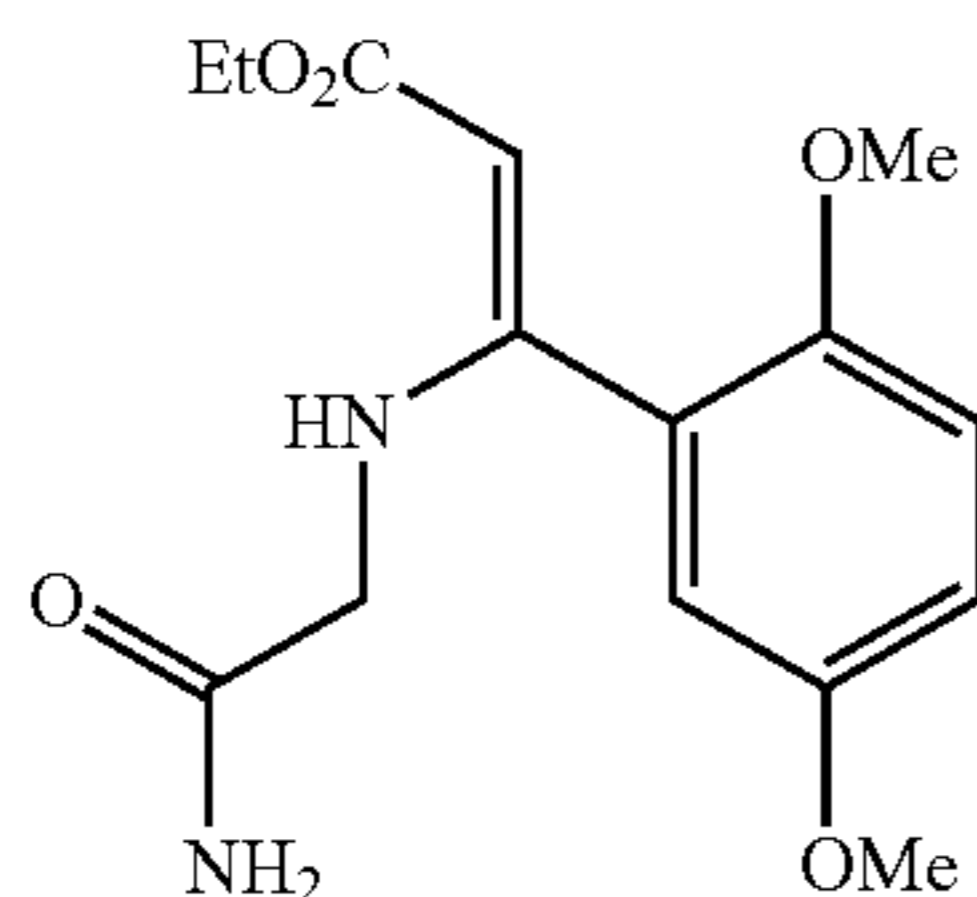
(Z)-Ethyl 3-((2-amino-2-oxoethyl)amino)-3-(2,5-dimethoxyphenyl)acrylate
