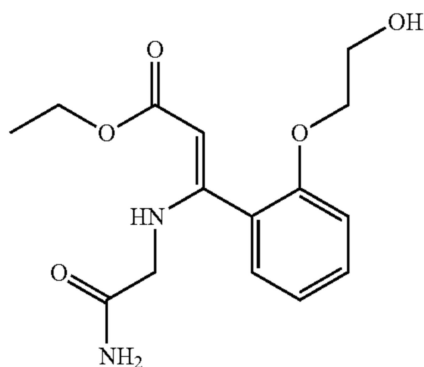
(Z)-Ethyl 3-((2-amino-2-oxoethyl)amino)-3-(2-(2-hydroxyethoxy)phenyl)acrylate
