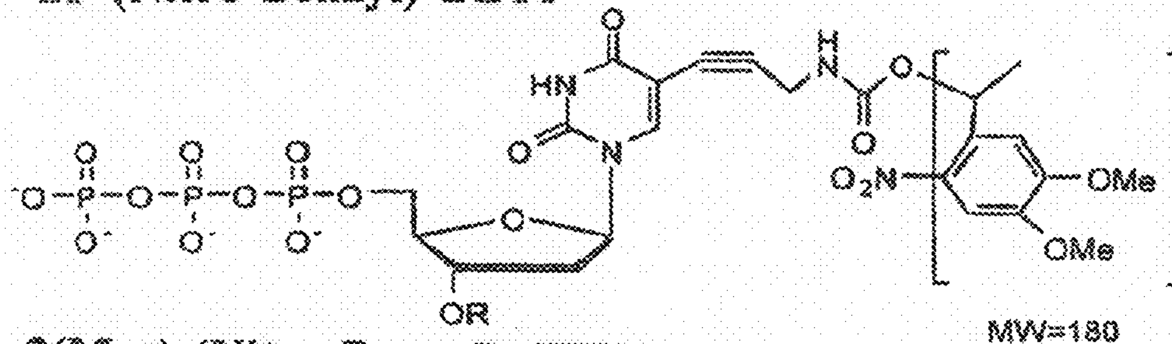
2(Meo)-(Nitro-Benzyl)-dTTP
