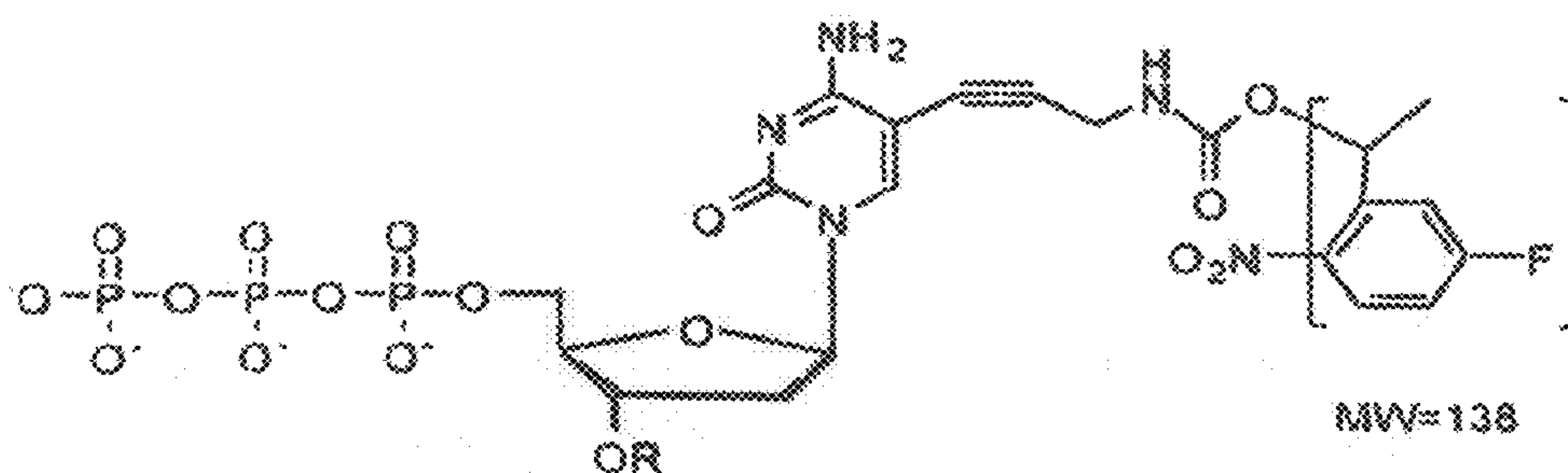
F-(Nitro-Benzyl)-dCTP
