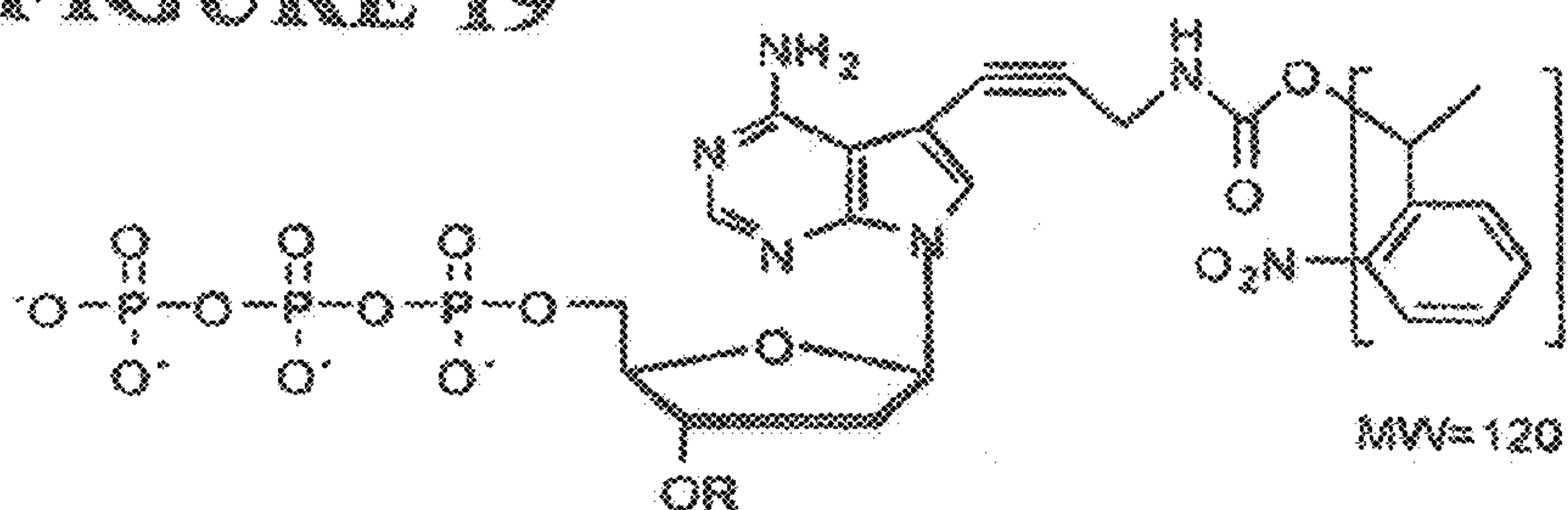
(Nitro-Benzyl)-dATP
