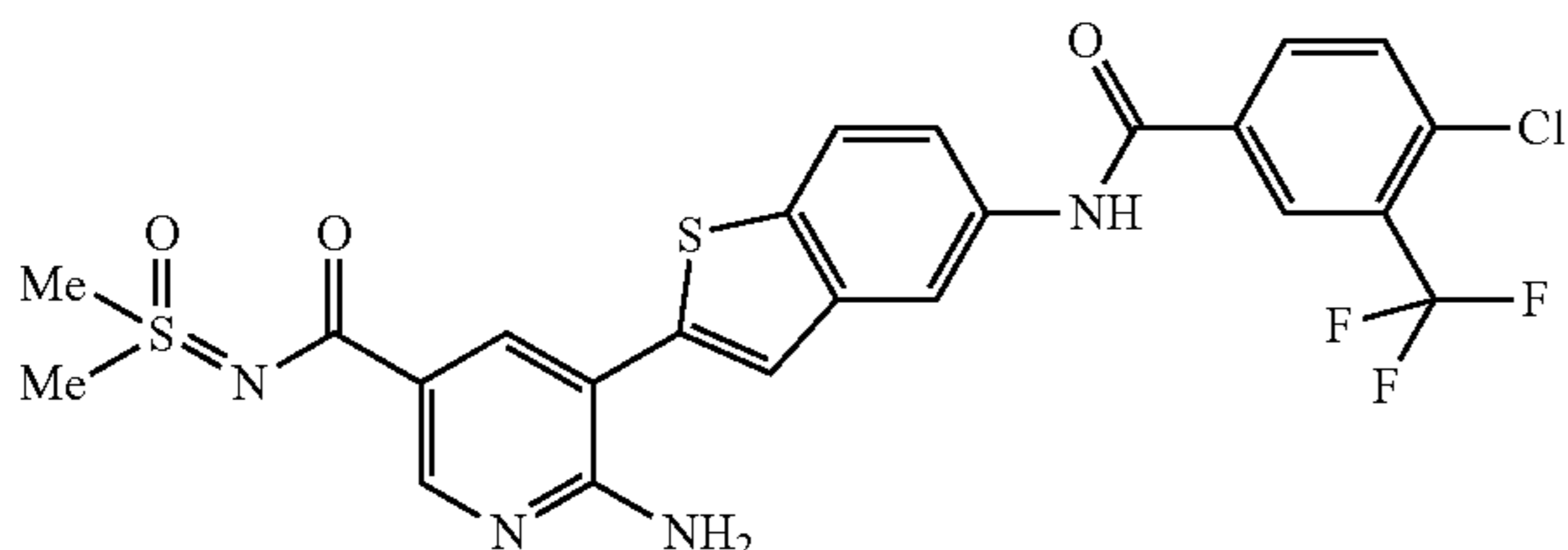
6-amino-5-(5-{[4-chloro-3-(trifluoromethyl)benzoyl]amino}-1-benzothien-2-yl)-N-[dimethyl(oxido)-λ 4 -sulfanylidene]nicotinamide
