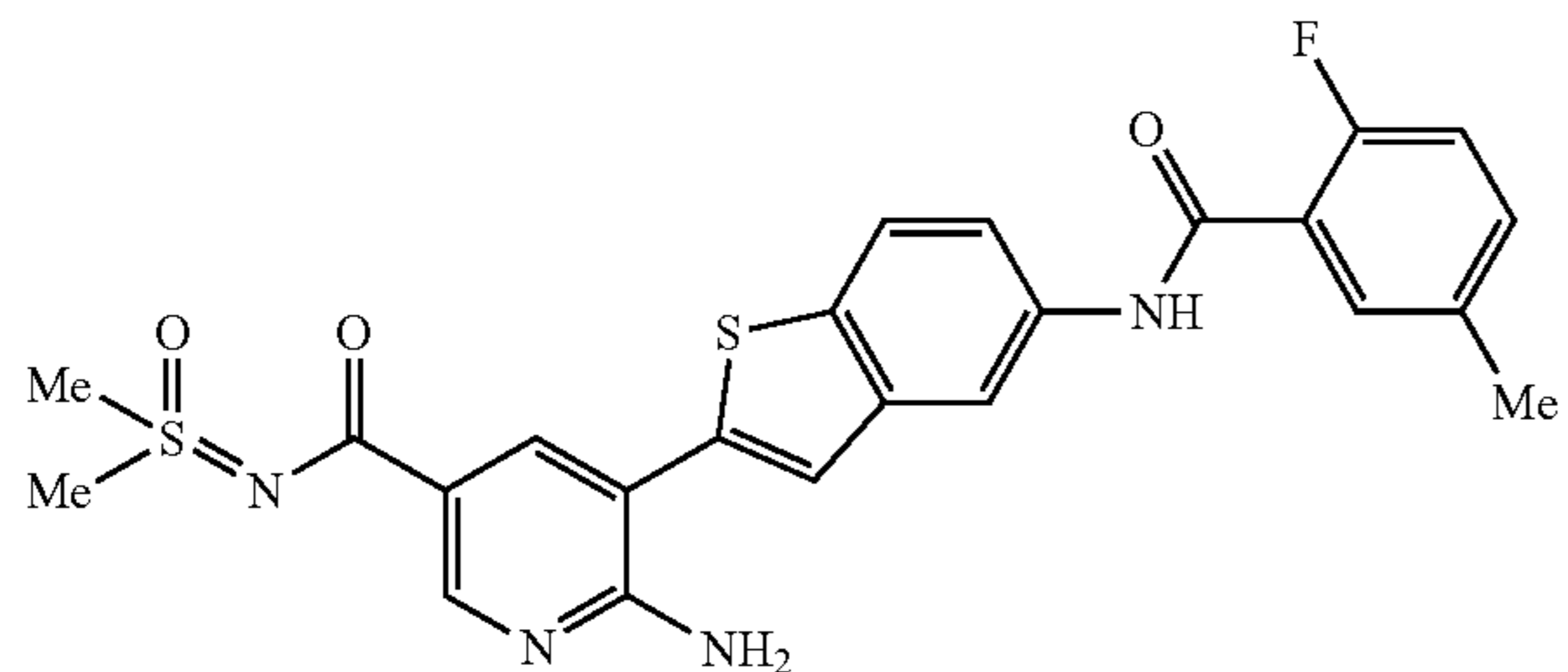
6-amino-N-[dimethyl(oxido)-λ 4 -sulfanylidene]-5-{5-[(2-fluoro-5-methylbenzoyl)amino]-1-benzothien-2-yl}nicotinamide
