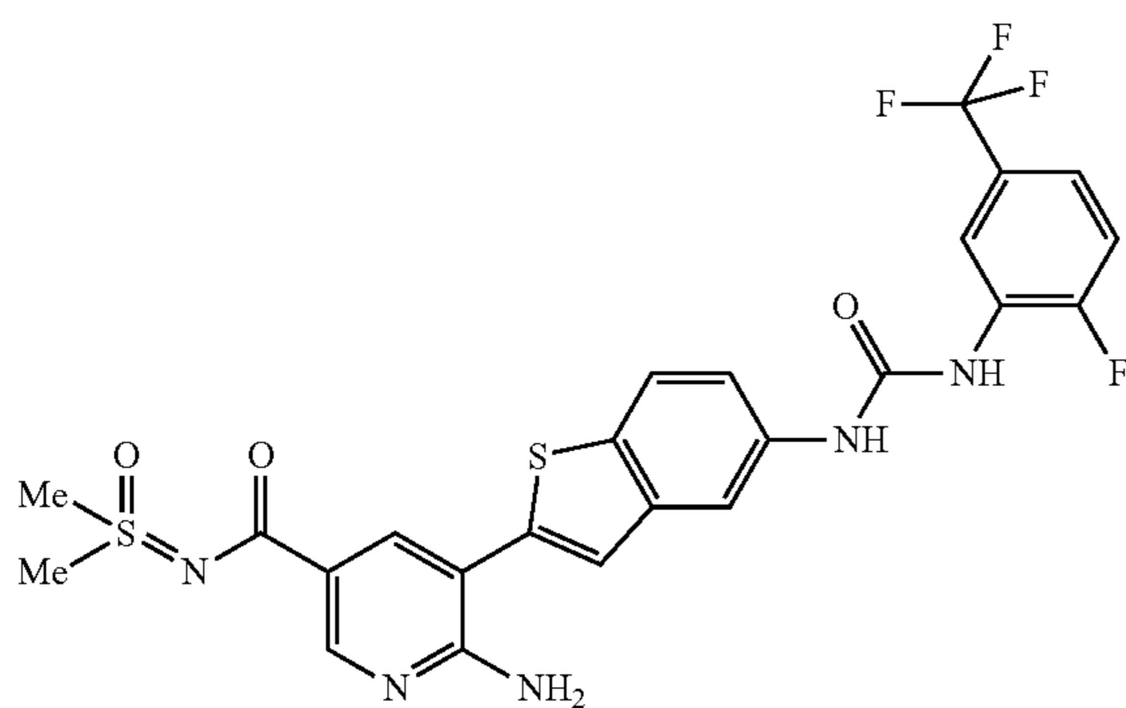
6-amino-N-[dimethyl(oxido)-λ 4 -sulfanylidene]-5-{5-[[[2-fluoro-5-(trifluoromethyl)phenyl]amino]carbonyl]amino]-1-benzothien-2-yl}nicotinamide
