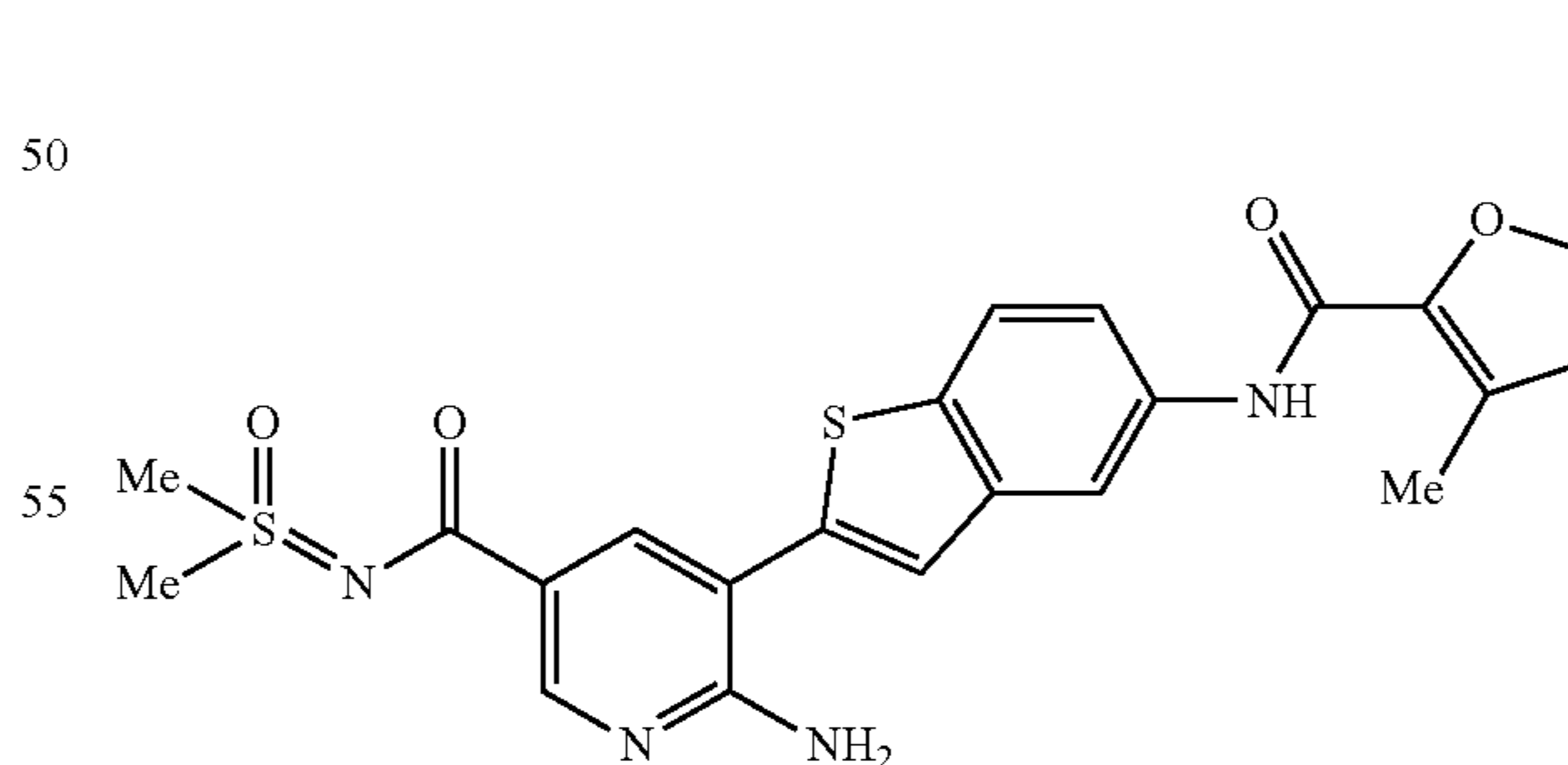
6-amino-N-[dimethyl(oxido)-λ 4 -sulfanylidene]-5-{5-[(3-methyl-2-furoyl)amino]-1-benzothien-2-yl}nicotinamide
