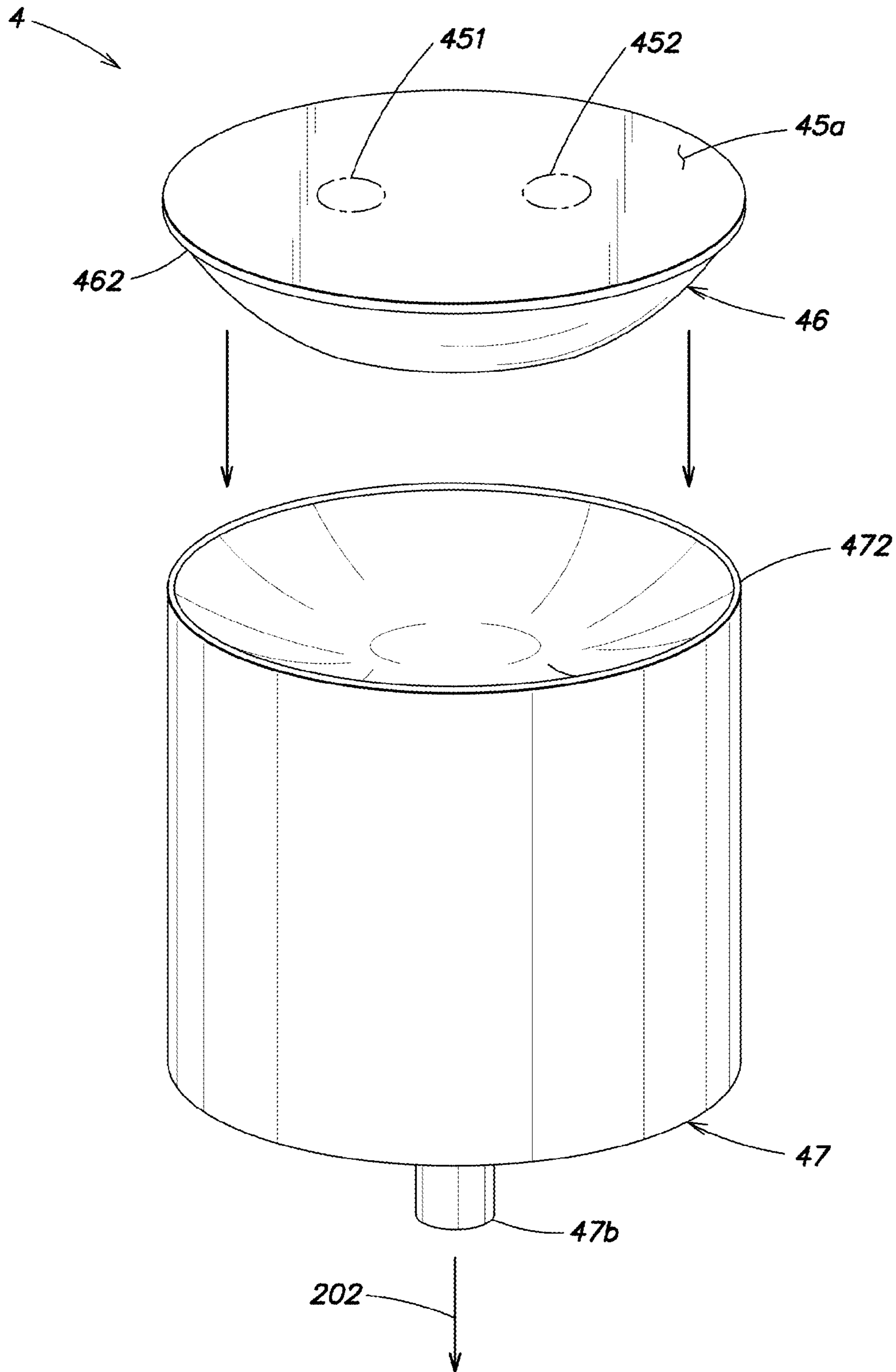
FIG. 64
