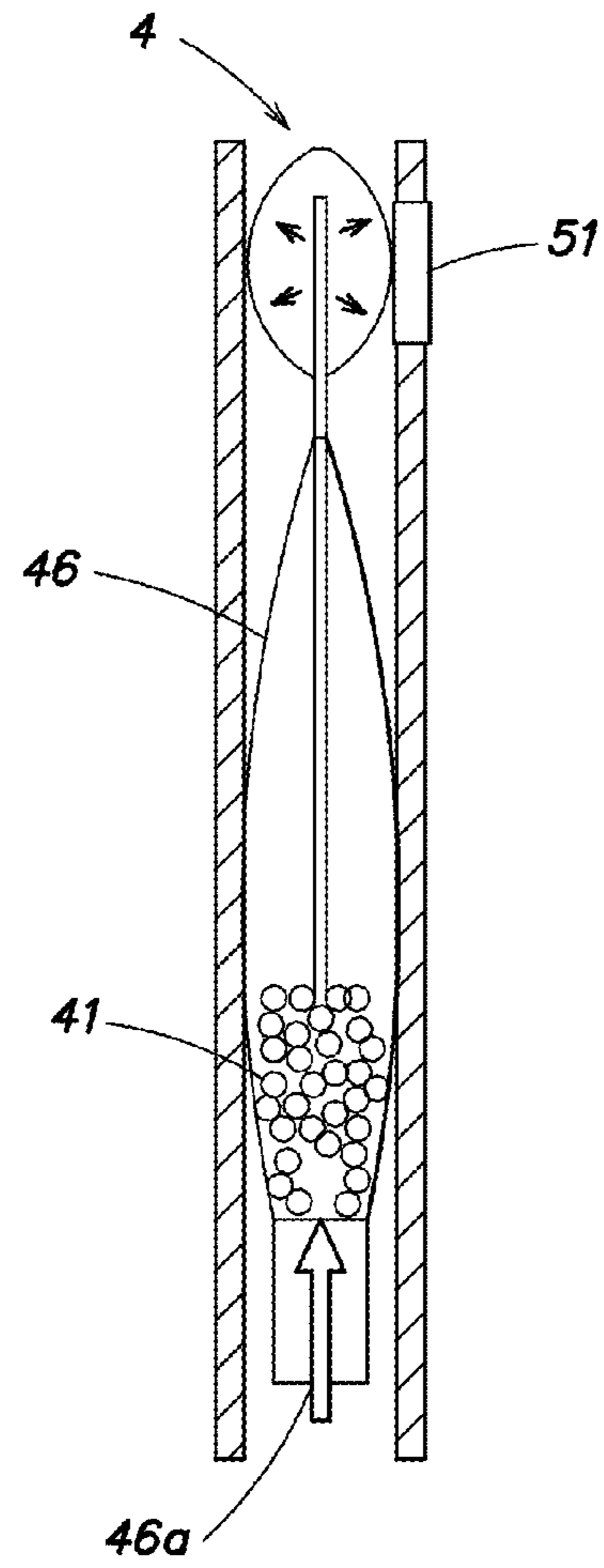
FIG. 44
