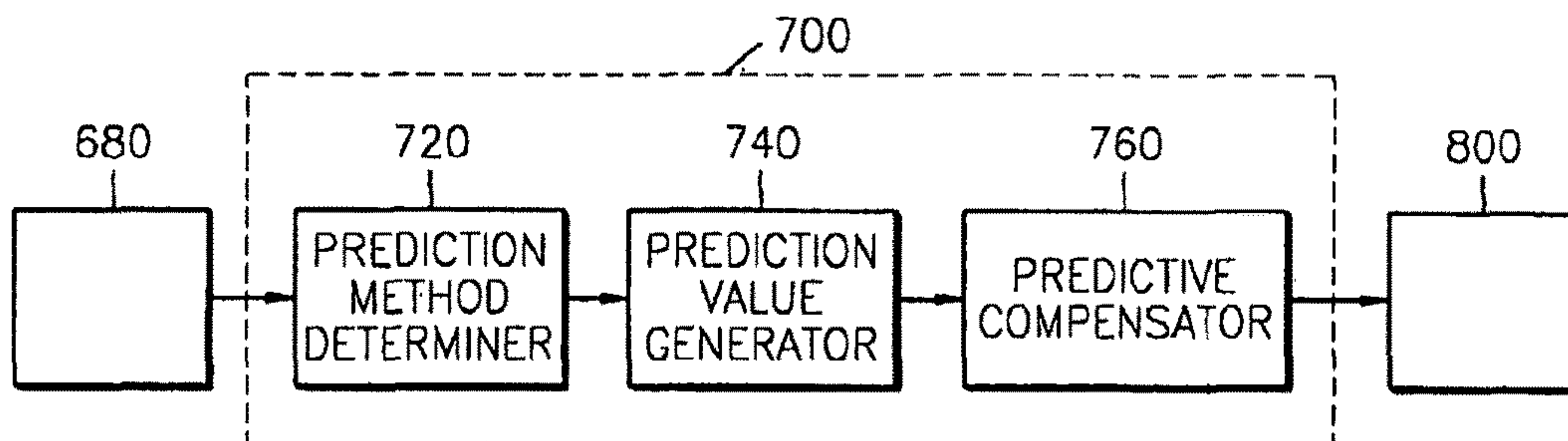
FIG. 7B
