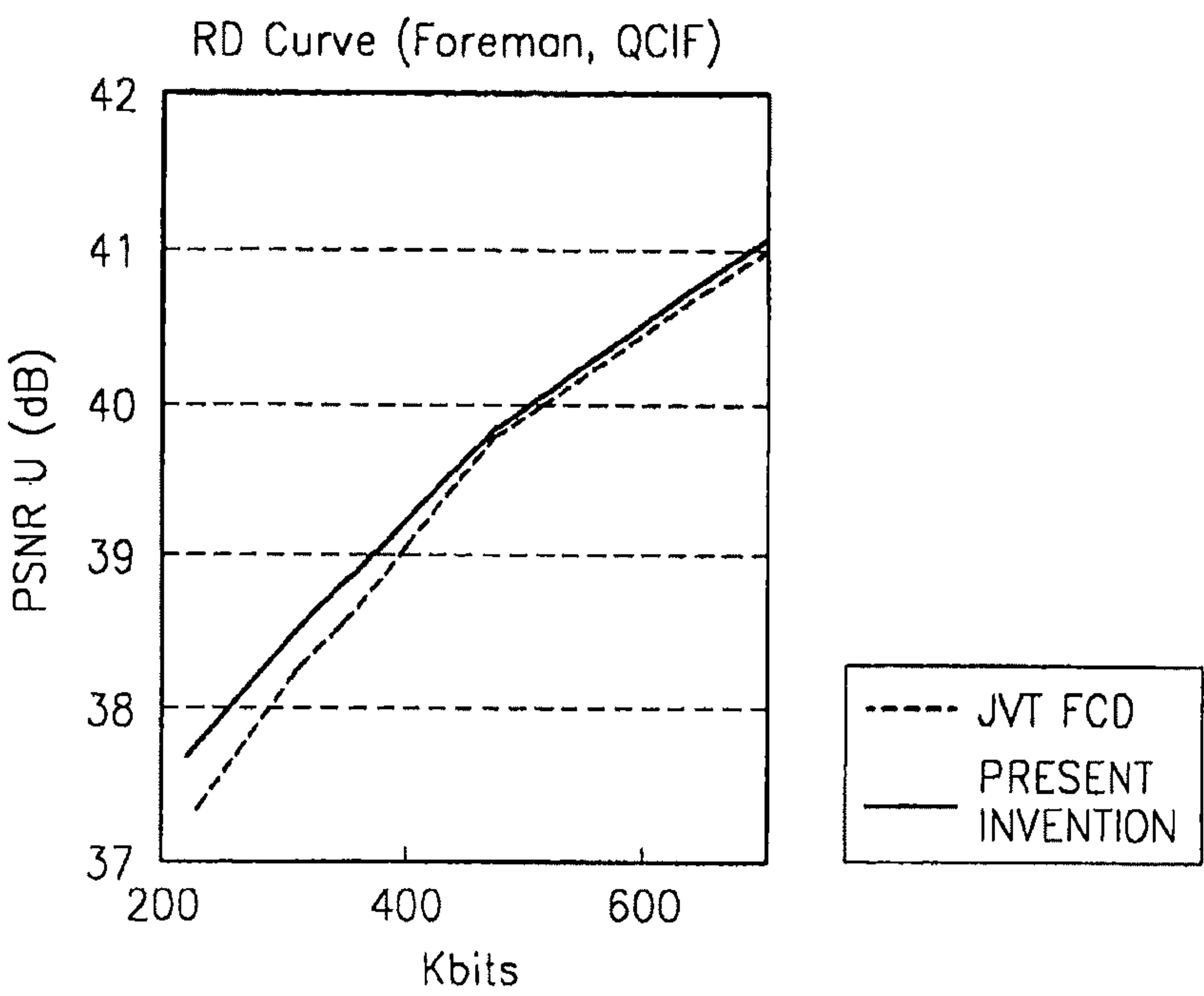
FIG. 8A
