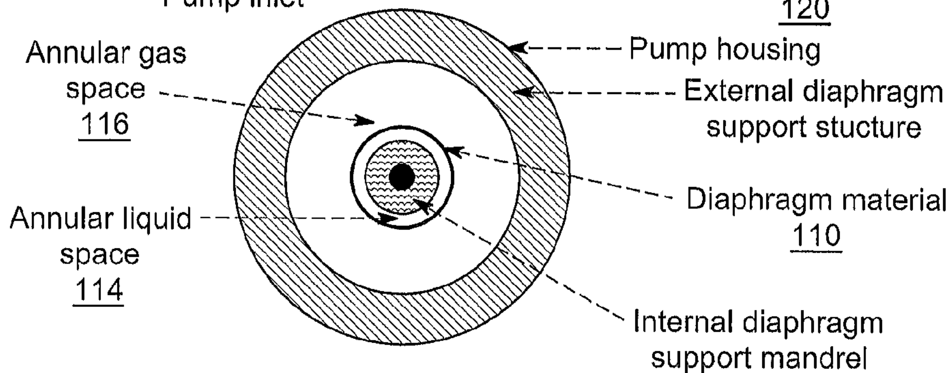
FIG. 21B
