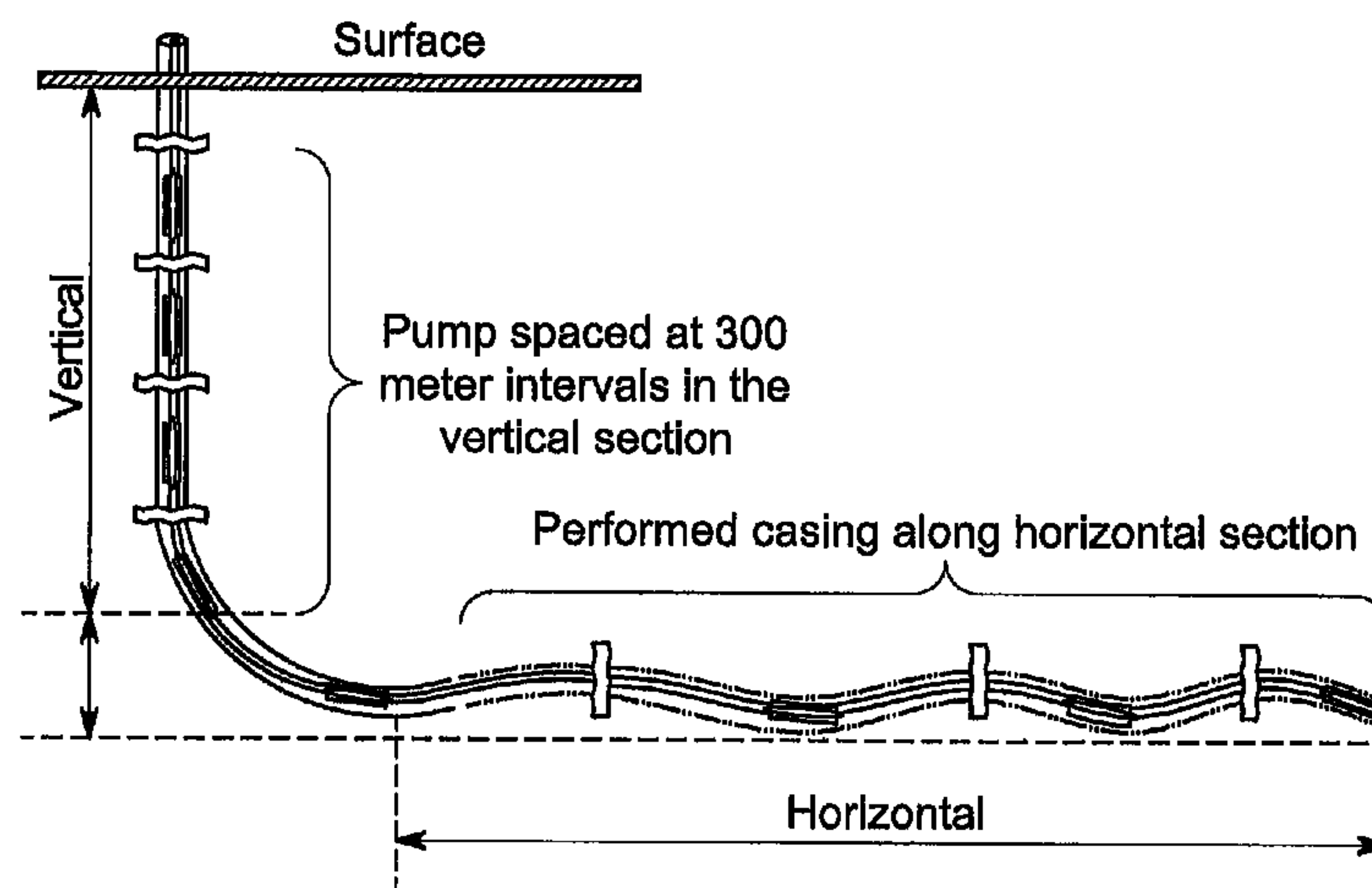
FIG. 29
