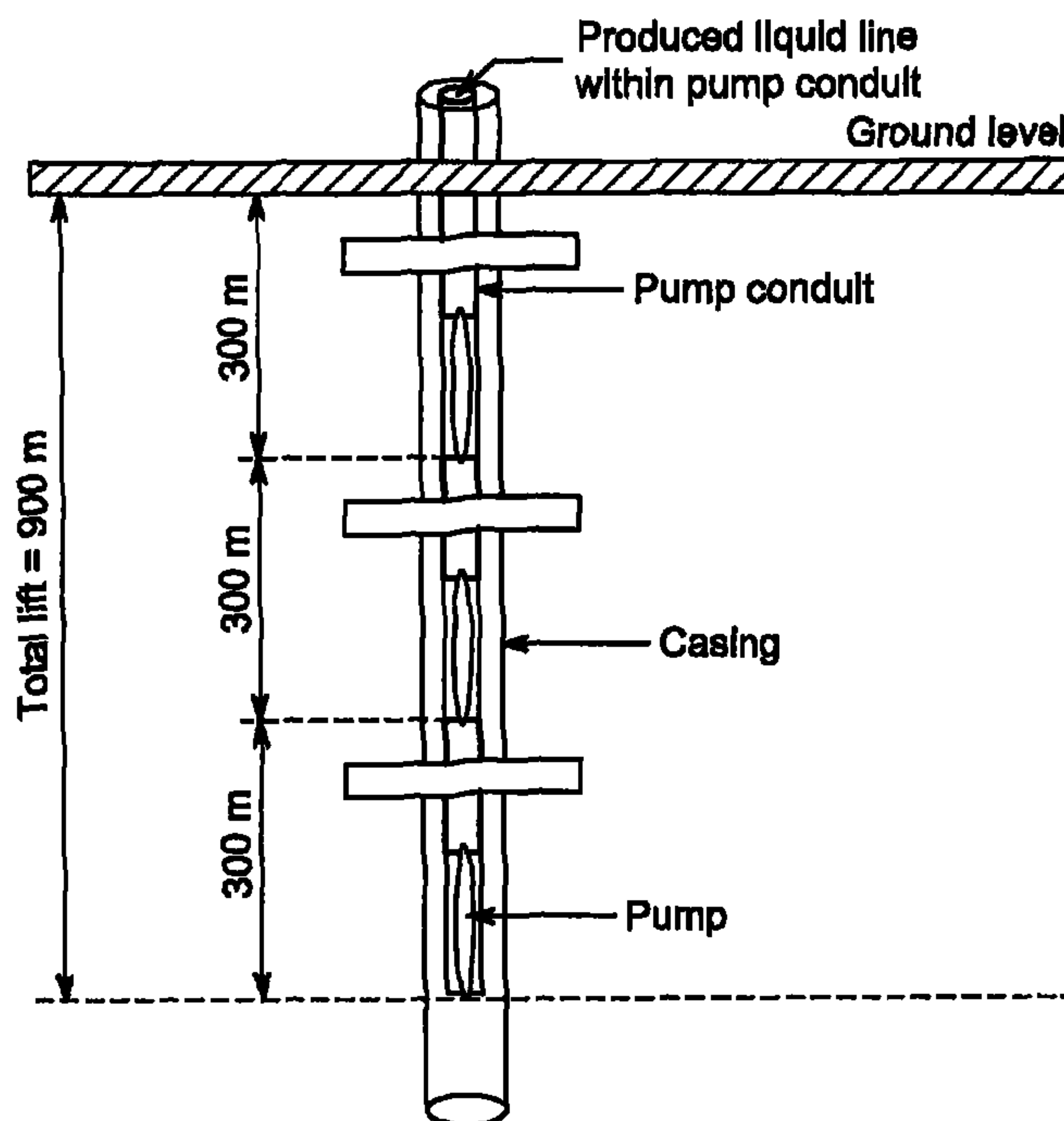
FIG. 24
