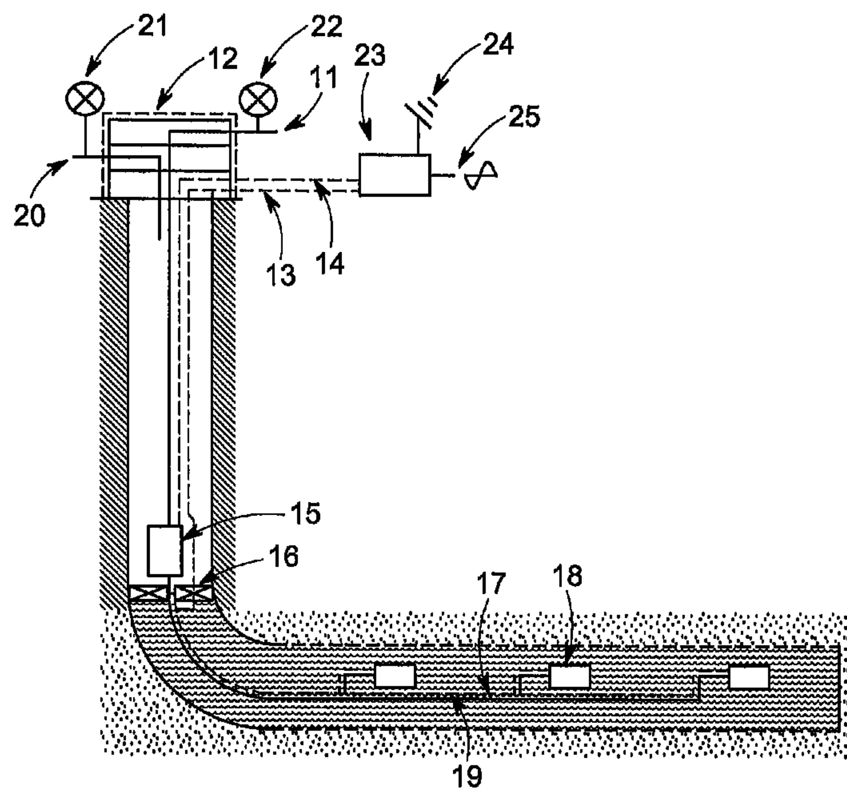
FIG. 13
