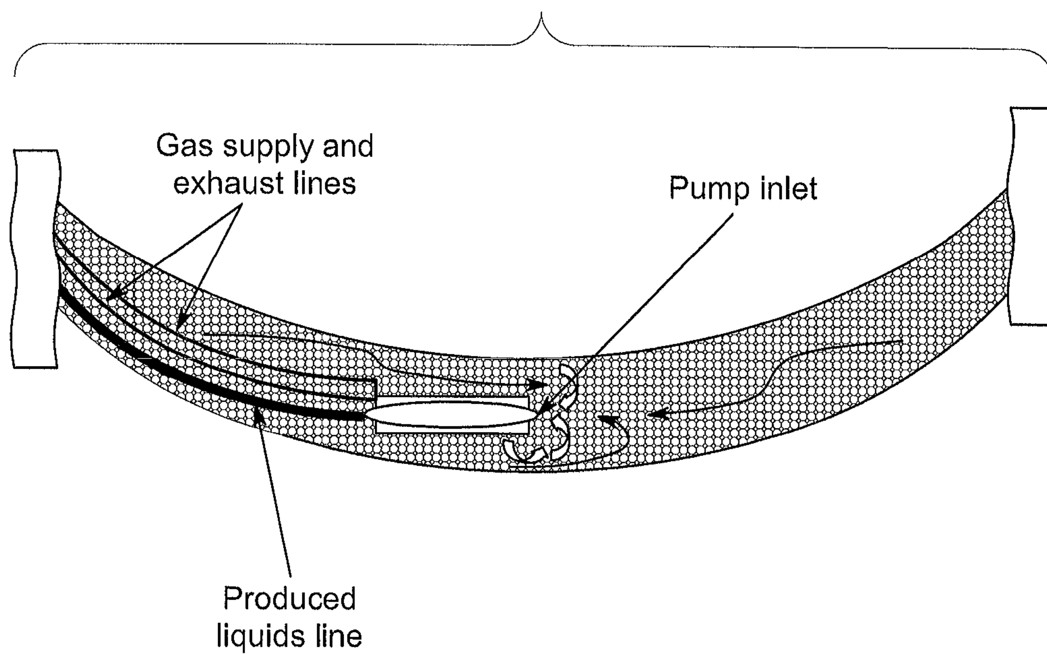
FIG. 27
