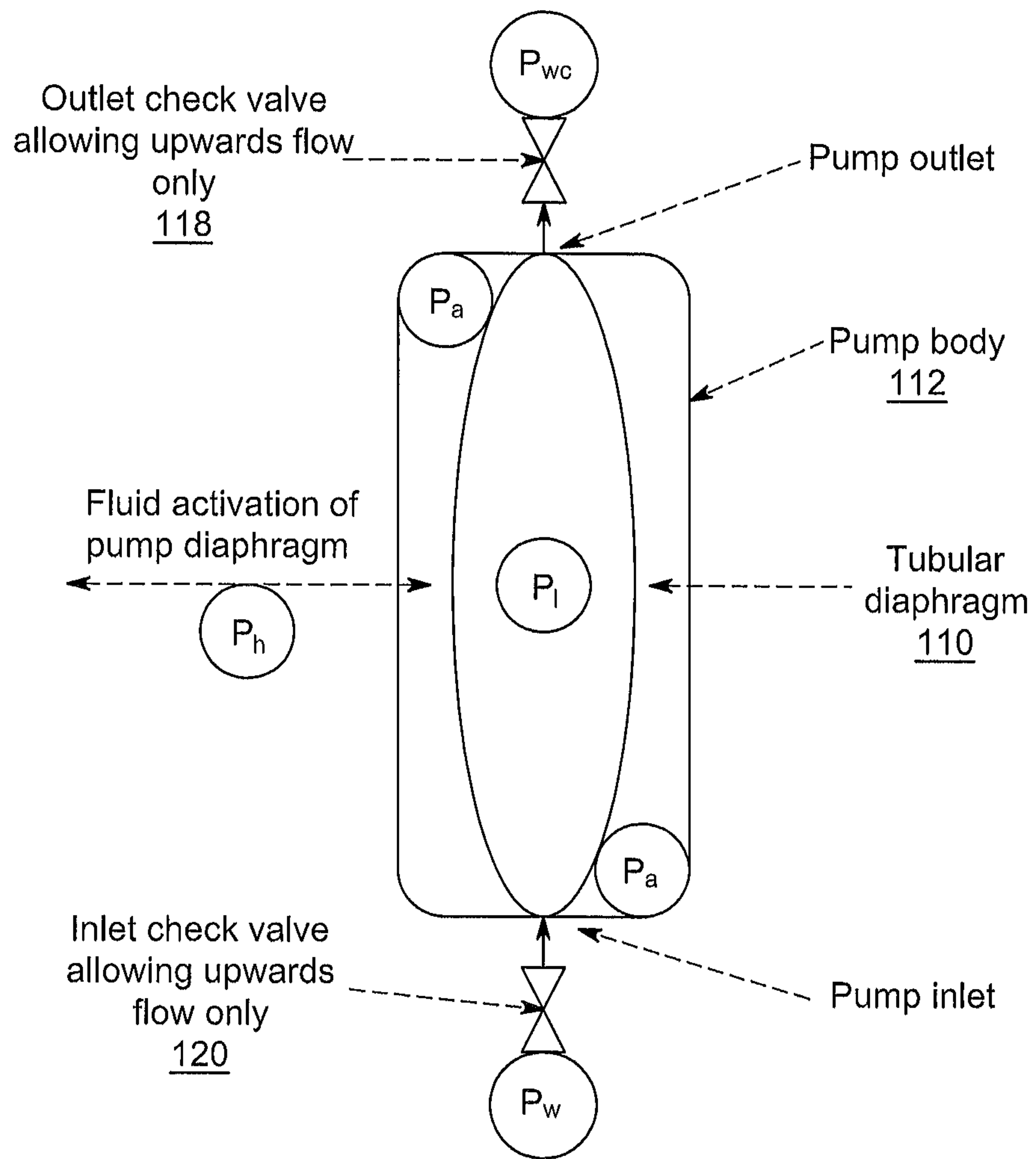
FIG. 18
