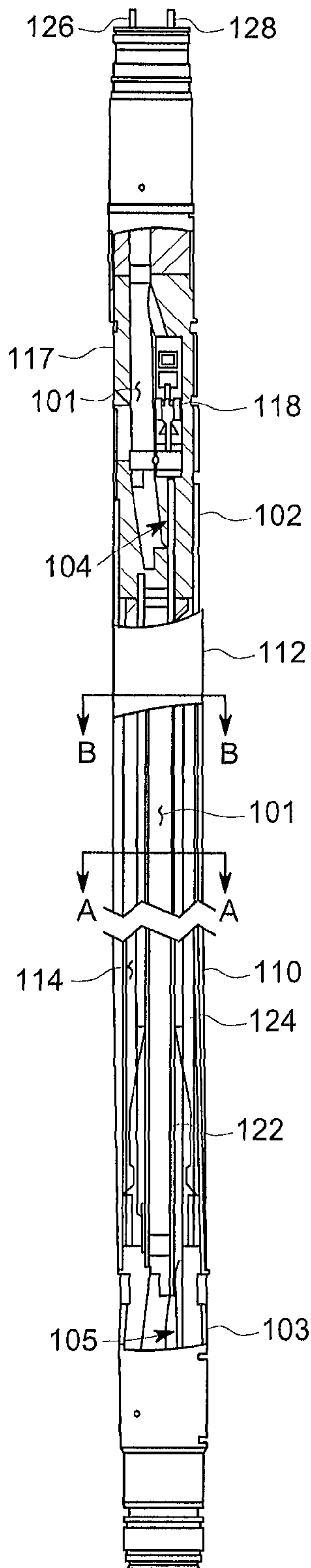
FIG. 22A
