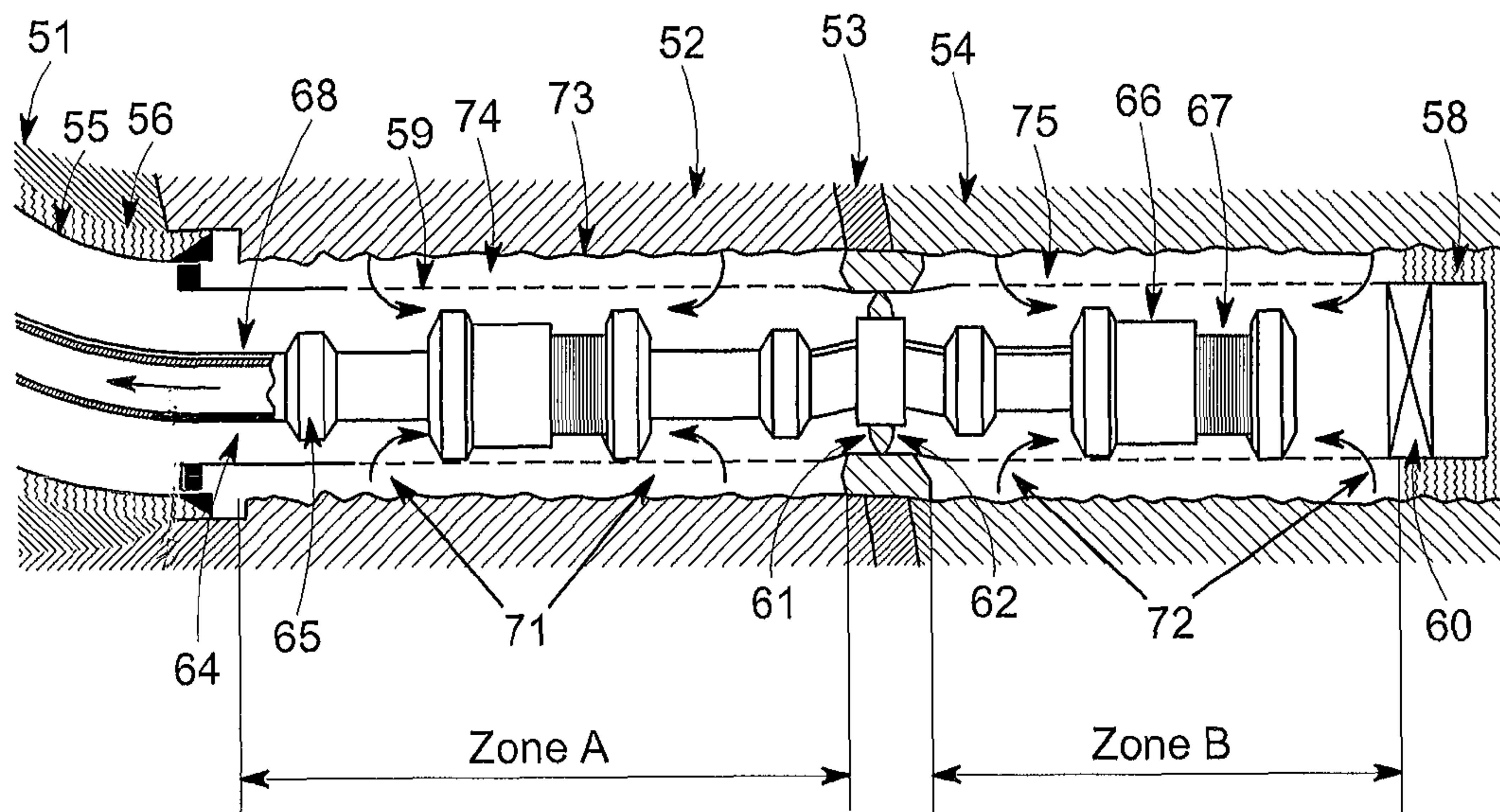
FIG. 15
