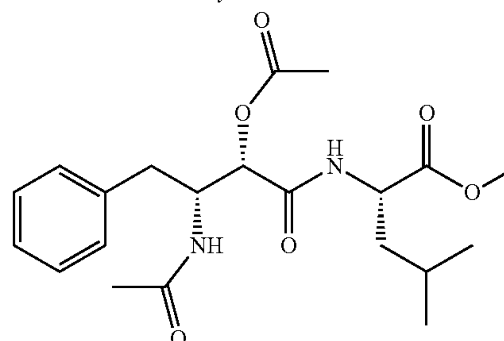
di-acyl ubenimex
