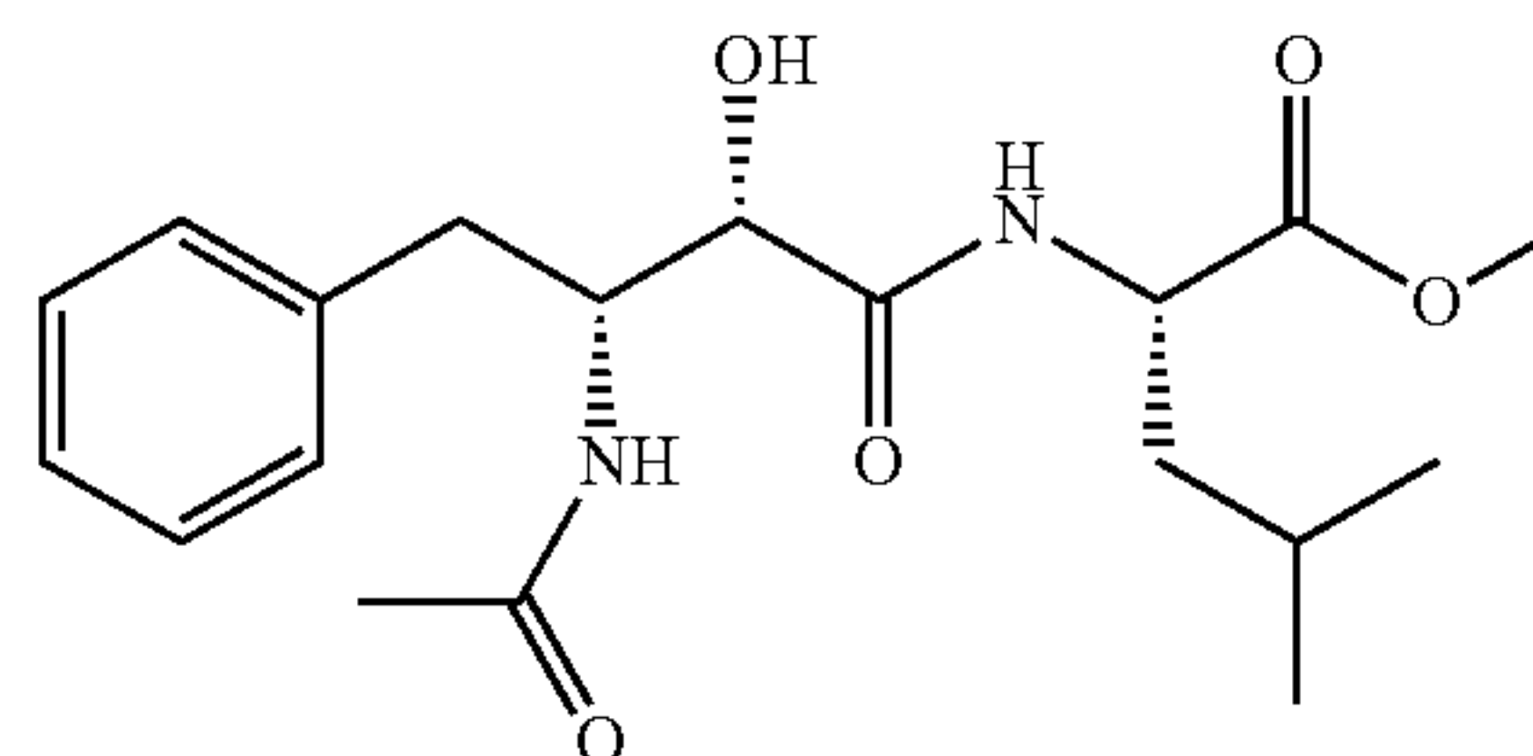
mono-acyl ubenimex
