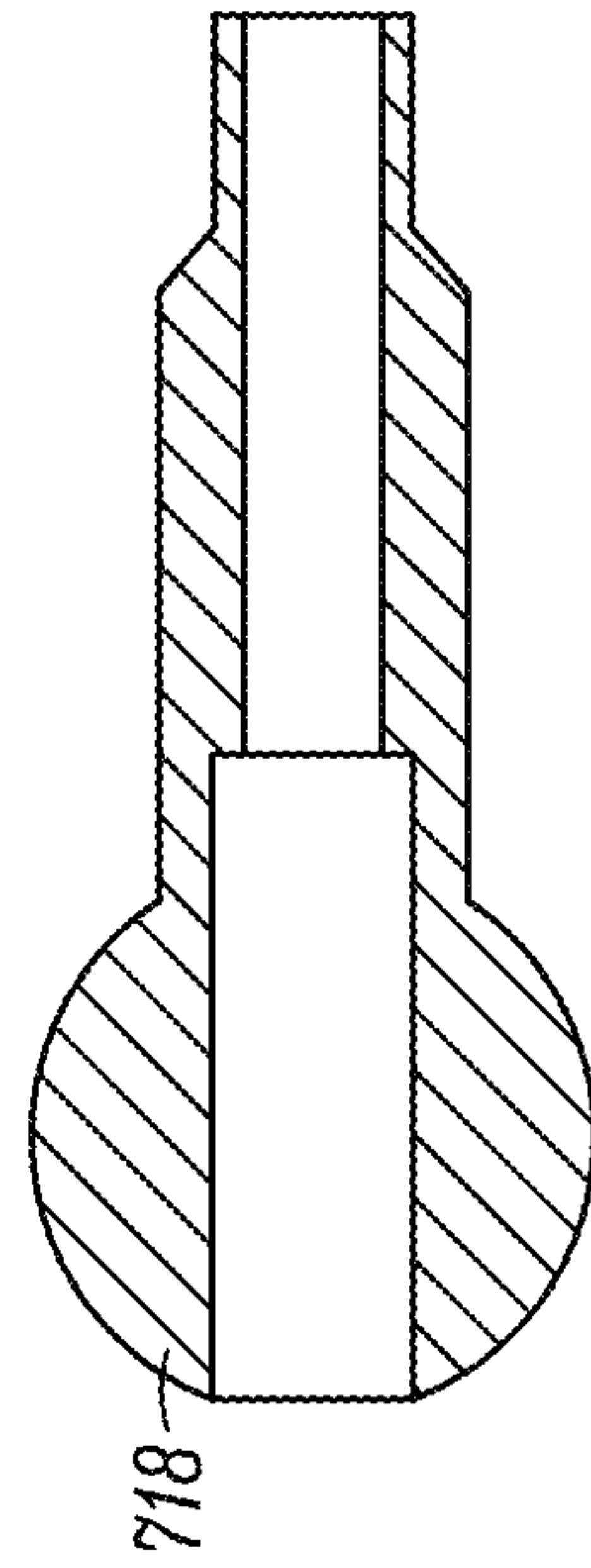
SECTION A-A FIG. 8E
