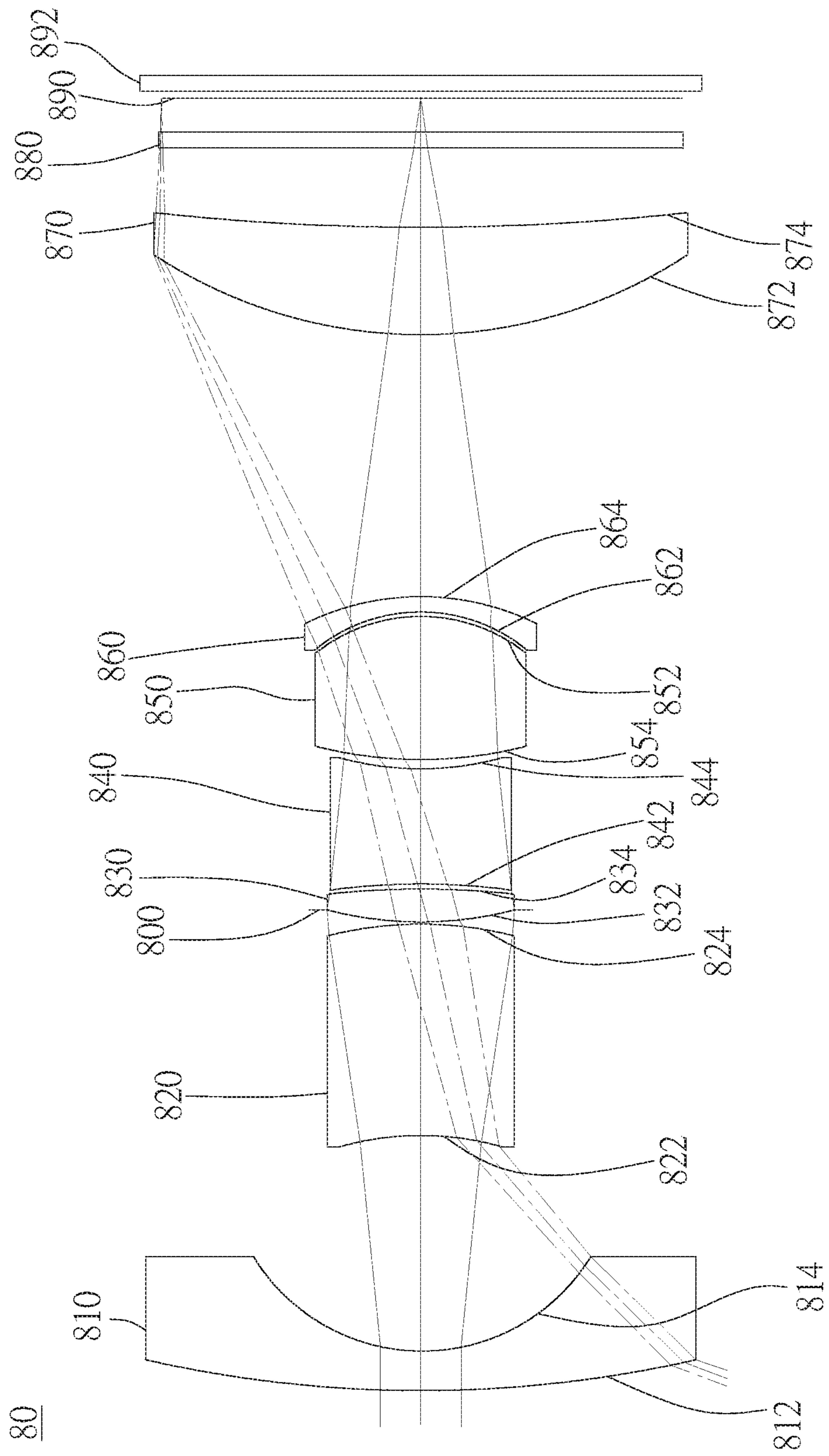
FIG. 8 A
