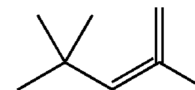
2,4,4-trimethylpent-2-ene ( \beta -DIB)
