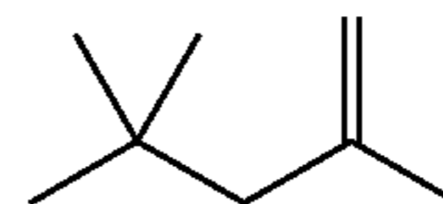
2,4,4-trimethylpent-1-ene ( \alpha -DIB)
