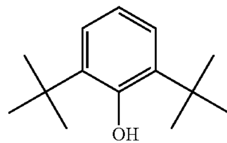
2,6-di-tert-butylphenol
