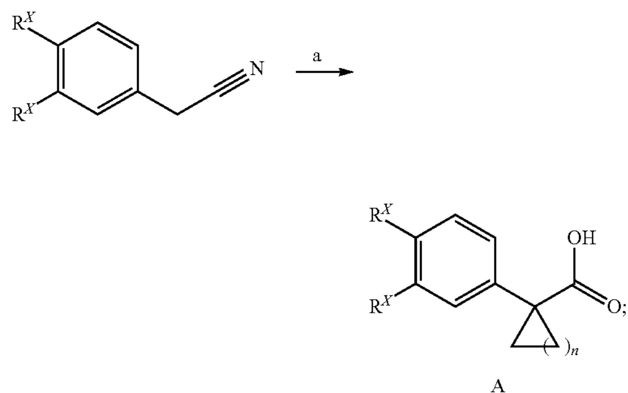
Scheme I-A:
