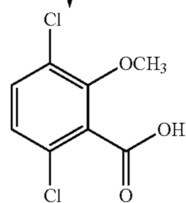
Dicamba
