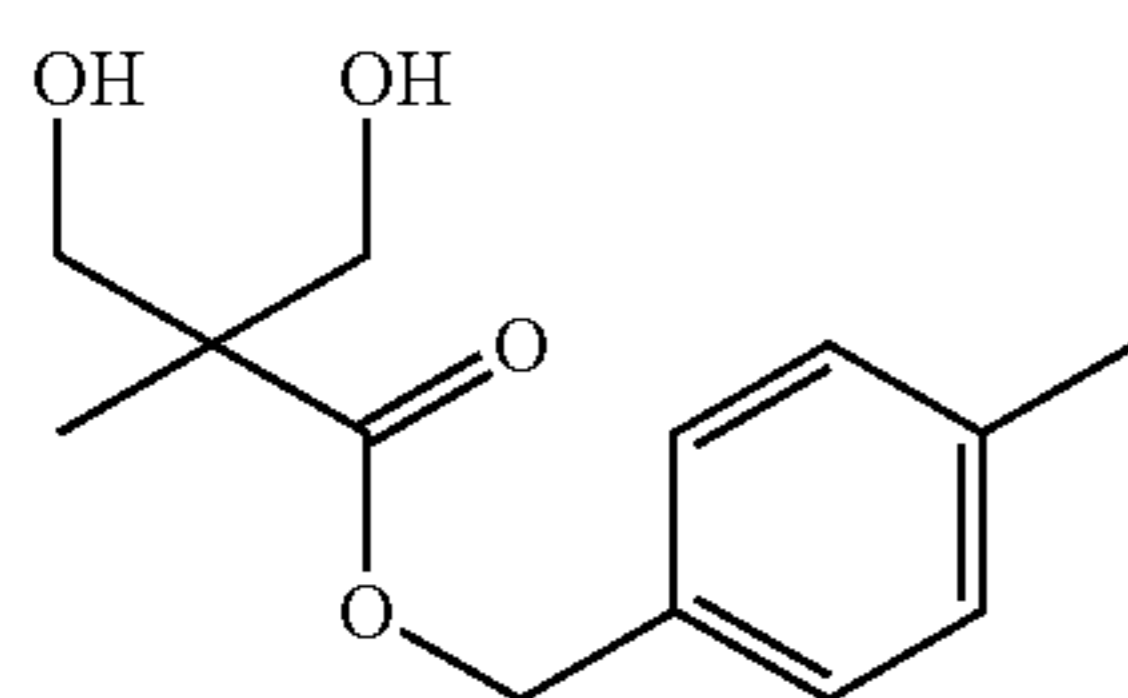
MPA-OCH2Tol MW 238.2
