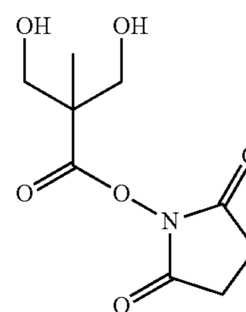
MPA-NHS
