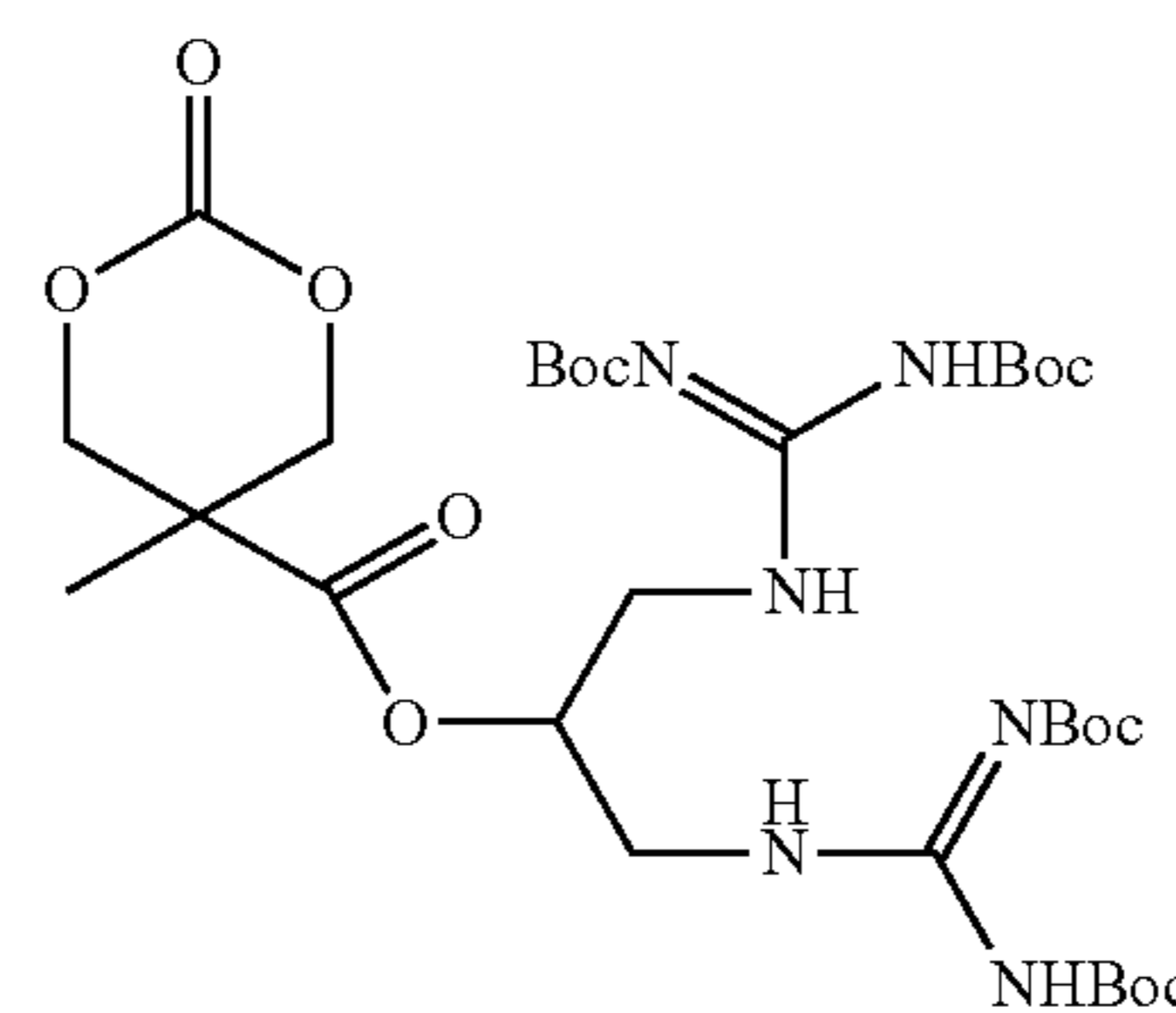
MTC-iPrG1
