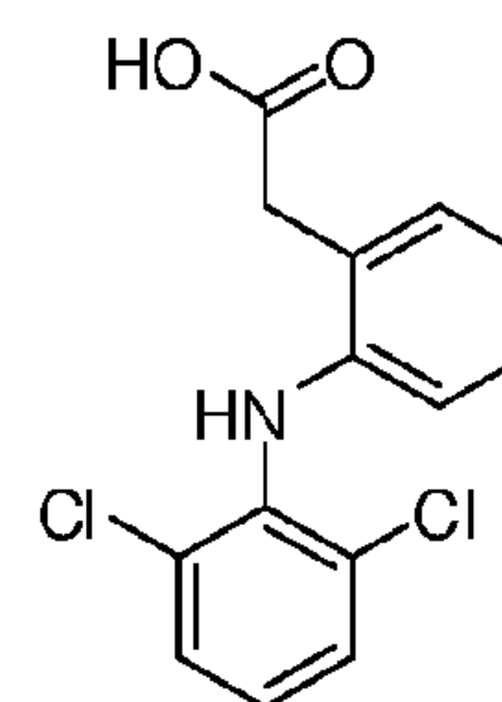
Diclofenac
