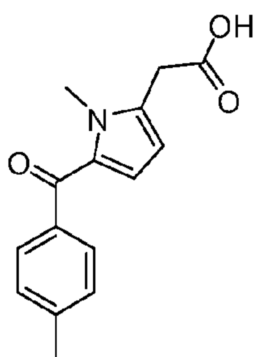
Tolmetin
