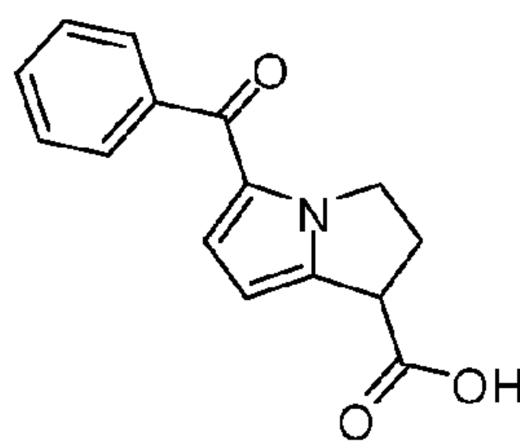
Ketorolac
