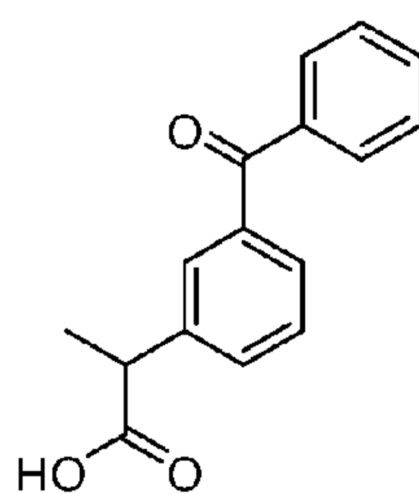
Ketoprofen
