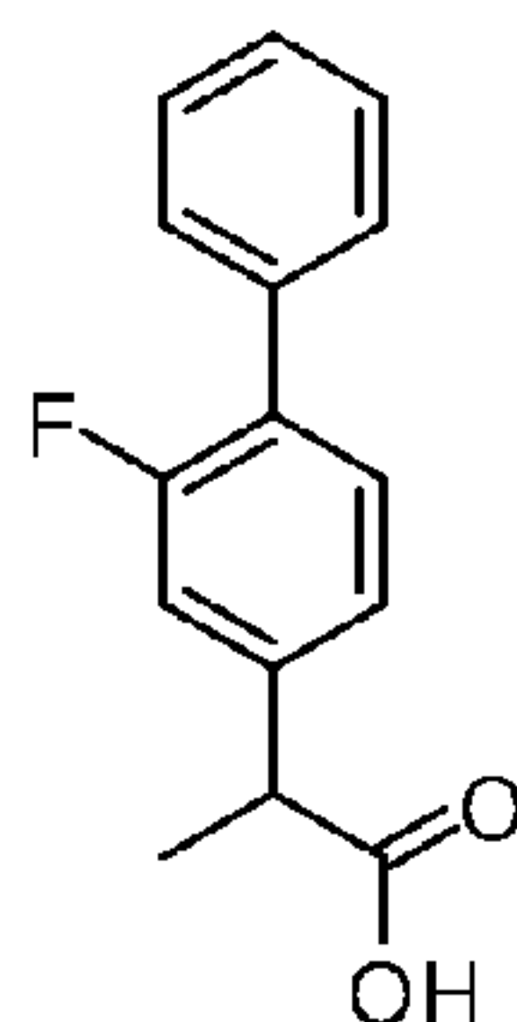
Flurbiprofen
