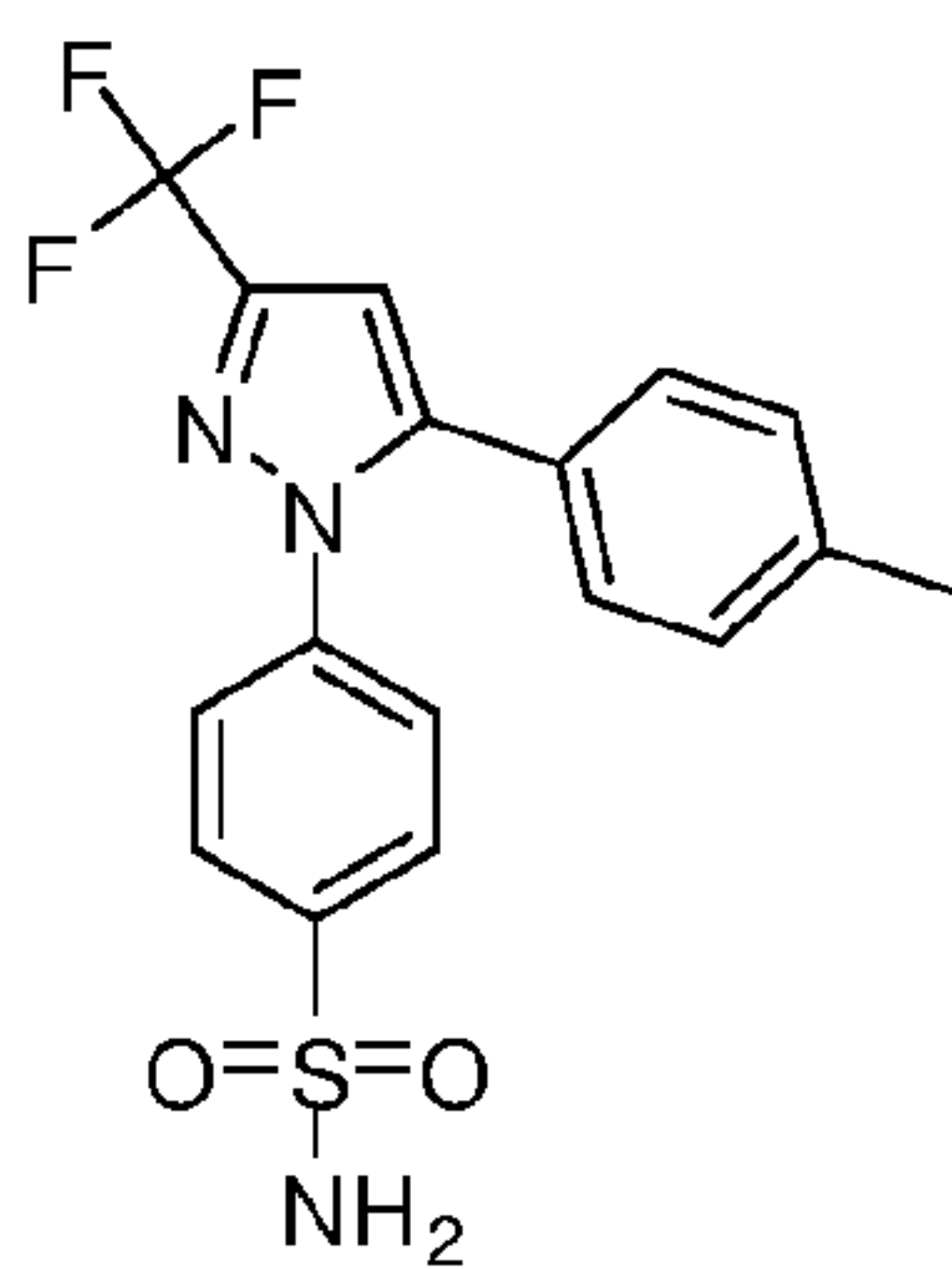
Celecoxib
