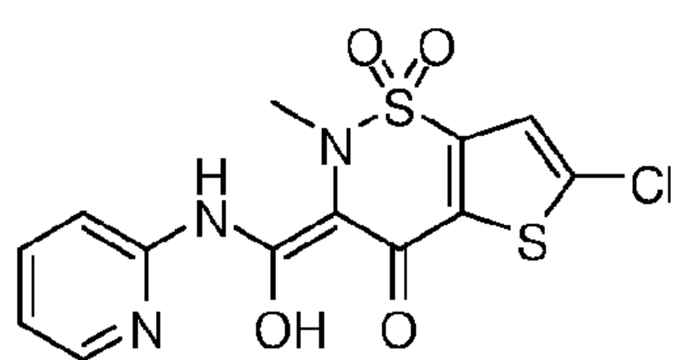
Lornoxicam
