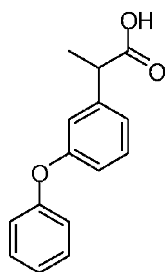
Fenopropfen
