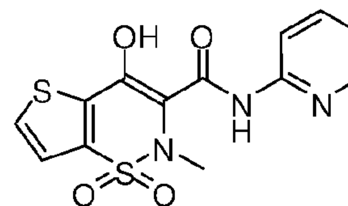
Tenoxicam
