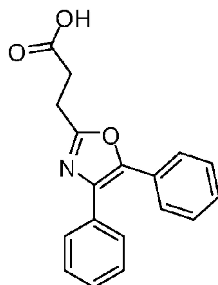
Oxaprozin
