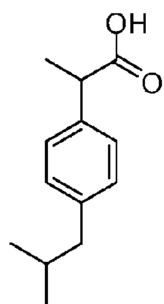
Ibuprofen
