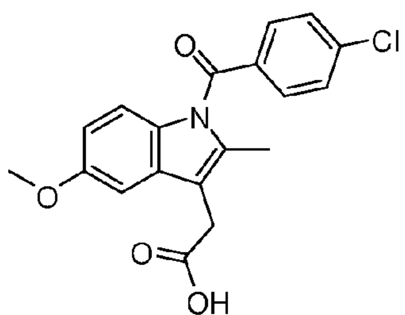
Indomethacin
