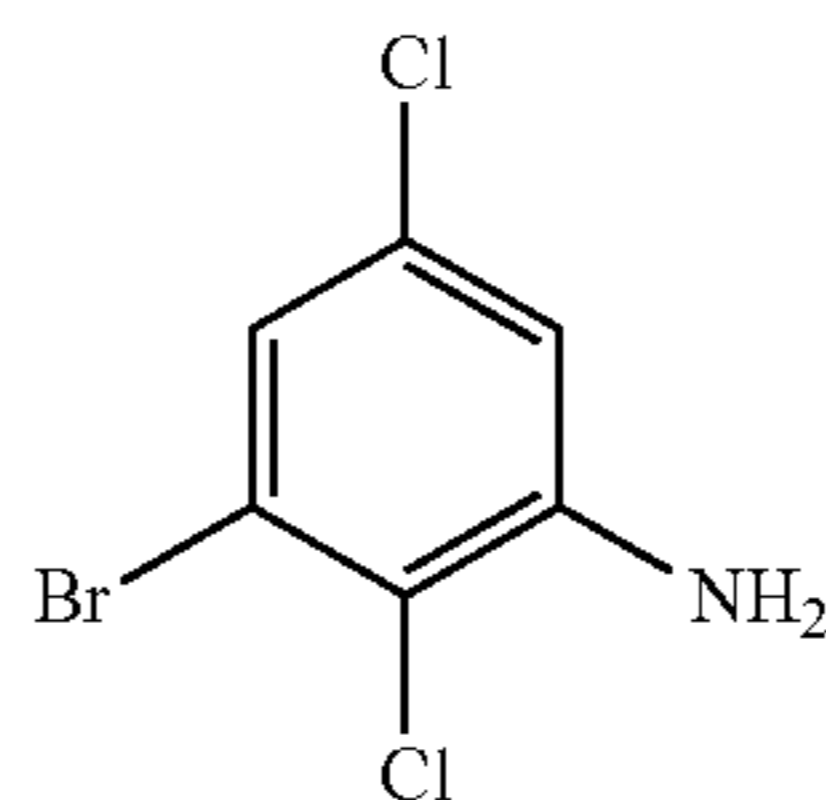
3-bromo-2,5-dichloroaniline
