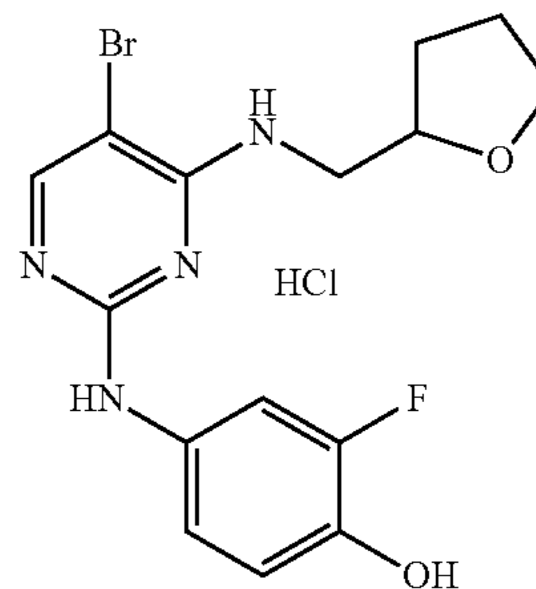
4-(5-bromo-4-((tetrahydrofuran-2-yl)methyl)amino)pyrimidin-2-ylamino)-2-fluorophenol (SK1-044)
