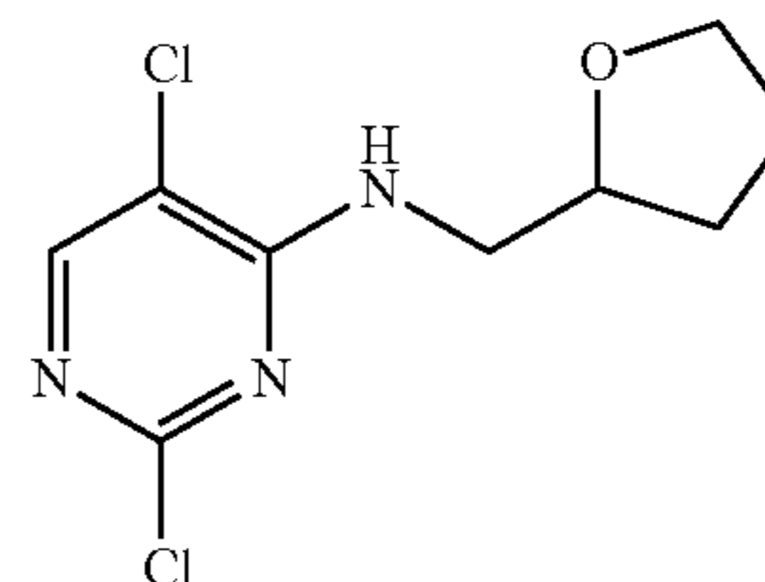
2,5-Dichloro-N-((tetrahydrofuran-2-yl)methyl)pyrimidin-4-amine (NT1-003)
