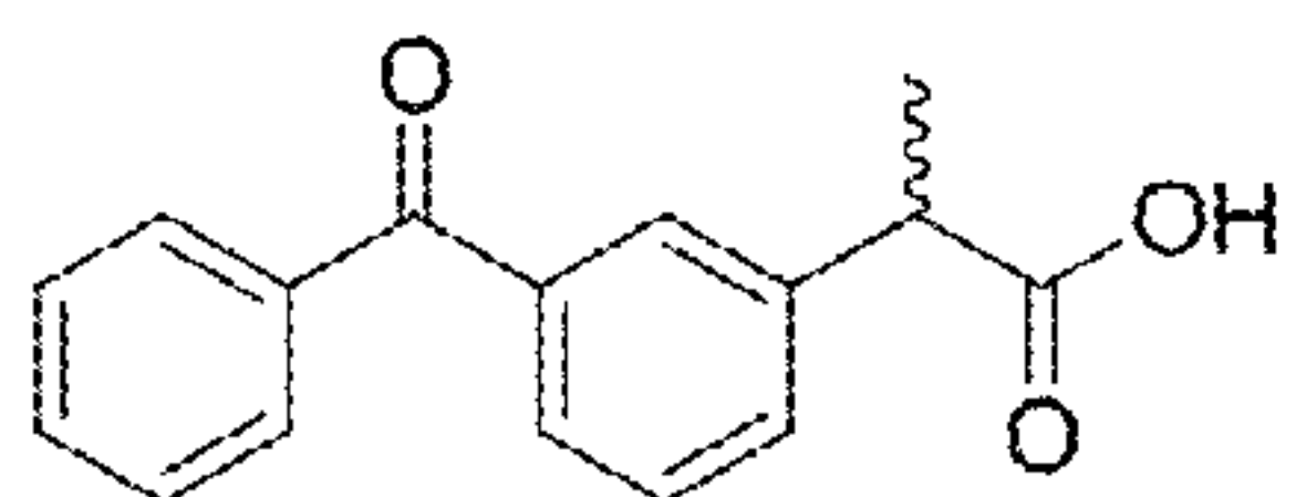
ketoprofen
