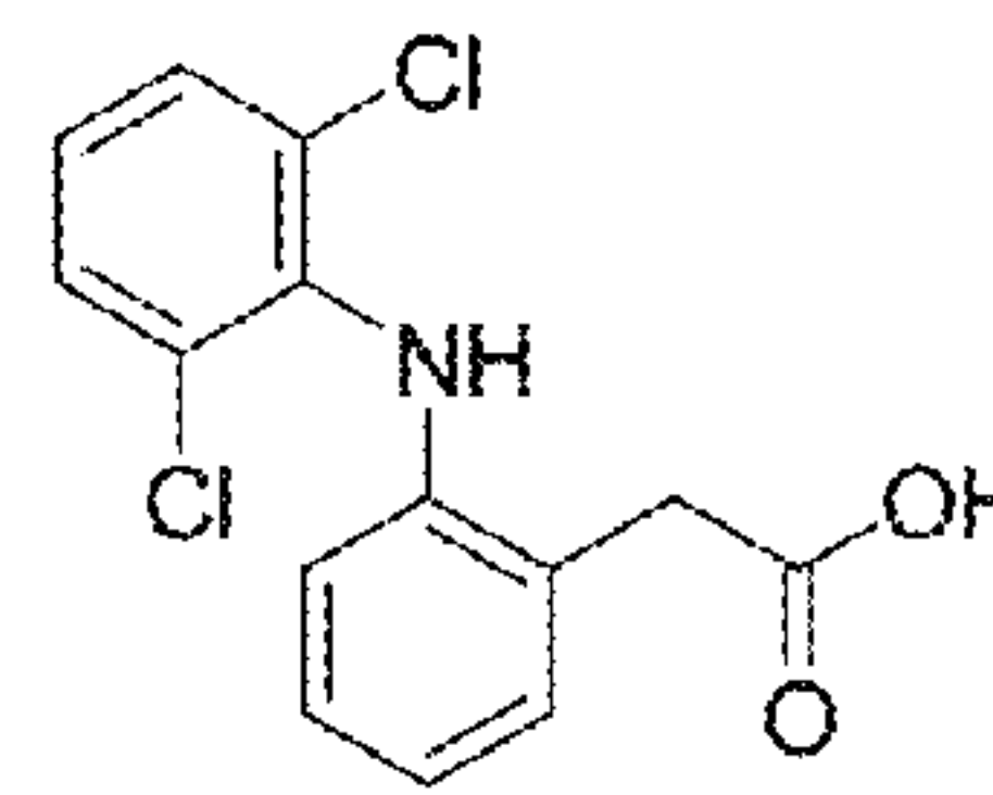
diclofenac
