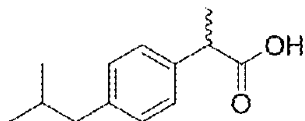
ibuprofen
