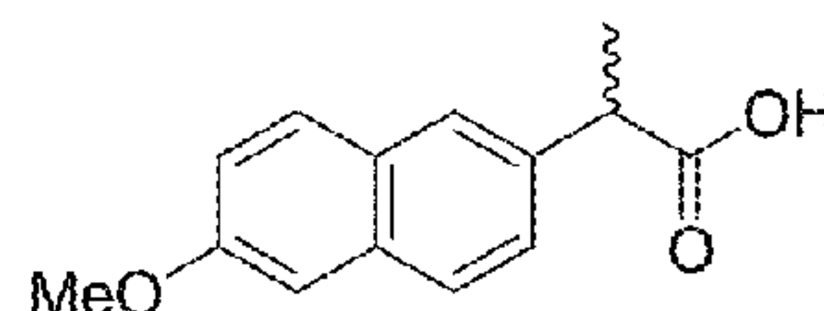
naproxen
