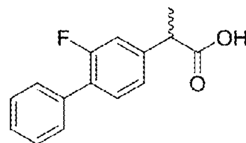
flurbiprofen
