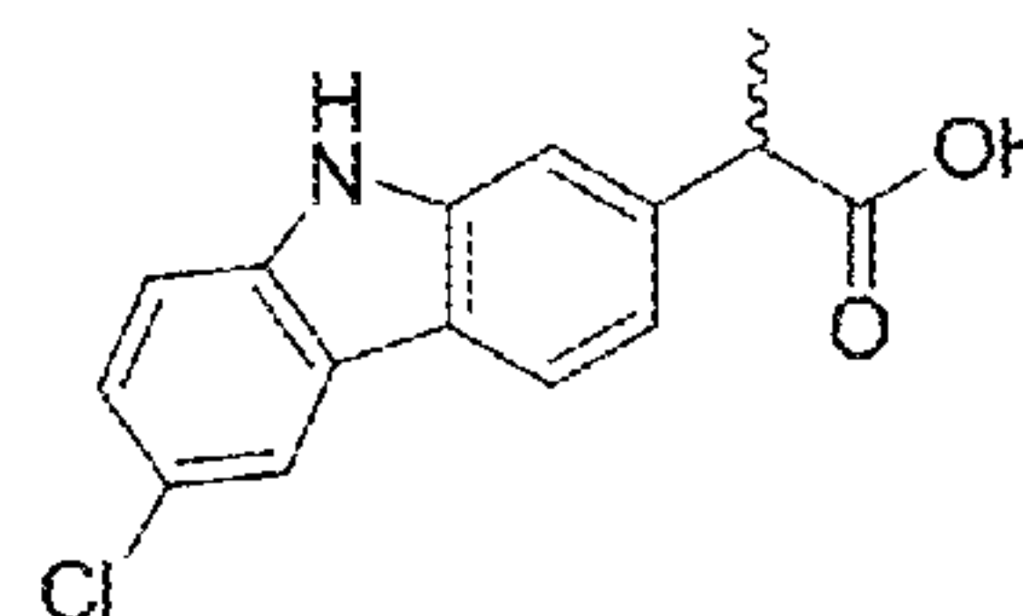
carprofen
