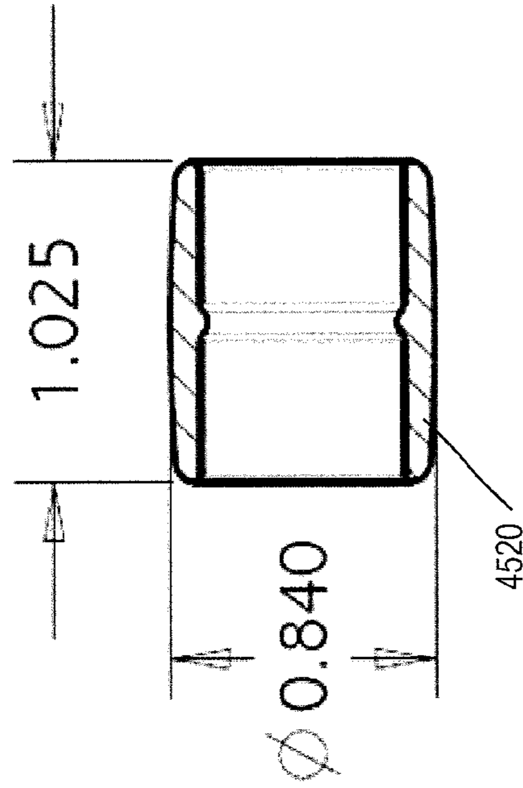
SECTION A-A
