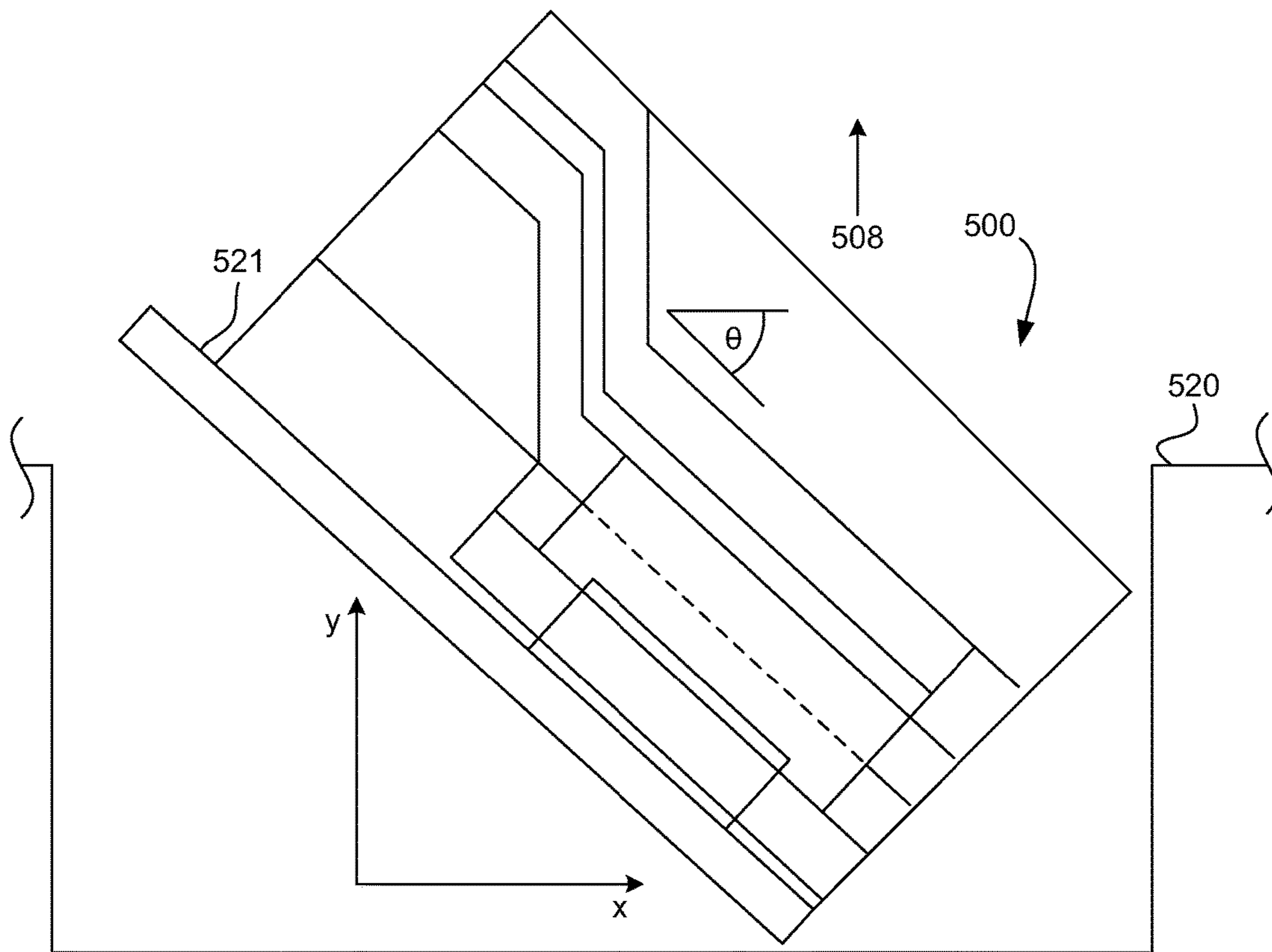
FIG. 5H
