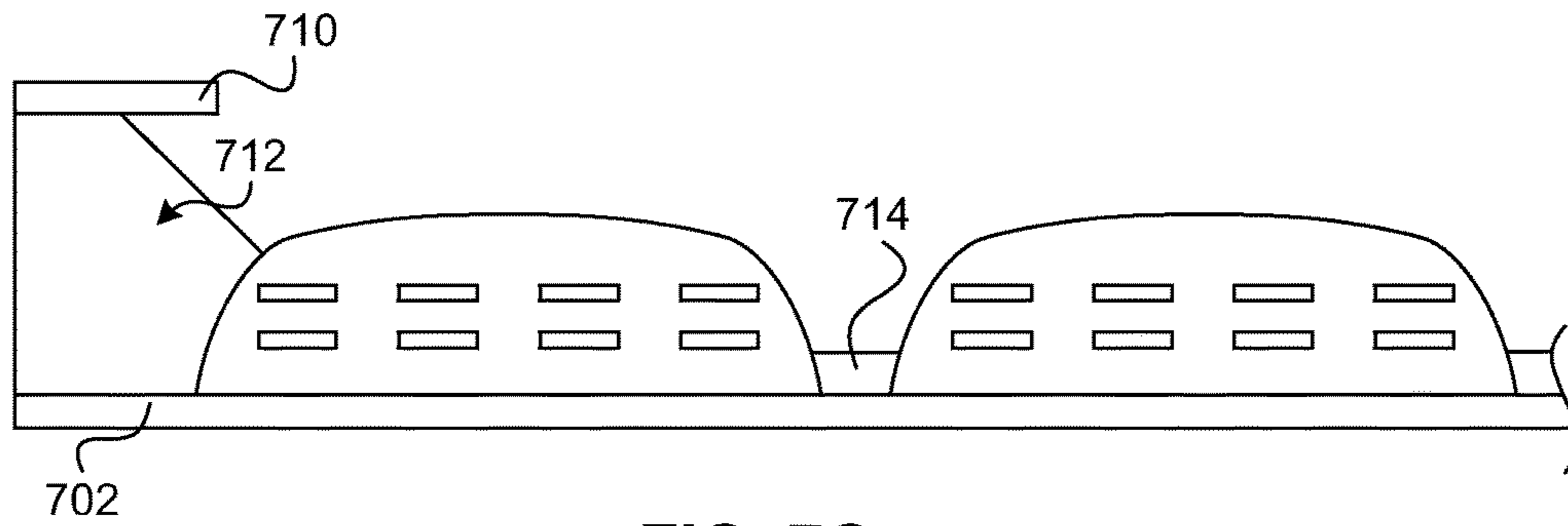
FIG. 7C
