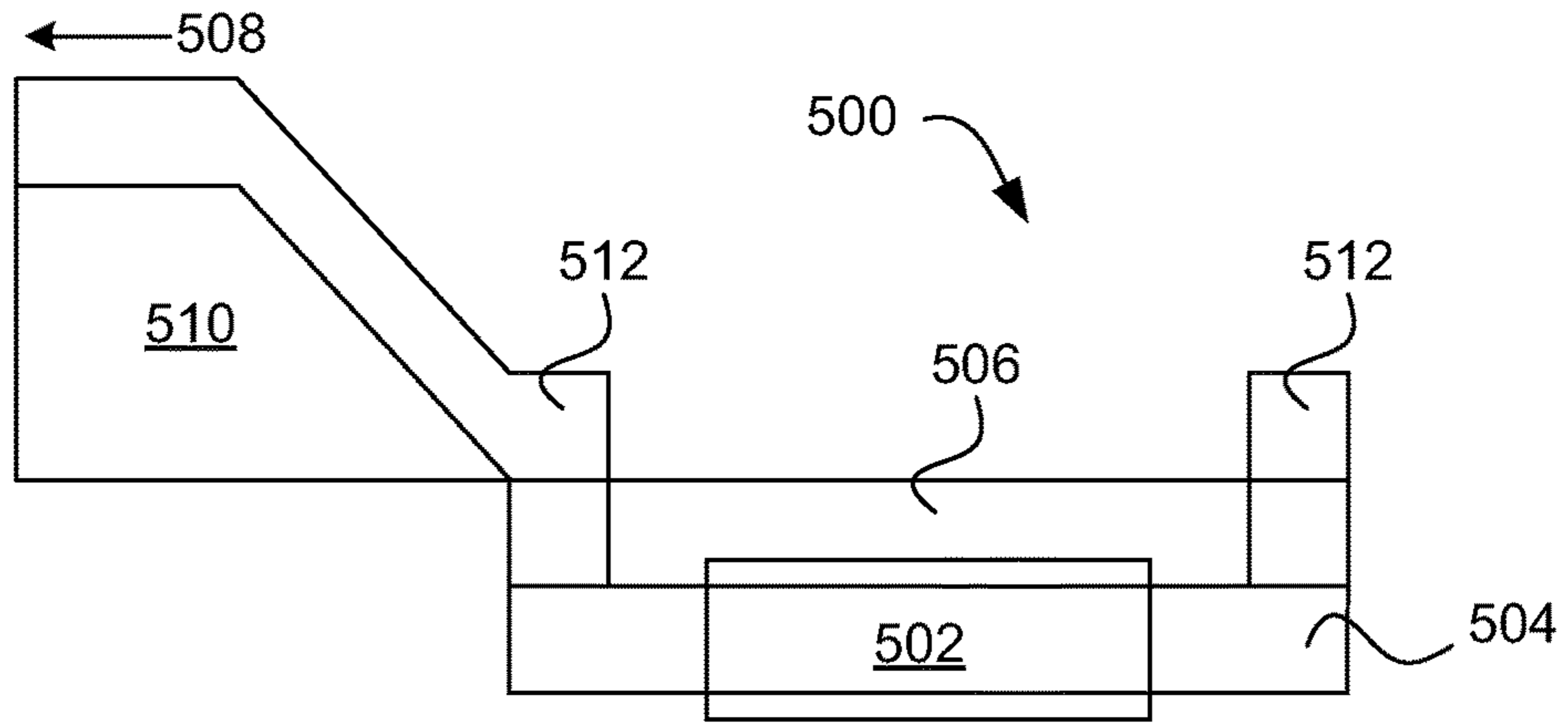
FIG. 5D
