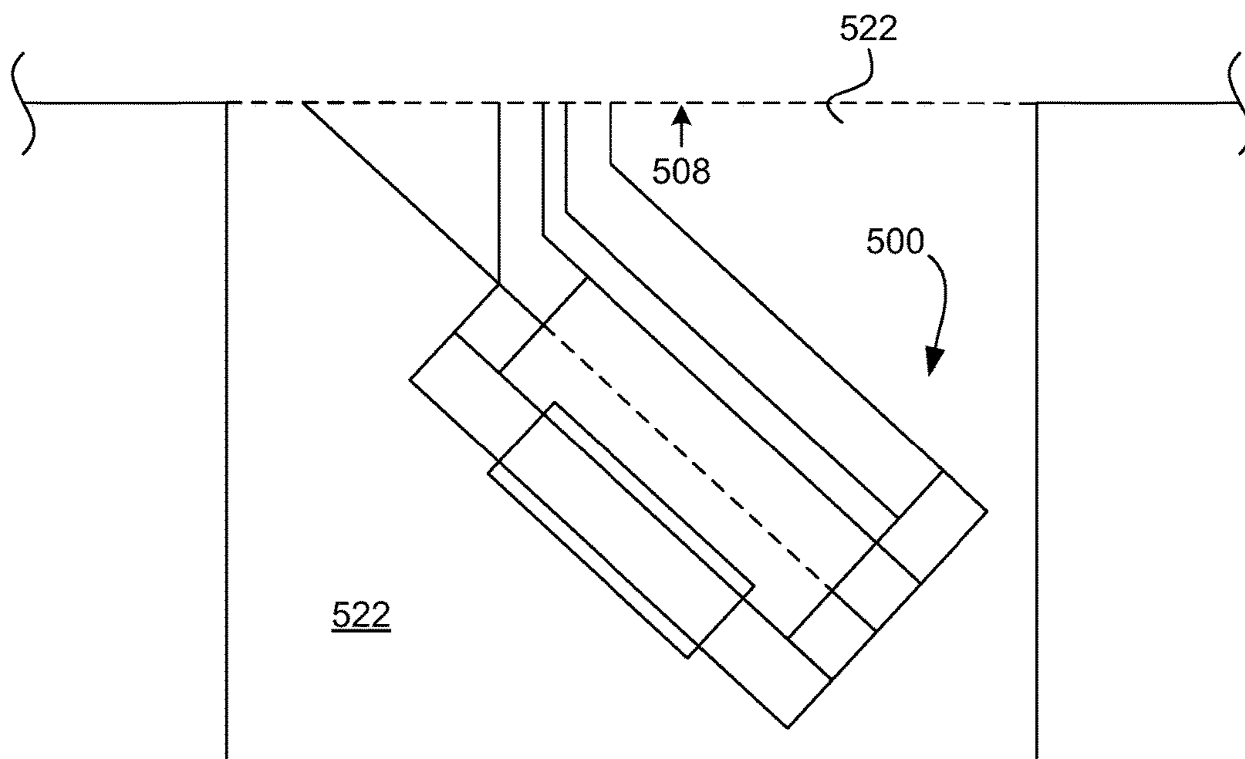
FIG. 5J
