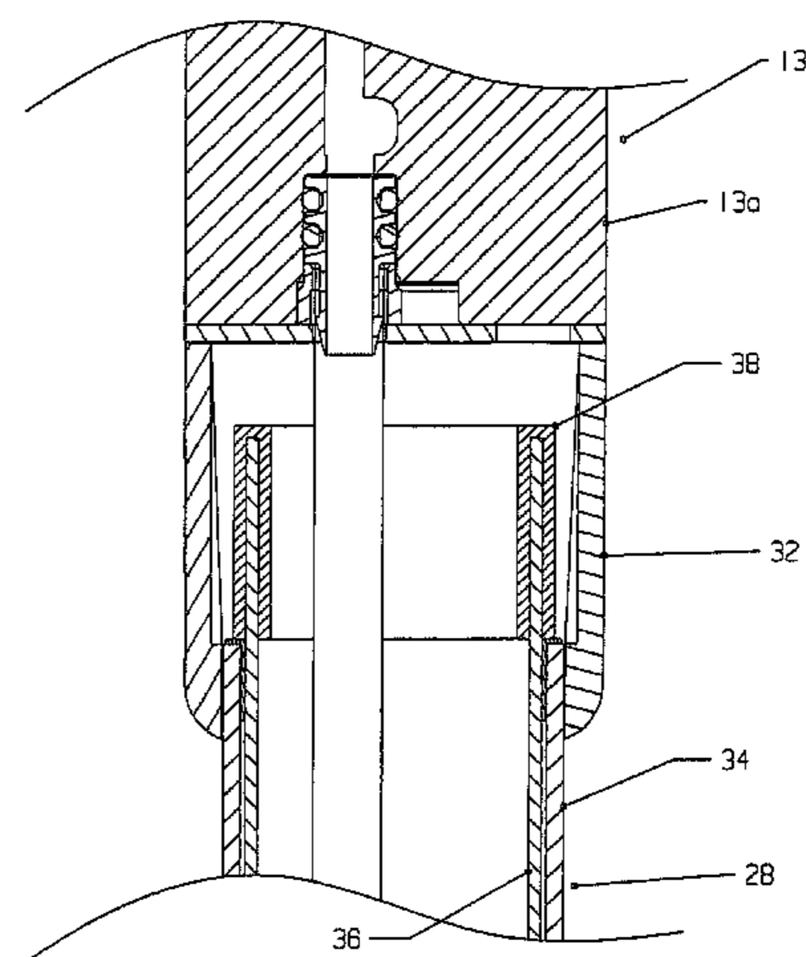
SECTION A-A
