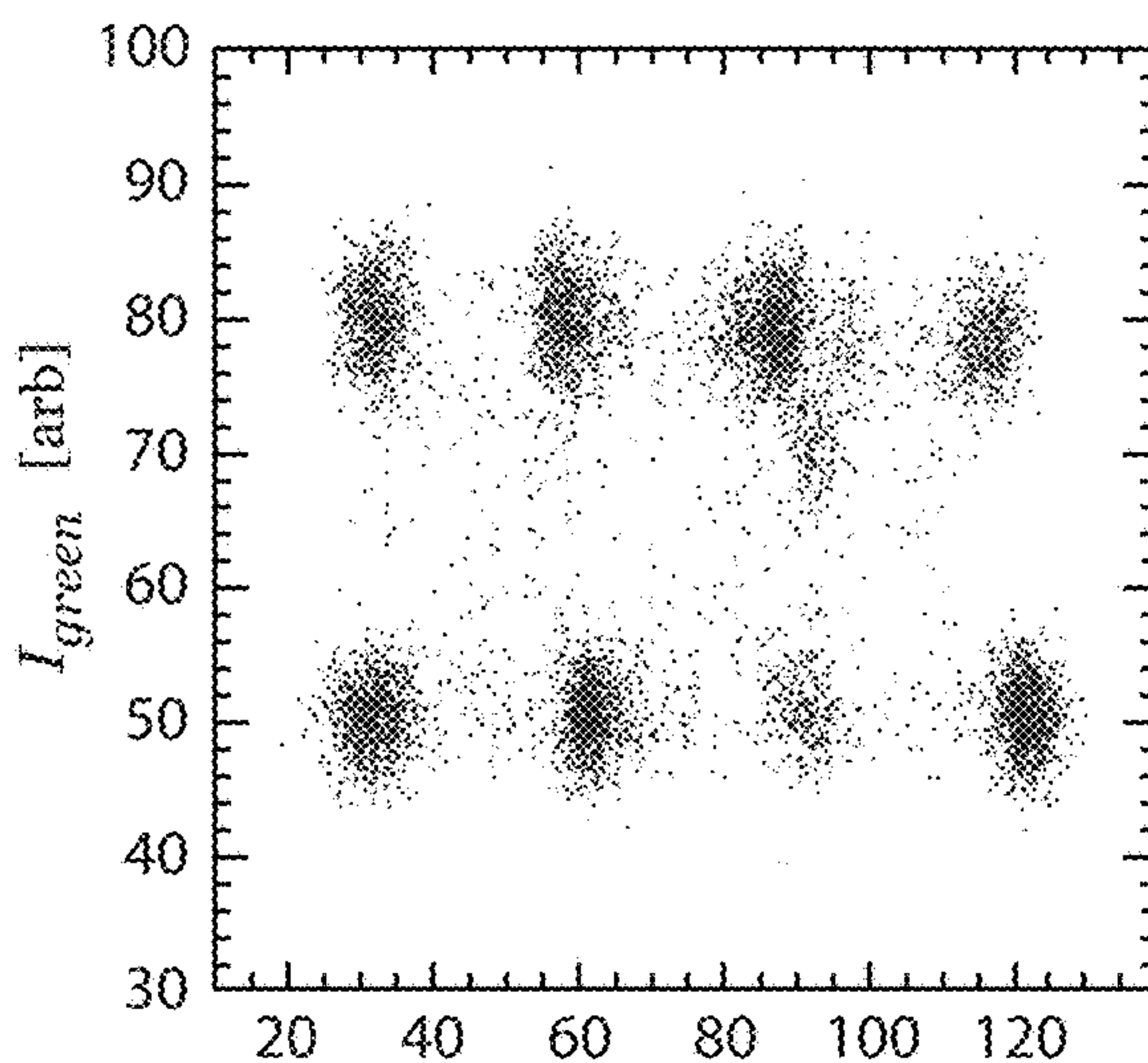
P(I_{red})
